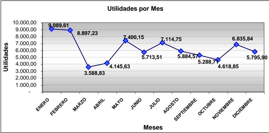
Gráfico 2.6: Utilidades Mensuales
