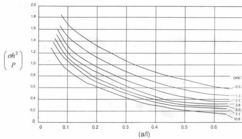
Figura 35.- Estimación de la expresión \left( \frac{\sigma * h^2}{P} \right)
