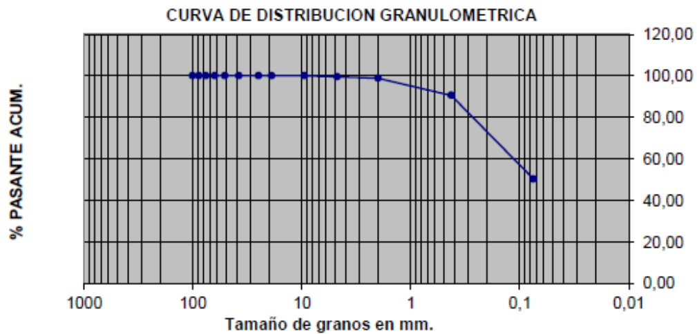
Figura 27.- Curva de Distribución Granulométrica Calicata No.2 (0.50 m.)
