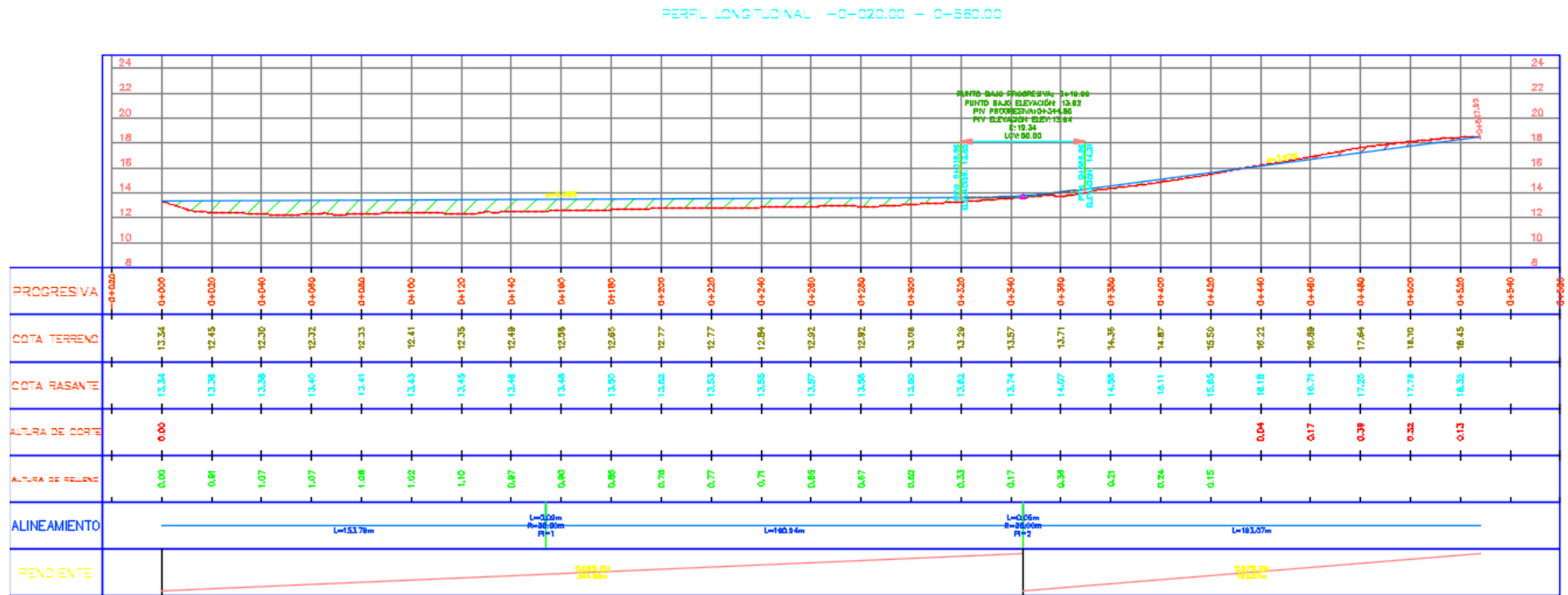
Figura 39 Perfil Longitudinal de la vía de Acceso de la Cabecera Parroquial de Manglaralto
