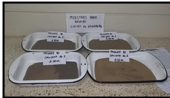
Figura 22.- Tamizado de las muestras para ensayo Límites de Atterberg.
