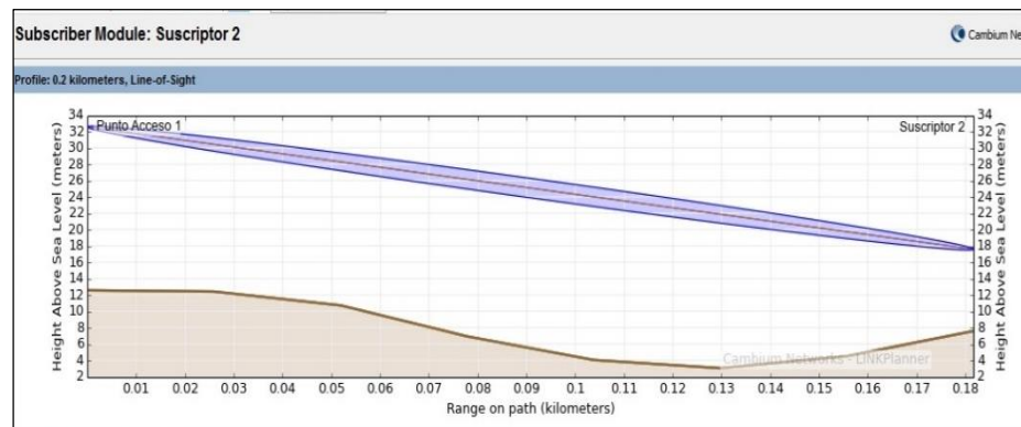
Figura 3.22. Perfil del enlace hacia el suscriptor 2
