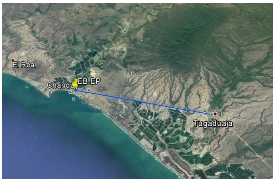
Figura 3.15. Línea de vista entre la Estación Base en Chanduy y la comuna de Tugaduaja
