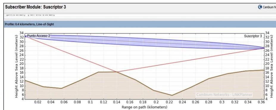
Figura 3.23. Perfil del enlace hacia el suscriptor 3
