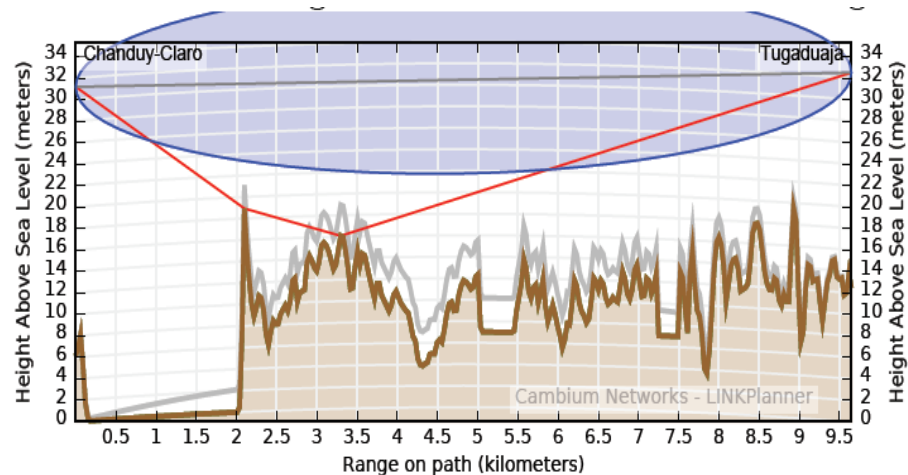
Figura 3.19. Detalles de en enlace Punto-Punto hacia la estación de la empresa privada.
