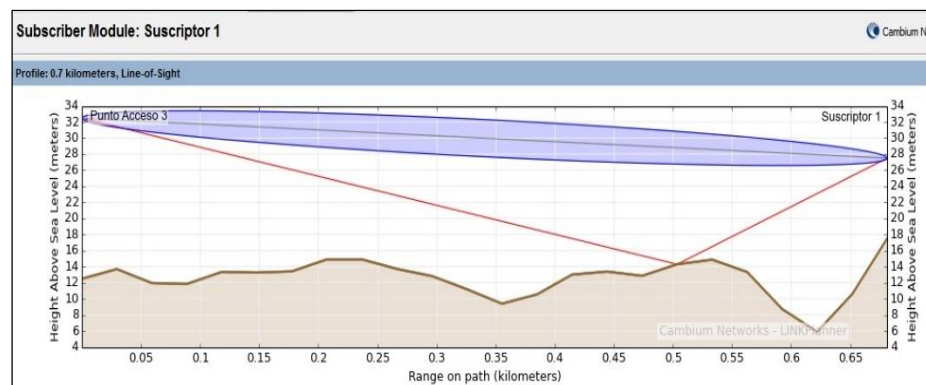
Figura 3.21. Perfil del enlace hacia el suscriptor 1
