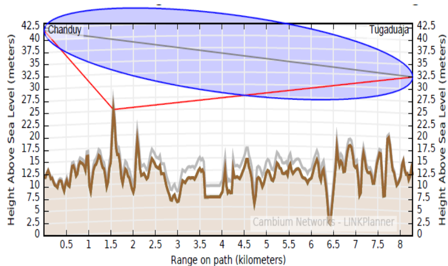
Figura 3.16. Zona de Fresnel Enlace Punto a Punto con la empresa Pública
