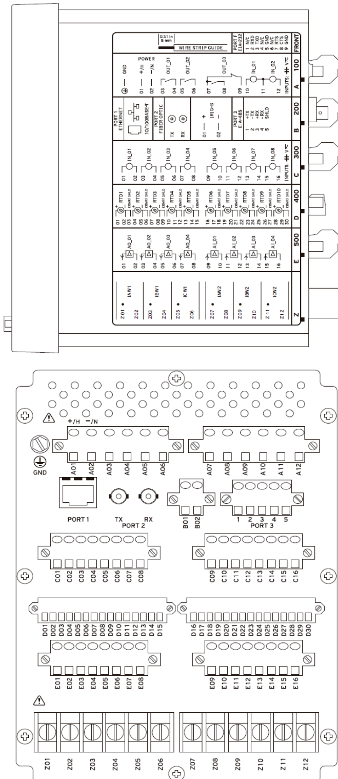
Figura 3. 8: Vista lateral y posterior SEL-787.
