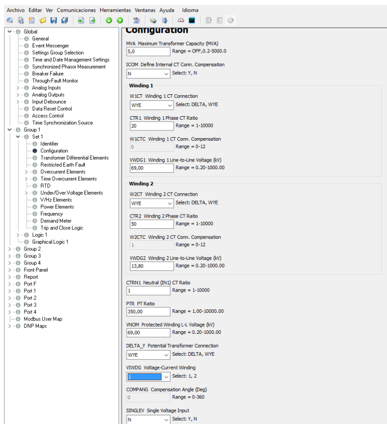
Figura 3. 16: Configuración general de parámetros.
