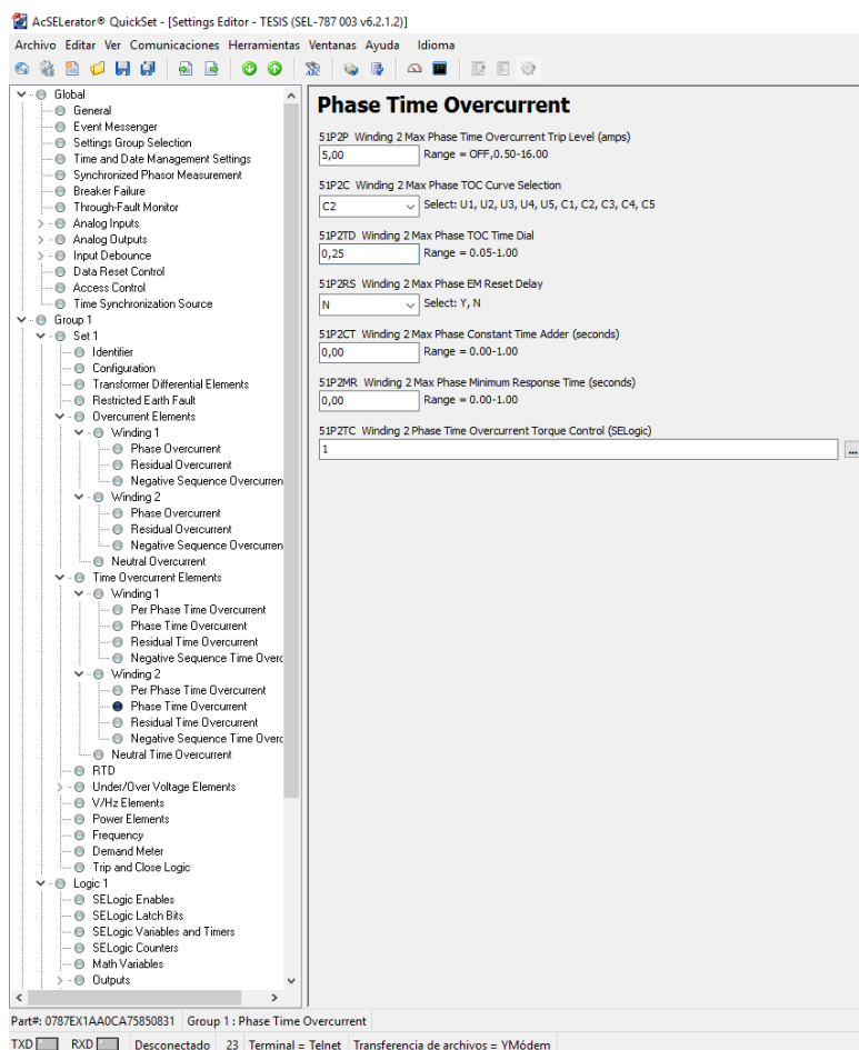
Figura 3. 23: Ajustes de sobrecorriente con retardo de tiempo en baja tensión.
