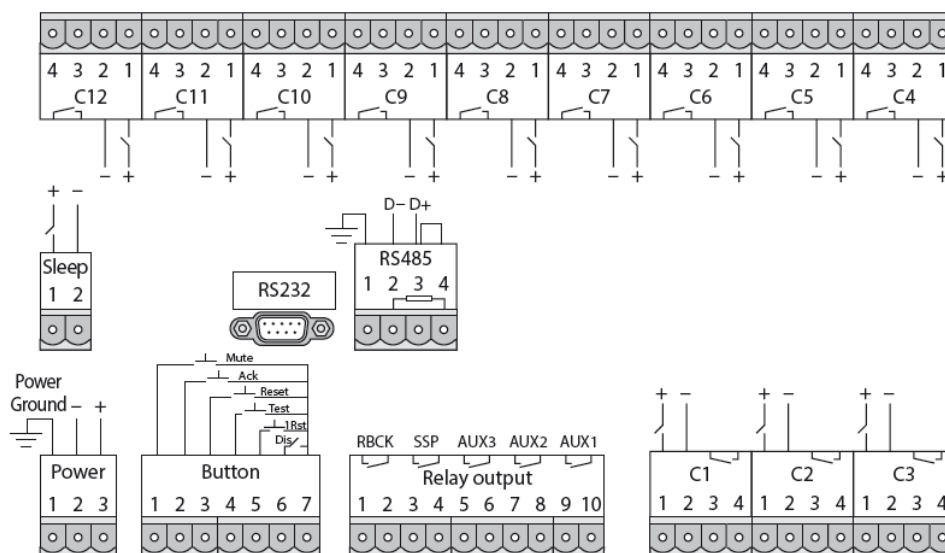
Figura 3. 9 Vista posterior del anunciador de alarmas Mikro
