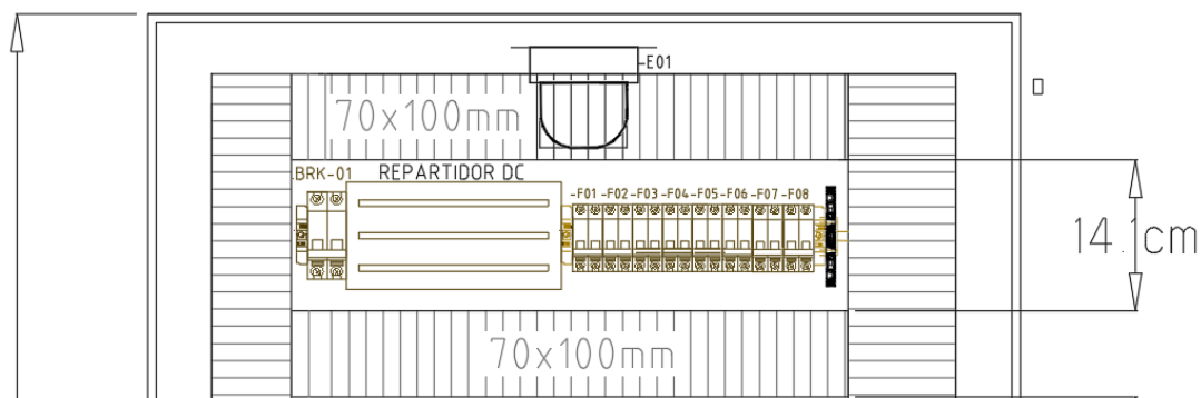
Figura 3. 3: Parte A- interior del tablero.
