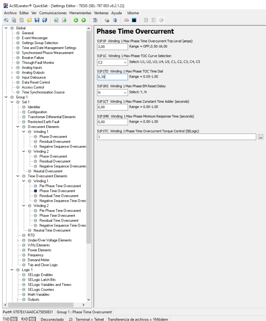
Figura 3. 22: Ajustes de sobrecorriente con retardo de tiempo en alta tensión.
