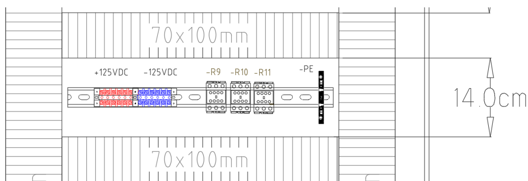
Figura 3. 5: Parte C - interior del tablero.
