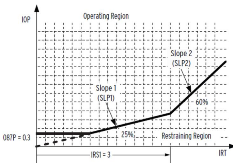
Figura 3. 17: Curva de operación diferencial.
