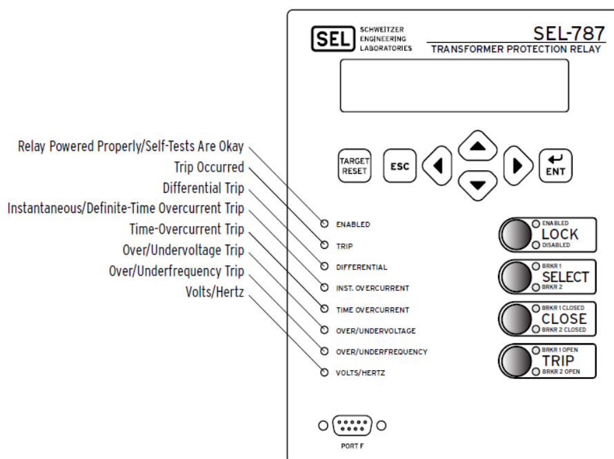
Figura 3. 7: Vista frontal SEL- 787.
