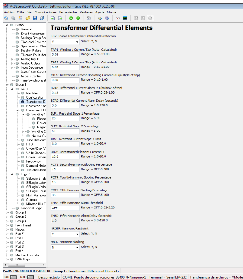
Figura 3. 18 Parámetros de la protección diferencial.
