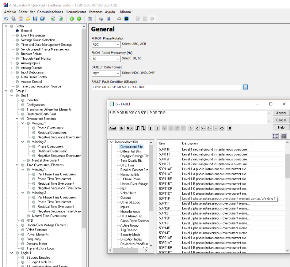
Figura 3. 14: Selección de protecciones.
