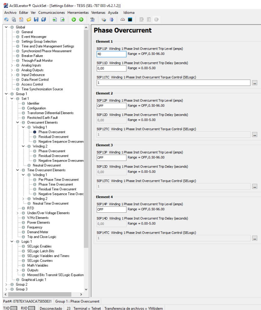
Figura 3. 20: Ajustes sobrecorriente de fase del devanado de alta tensión.
