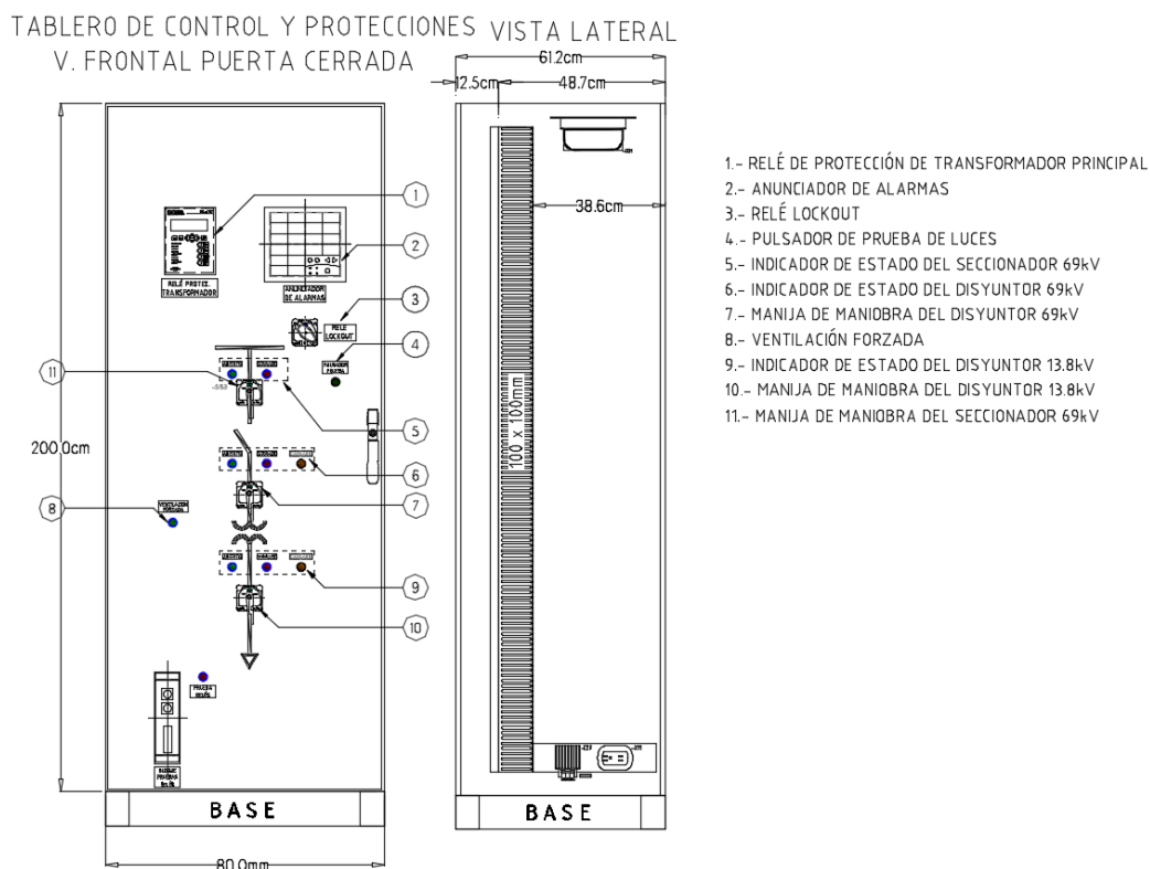
Figura 3. 2: Diseño del tablero de control.
