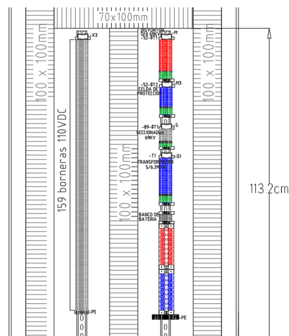
Figura 3. 6: Parte D - interior del tablero.
