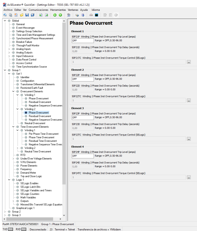
Figura 3. 21: Ajustes de sobrecorriente del devanado de baja tensión.
