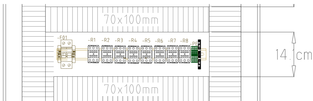
Figura 3. 4: Parte B - interior del tablero.
