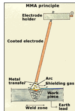
Figura. 2.1 Proceso de Soldadura de Electrodo Cubierto
