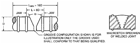
Figura. 3.6 Sección a realizar ensayo de tracción y microscopia para calificación de soldador y proceso de soldadura.
