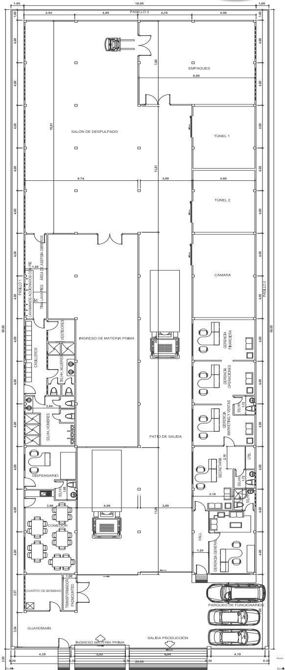
PLANTA GENERAL
