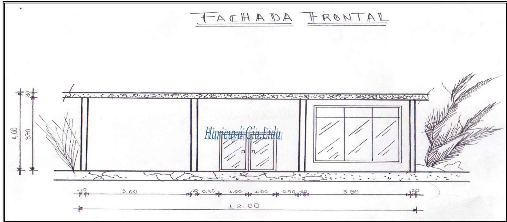
GRAFICO 13: FACHADA FRONTAL DE LA PLANTA
