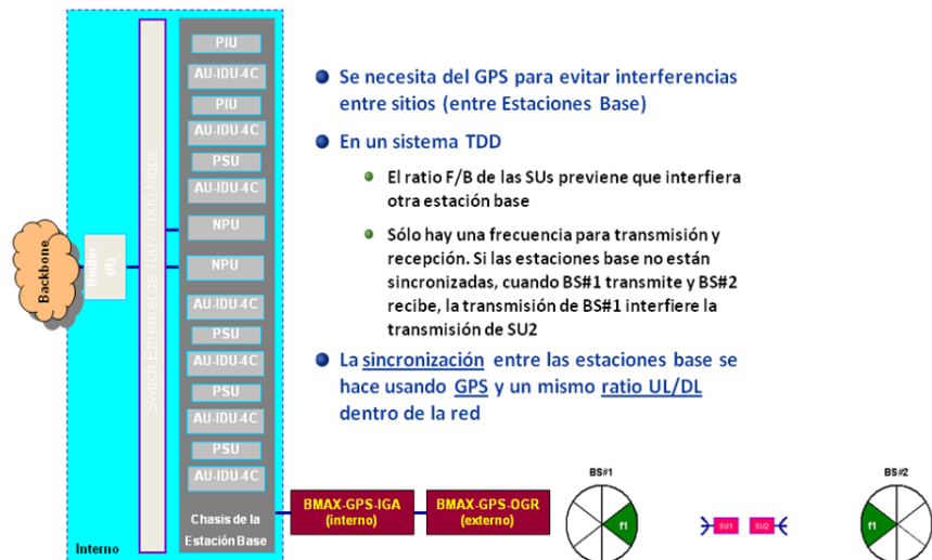
Fig. 4.29.- Sistema de Sincronización mediante GPS.
