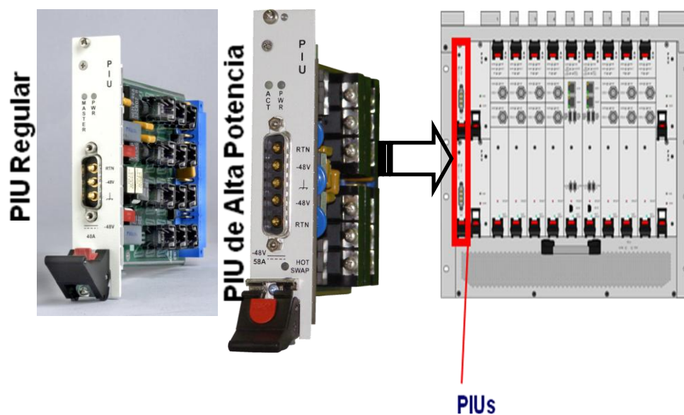
Fig. 4.26.- Unidad de Interface de Energía (PIU)
