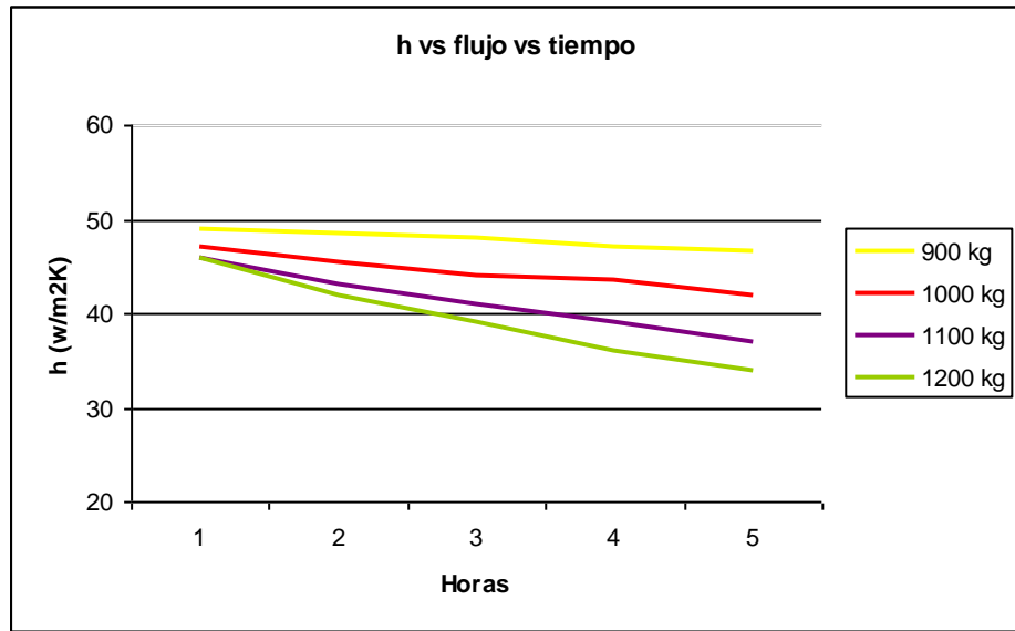
Figura 5.2 Relación de transferencia de calor y flujo a través del tiempo.
