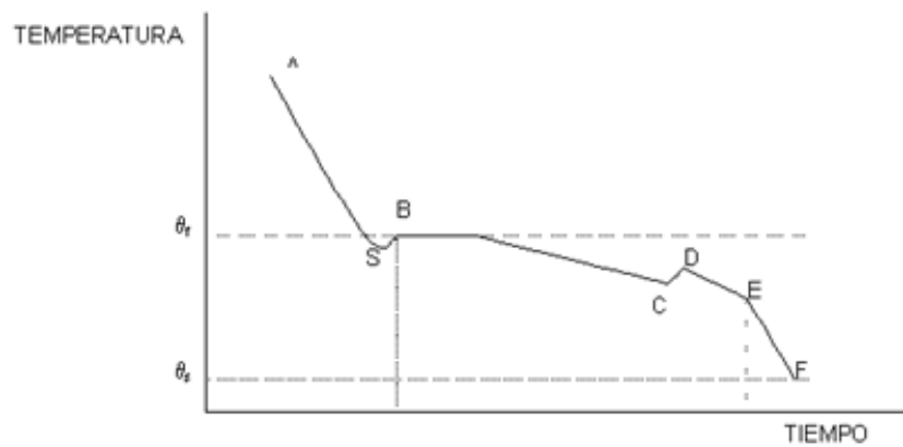
Figura 1.4. Curva de Congelación de una solución típica
