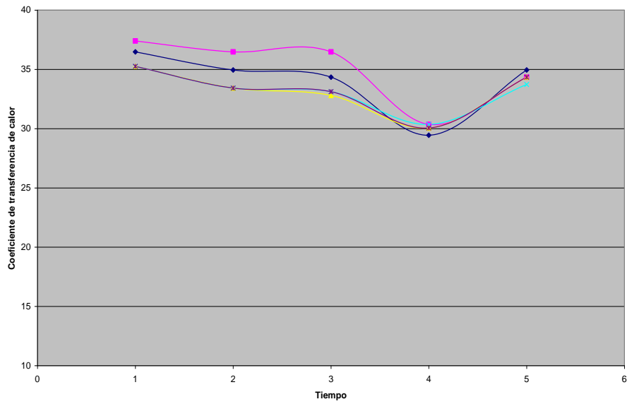
Figura 4.8 Coeficiente de Transferencia de Calor vs Tiempo
