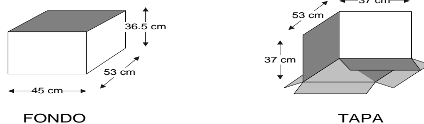
FIGURA 4.5. DIMENSIONES DE FONDOS TAPAS DE CAJAS
