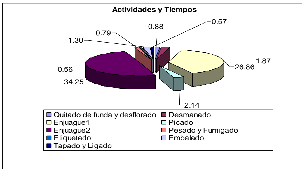
FIGURA 4.10. DIAGRAMA DE PASTEL CON TIEMPOS DE ACTIVIDADES DEL PROCESO
