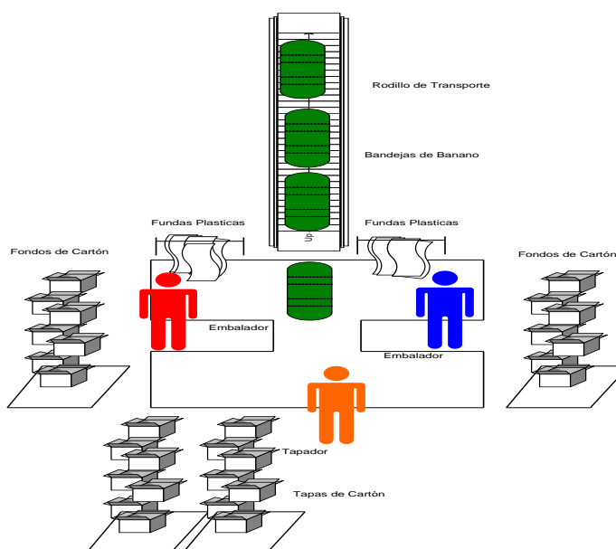
FIGURA 4.9. ESQUEMA PROPUESTO DEL ÁREA DE EMBALADO DE BANANO
