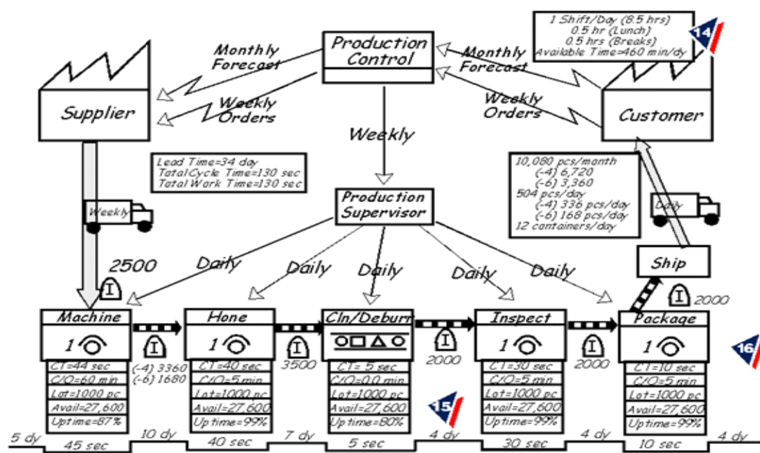
FIGURA 2.7 DIAGRAMA DE DEL PROCESO CON INFORMACION EXTRA.
