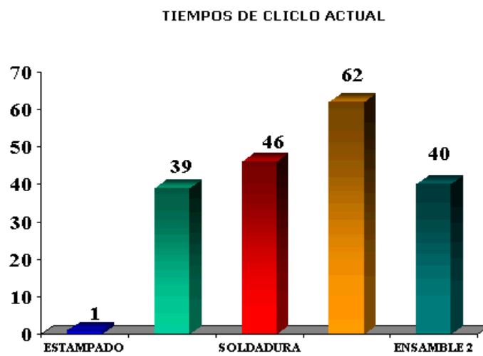
FIGURA 2.14 HISTOGRAMA DE TIEMPOS DE PROCESOS
