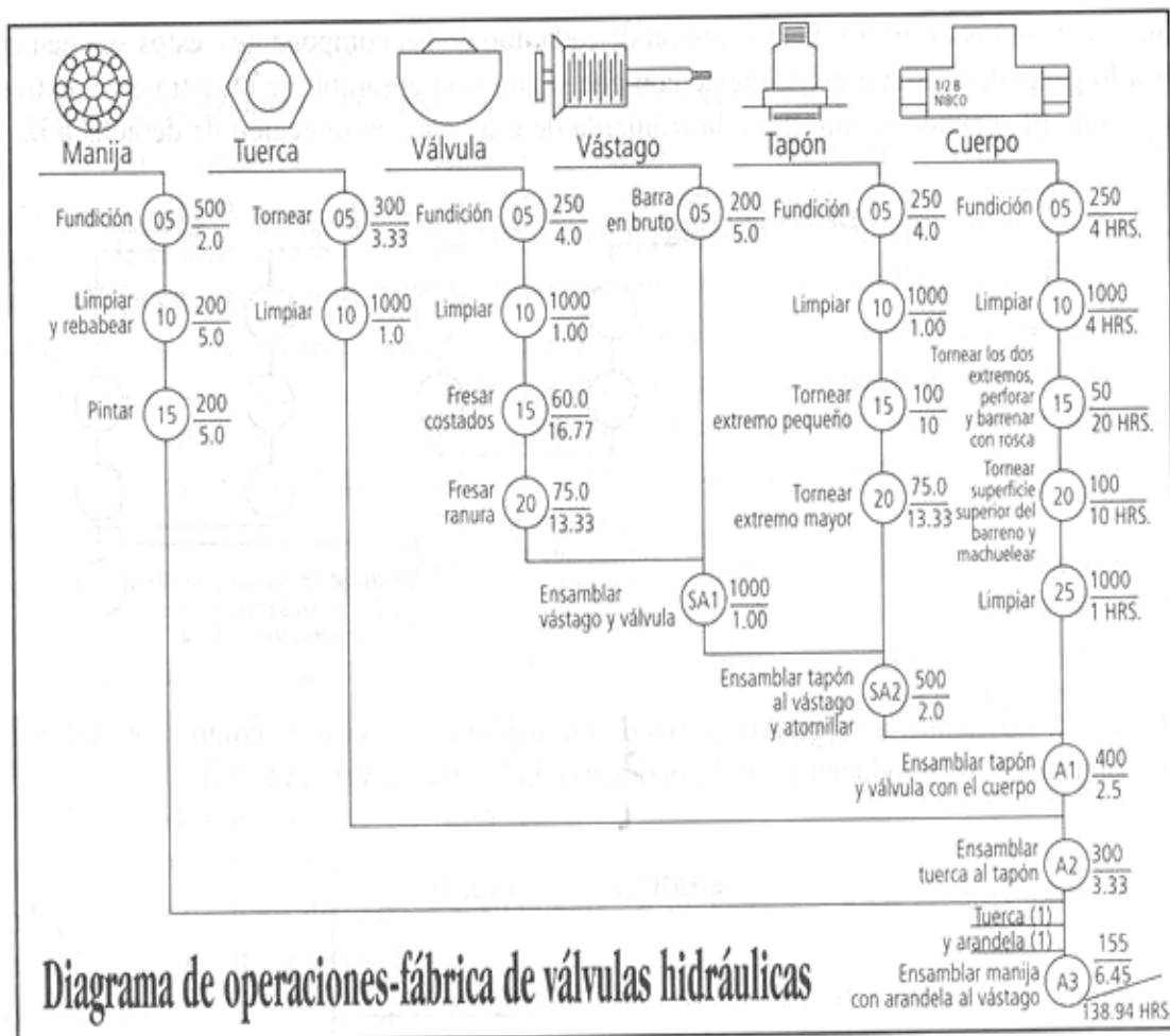
FIGURA 2.1 DIAGRAMA DE OPERACIONES-FABRICA DE VÁLVULAS HIDRÁULICAS.
