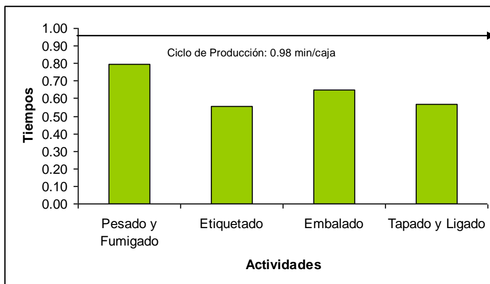
FIGURA 4.13. HISTOGRAMA DE ACTIVIDADES BALANCEADAS
