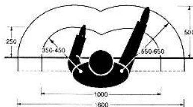
FIGURA 2.13. ARCO HORIZONTAL DE ALCANCE DEL BRAZO Y ÁREA DE TRABAJO SOBRE UNA MESA (COTAS EN MM)
