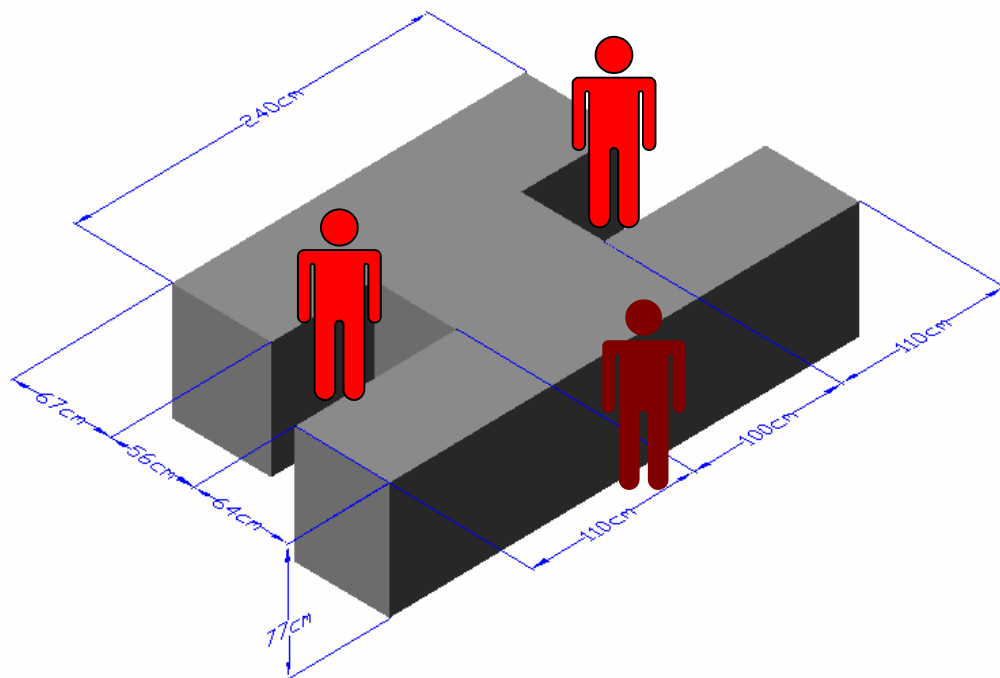
FIGURA 4.6. MESA DE TRABAJO PARA EL EMBALADO DEL BANANO
