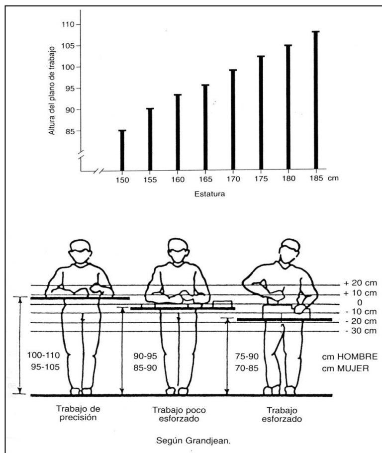
FIGURA 2.11 PLANOS DE TRABAJO EN POSICION DE PIE Fuente: Farrer, Minaya, Niño, Ruiz. Manual de Ergonomía, 1995.
