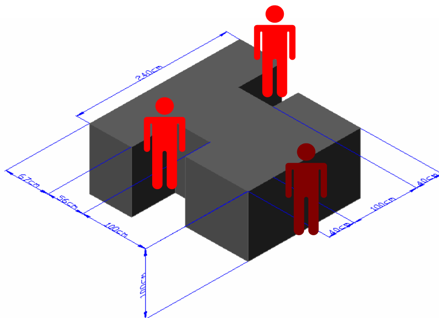
FIGURA 4.7. MESA DE TRABAJO PROPUESTA PARA EL EMBALADO DEL BANANO
