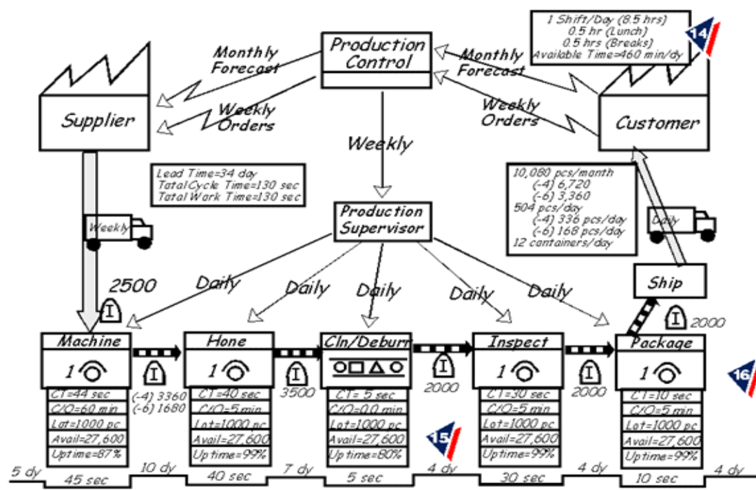
FIGURA 2.8 DIAGRAMA DE CADENA DE VALOR DEL PROCESO ACTUAL
