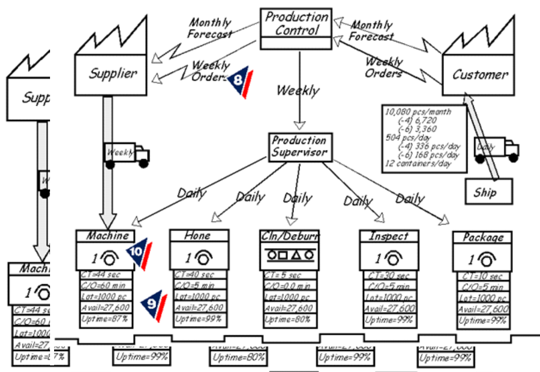
FIGURA 2.6 DIAGRAMA DE DESPLAZAMIENTO DE ACUERDO AL PROCESO CON SUS DATOS.
