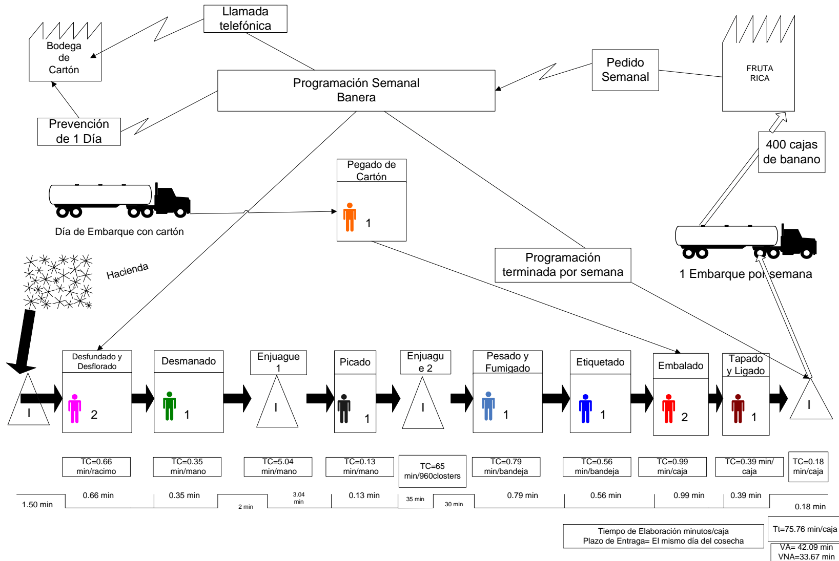
FIGURA 5.1. VSM PROPUESTO DEL PROCESO DE EMBALADO DE BANANO Y SUBPROCESO DE ELABORACIÓN DE CAJAS
