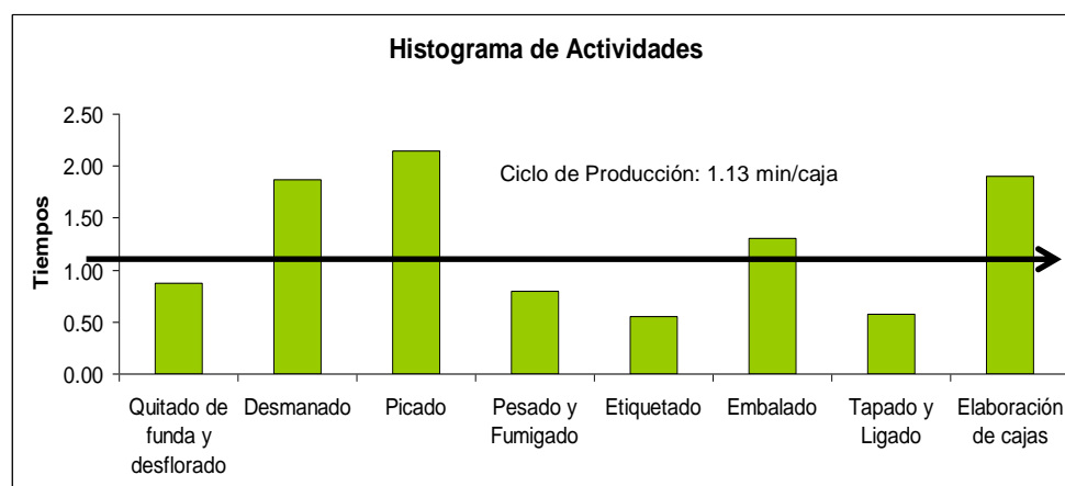
FIGURA 4.11. HISTOGRAMA DE ACTIVIDADES DEL PROCESO
