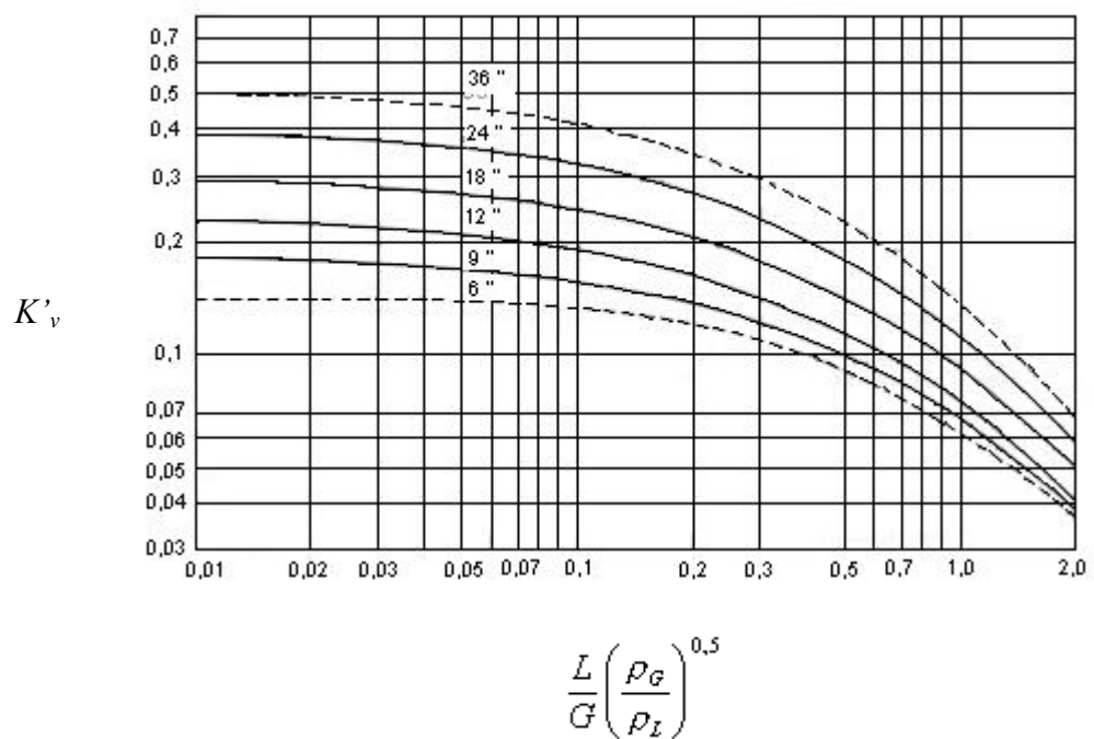
FIGURA 4.1 VALORES DE K_v EN FUNCION DEL ESPACIADO
