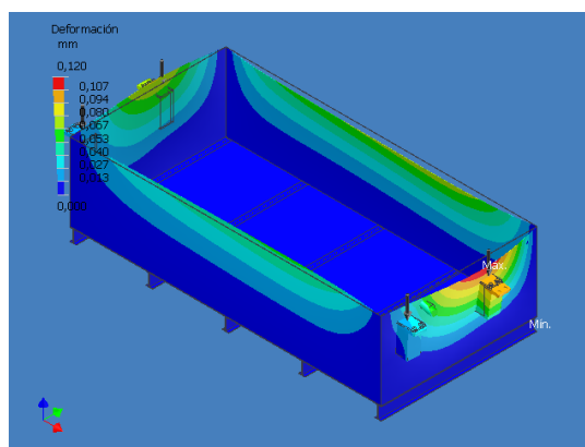
FIGURA 4.13. DEFORMACION
