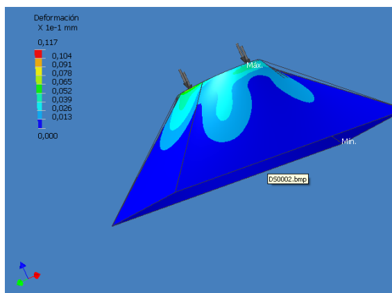
FIGURA 4.18. DEFORMACION
