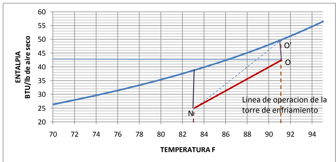
FIGURA 3.20. DIAGRAMA DE OPERACIÓN DE ENFRIAMIENTO DEL AGUA
