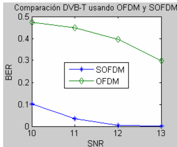
Figura 12: BER vs SNR del estándar DVB-T usando ambas modulaciones
