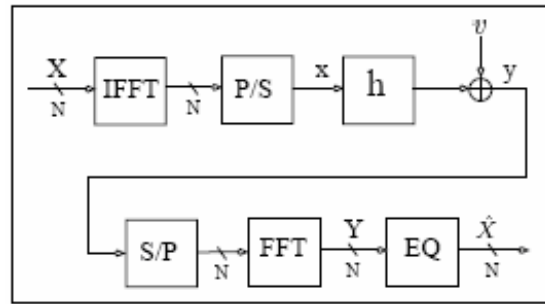
Figura 1. Sistema OFDM Convencional
