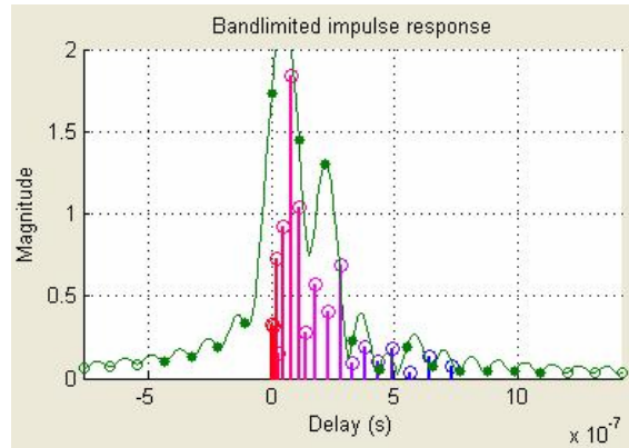
Figura 11. Respuesta impulsional de canal multiruta
