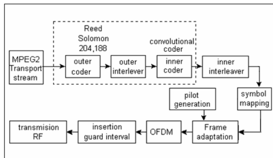
Figura 3. Diagrama de bloques de sistema DVB-T
