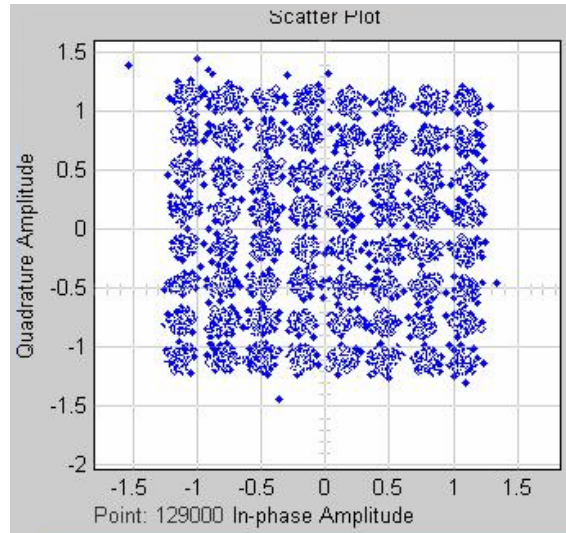
Figura 10. Constelación QAM 64 resultante después de la ecualización y la decodificación de la matriz de hadamard
