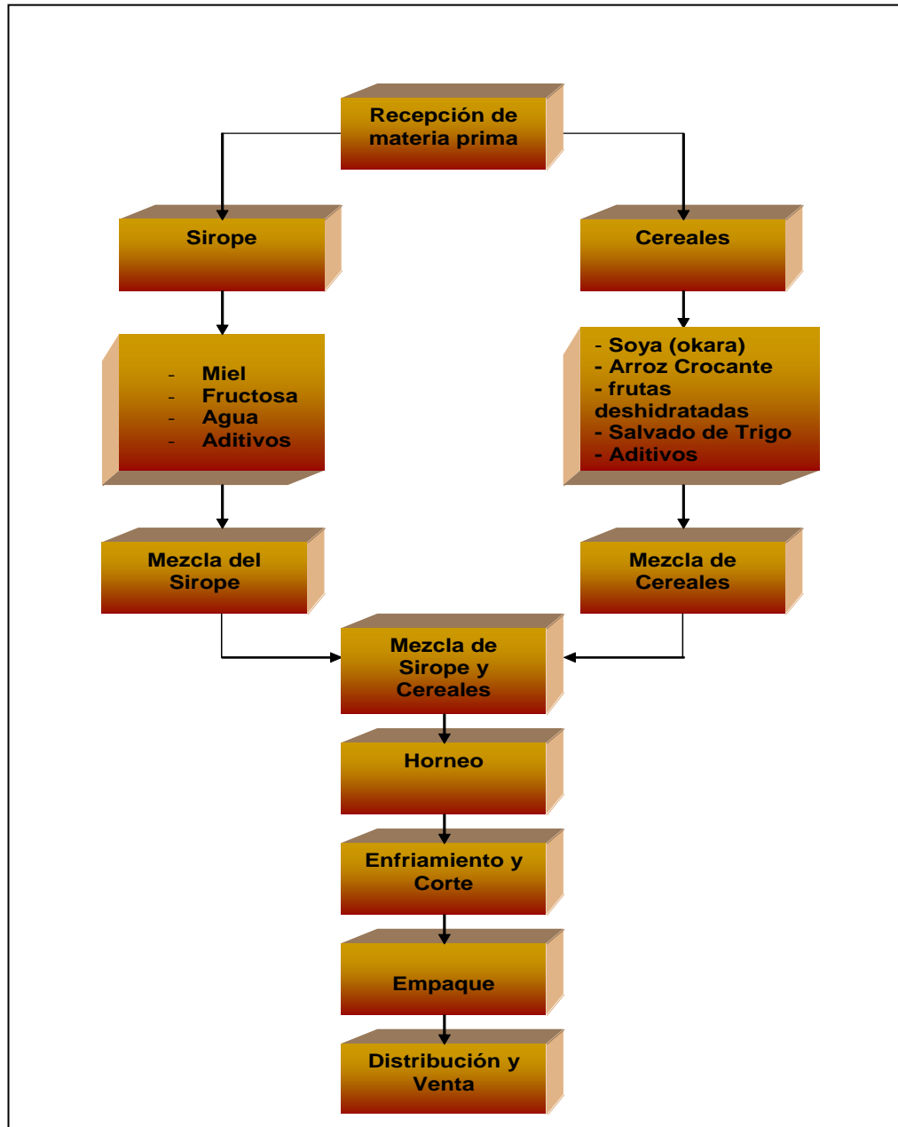
Figura 3.16 Diagrama de Flujo Barras Energéticas
