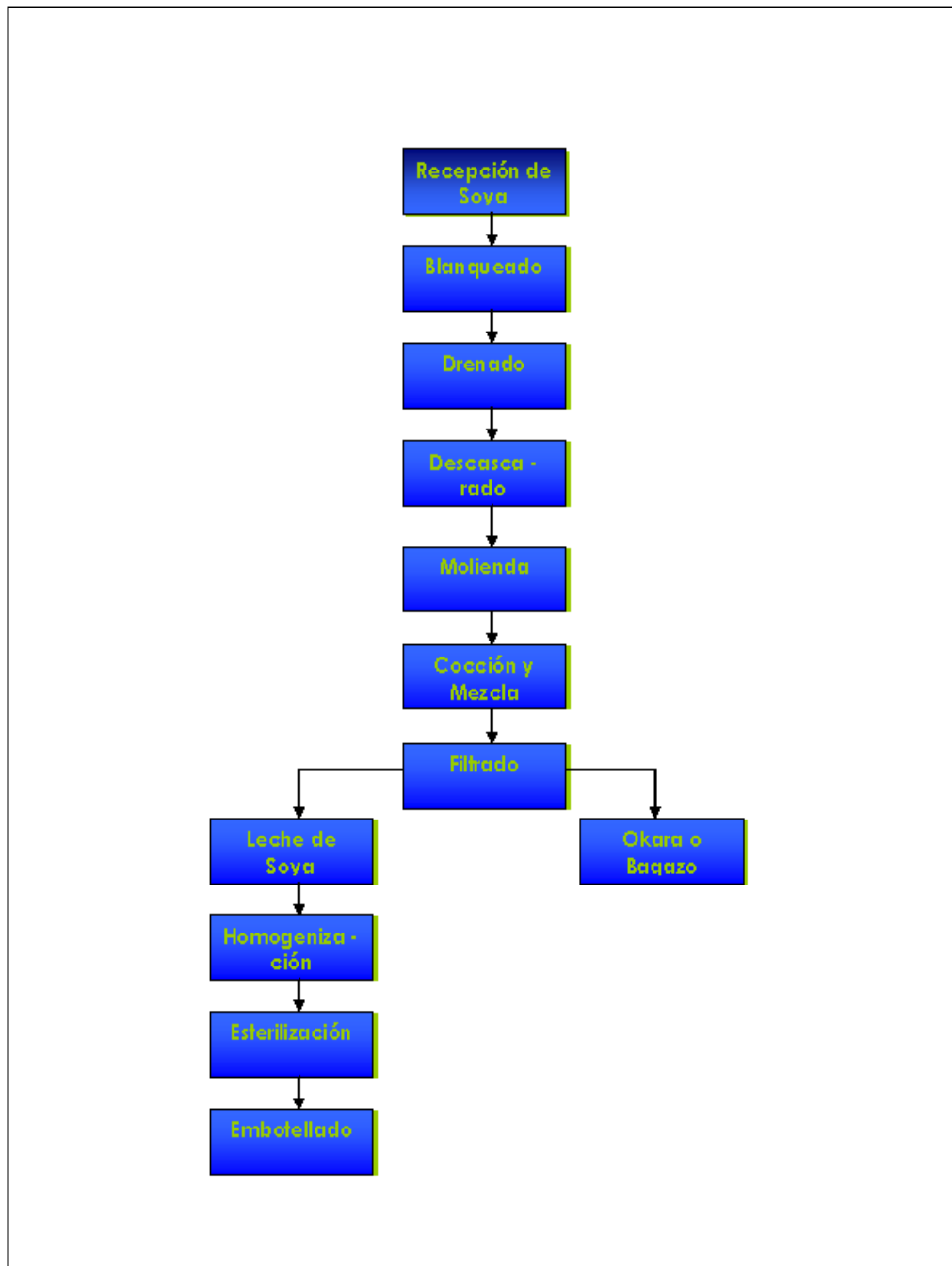
Figura 1.4 Diagrama de Flujo Método Illinois
