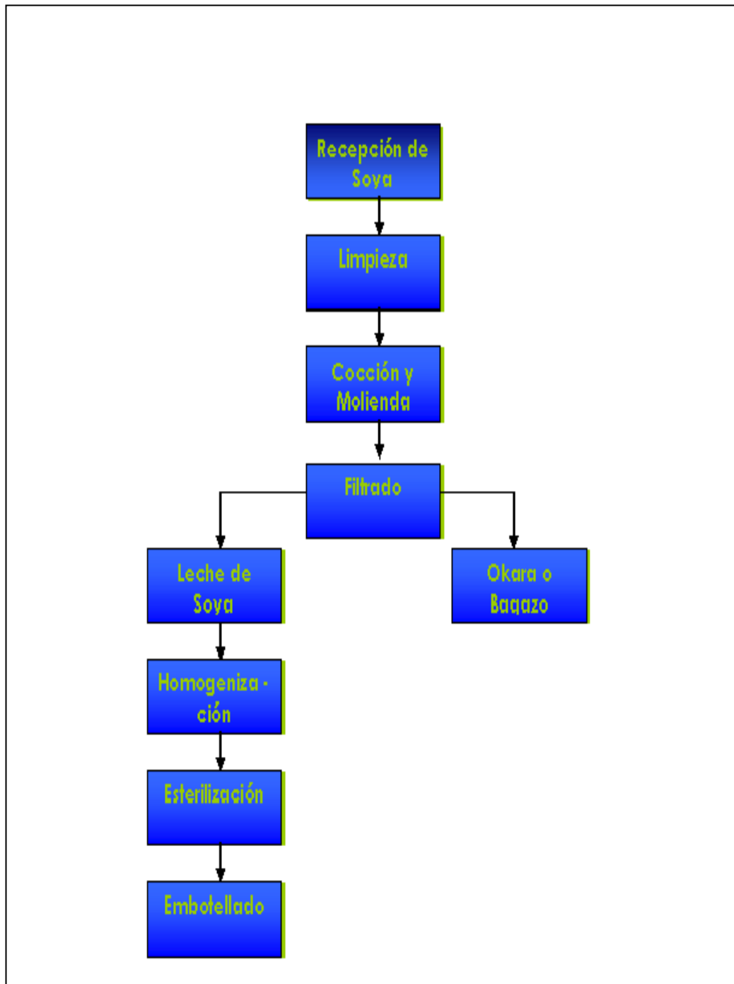
Figura 1.5 Diagrama de Flujo Método de Cornell
