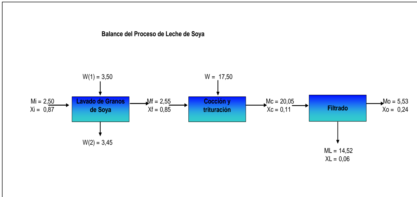
Figura 3.15 Balance del Proceso Leche de Soya
