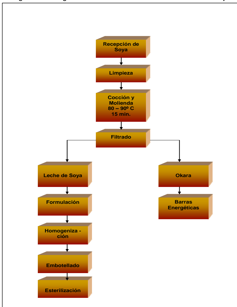
Figura 3.1 Diagrama de Proceso de Leche Saborizada de Soya
