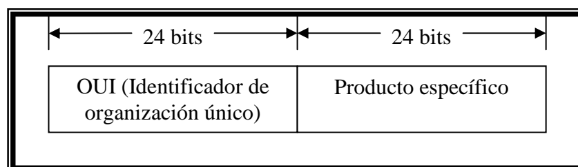
Figura 2.2 Dirección MAC
