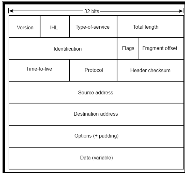
Figura 2.18 Formato estructura IP
