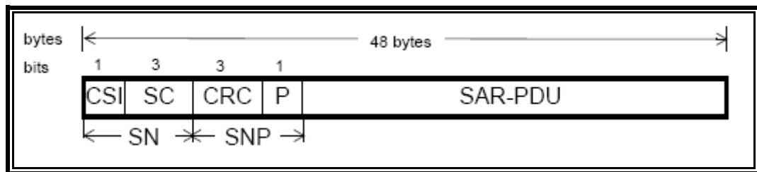
Figura 2.16 PDU SAR-AAL1 14
