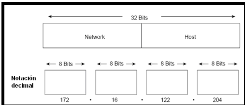
Figura 2.19 Dirección IP
