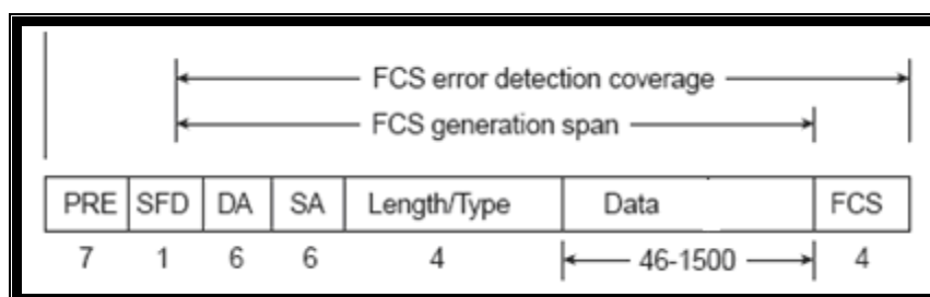
Figura 2.3 Formato MAC data frame
