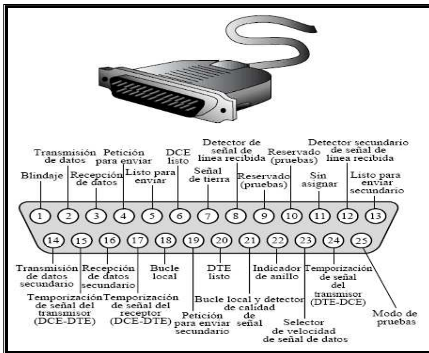
Figura 1.6 Funciones de los pines en la versión DB-25 6
