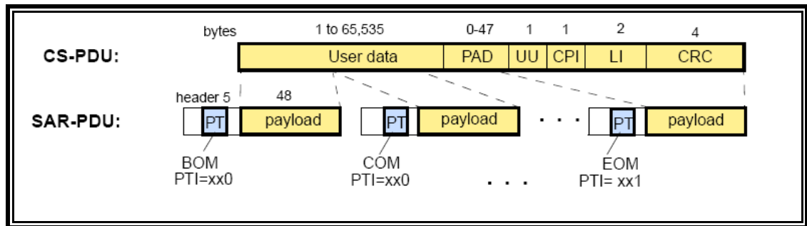
Figura 2.17 Ensamblado de PDU AAL5 15
