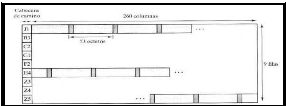
Figura 2.13 Carga útil STM-1 para transmisión de celdas ATM basada en SDH
