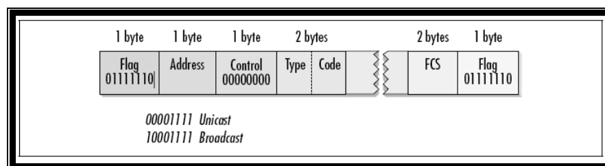
Figura 2.4 Trama cHDLC 8
