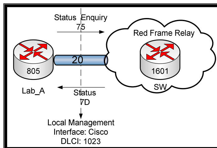
Figura 4.5.15 Intercambio de mensajes LMI
