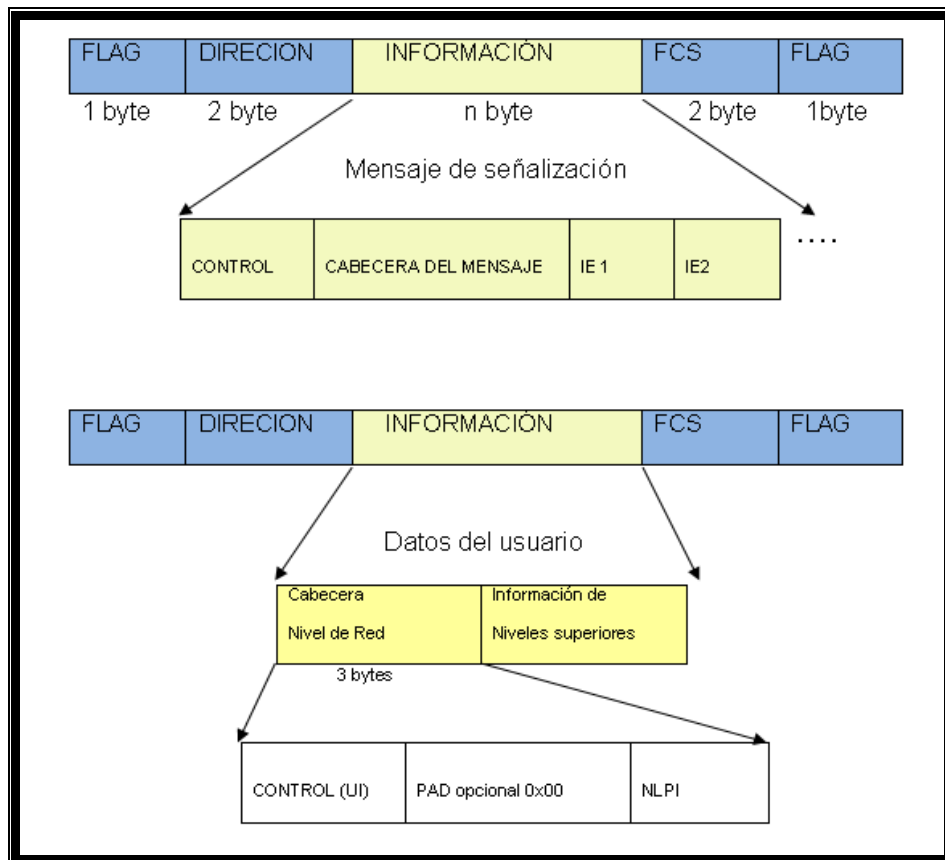
Figura 2.7 Campo de información
