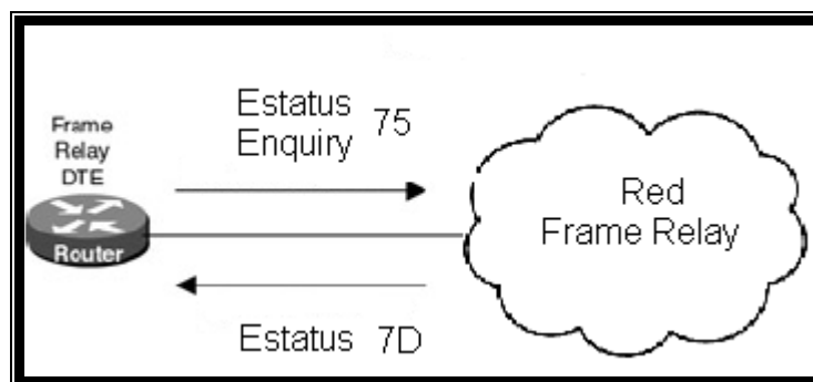
Figura 2.9 Intercambio de mensajes del estado del enlace.
