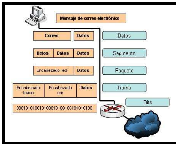
Figura 1.2 Proceso detallado de encapsulamiento 2
