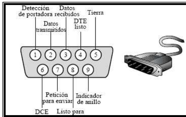
Figura 1.7 Funciones de los pines en la versión DB-9 7
