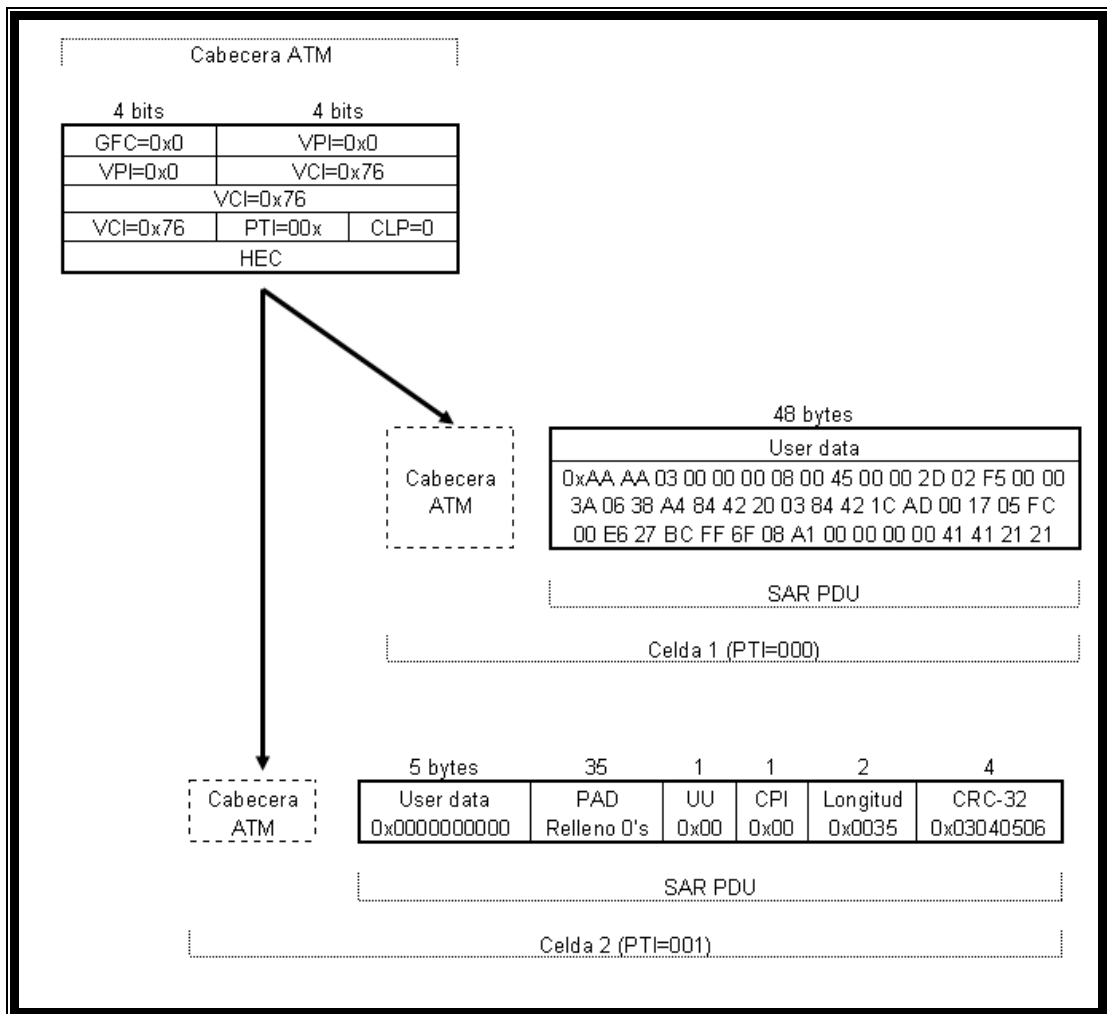
Figura 4.6.6 Reensamble de celdas en SAR-PDU
