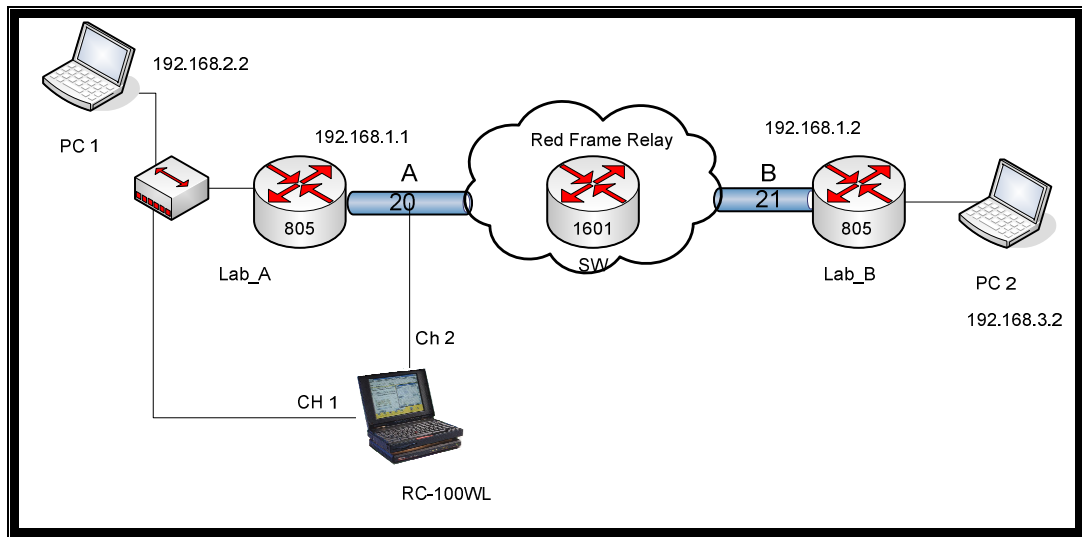
Figura 4.5.1 Diagrama de red
