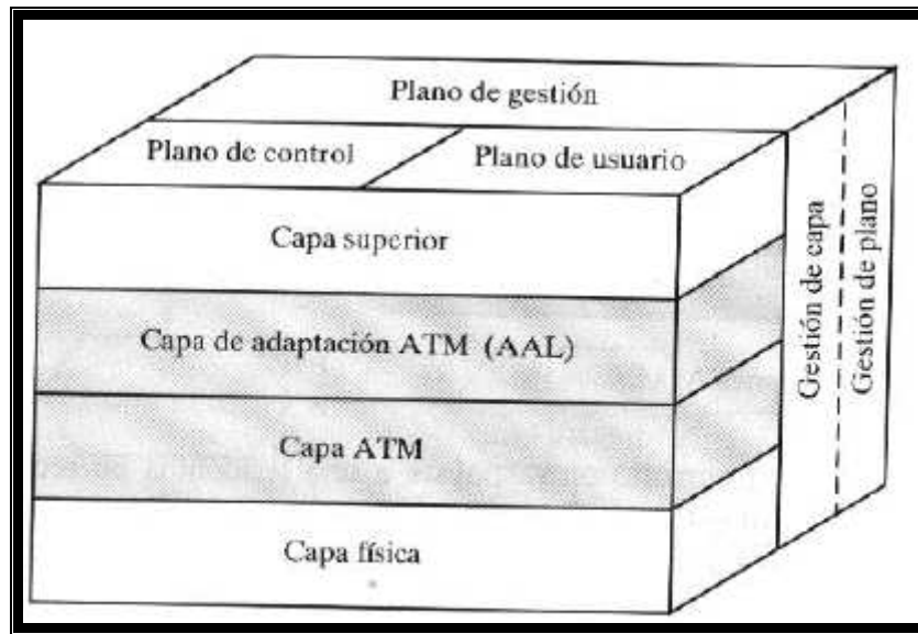
Figura 2.10 Modelo de referencia del Protocolo ATM 11
