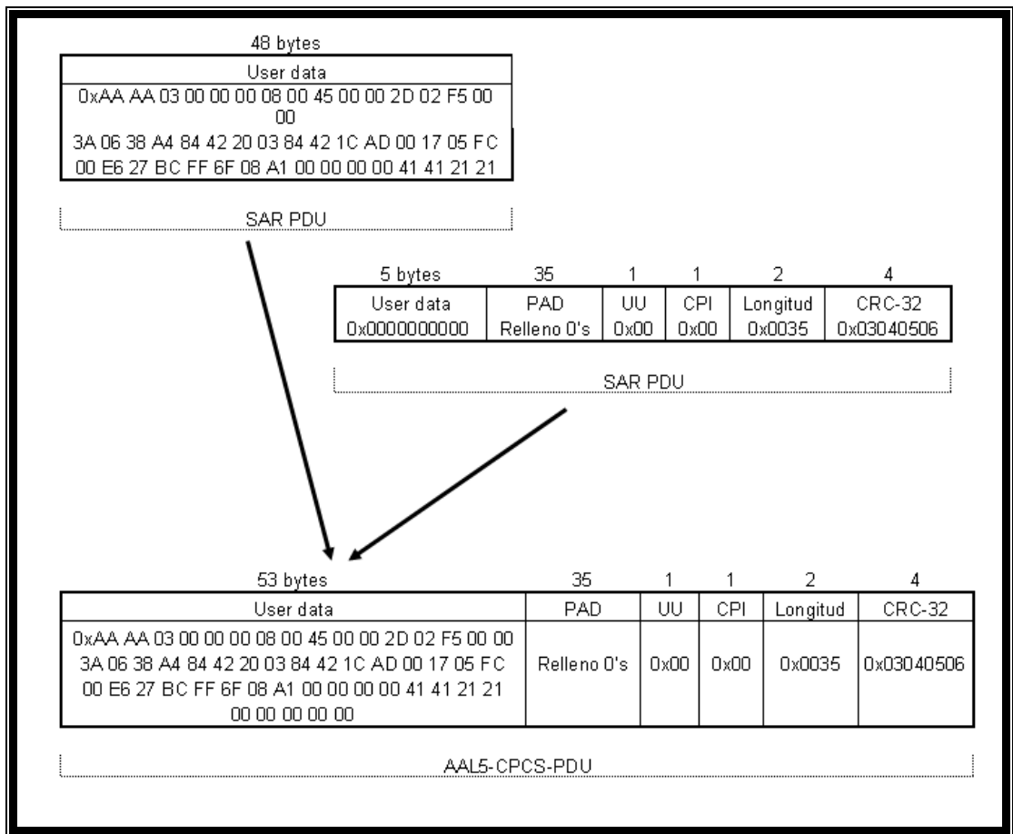
Figura 4.6.7 Reensamble de SAR-PDU en AAL5-CPCS-PDU
