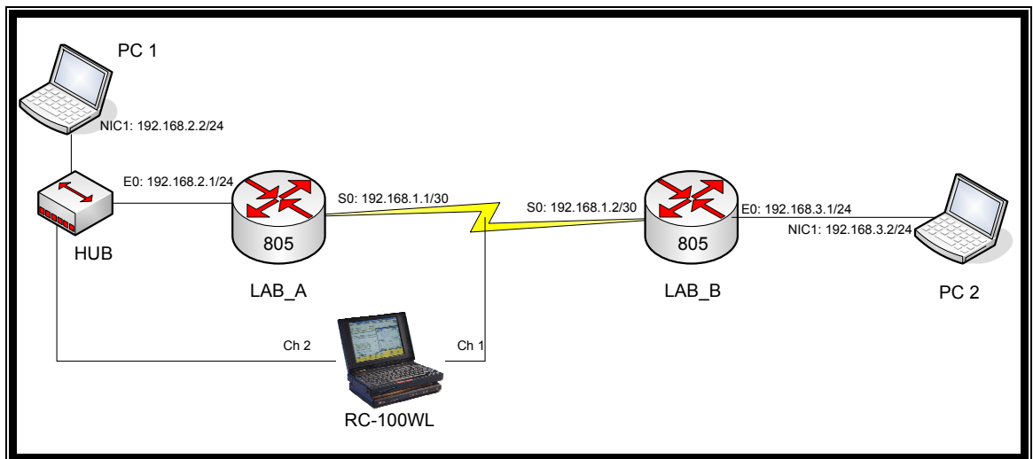
Figura 4.4.1 Diagrama de red
