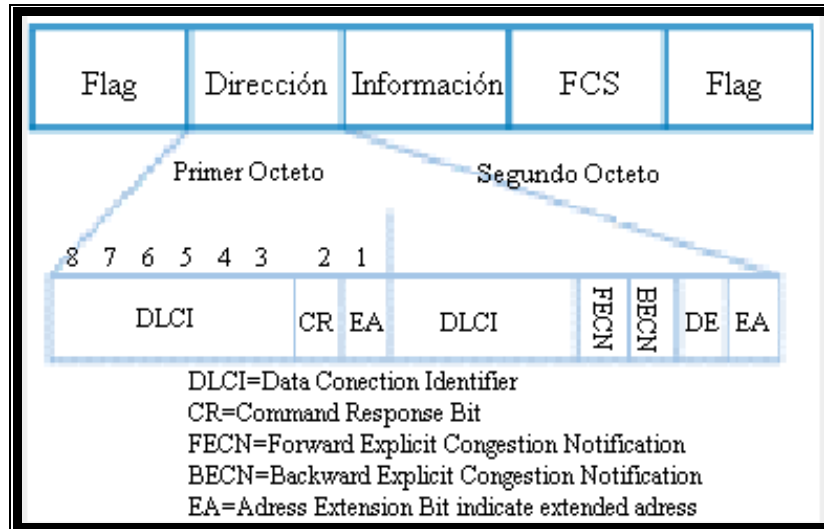
Figura 2.6 Campo de Dirección 9
