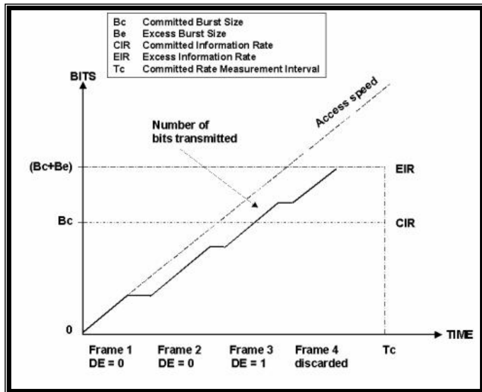
Figura 2.8 Parámetros de frame relay 10
