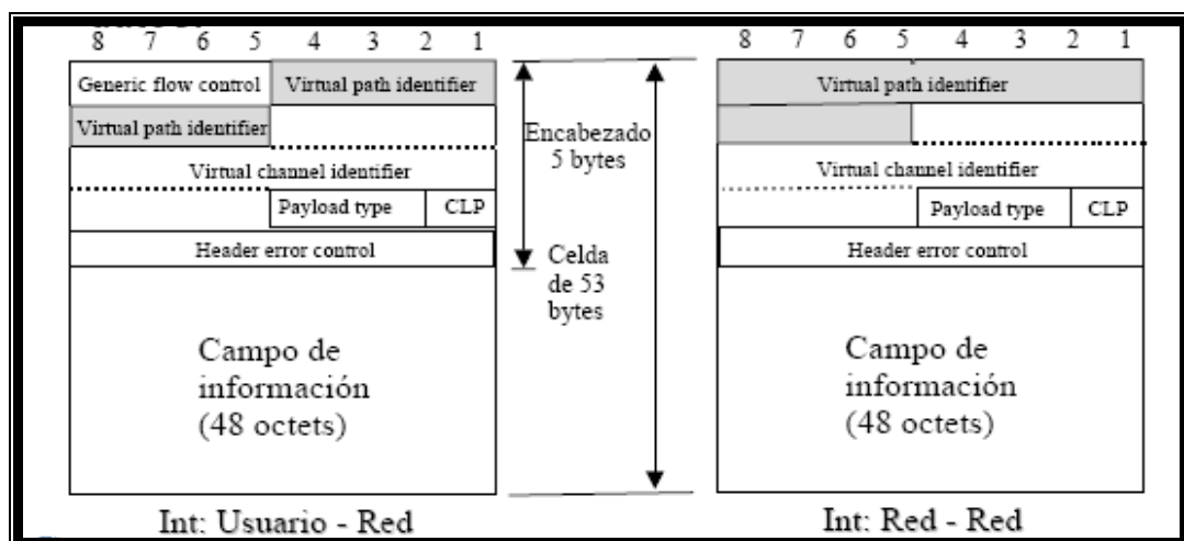
Figura 2.12 Formato de cabecera
