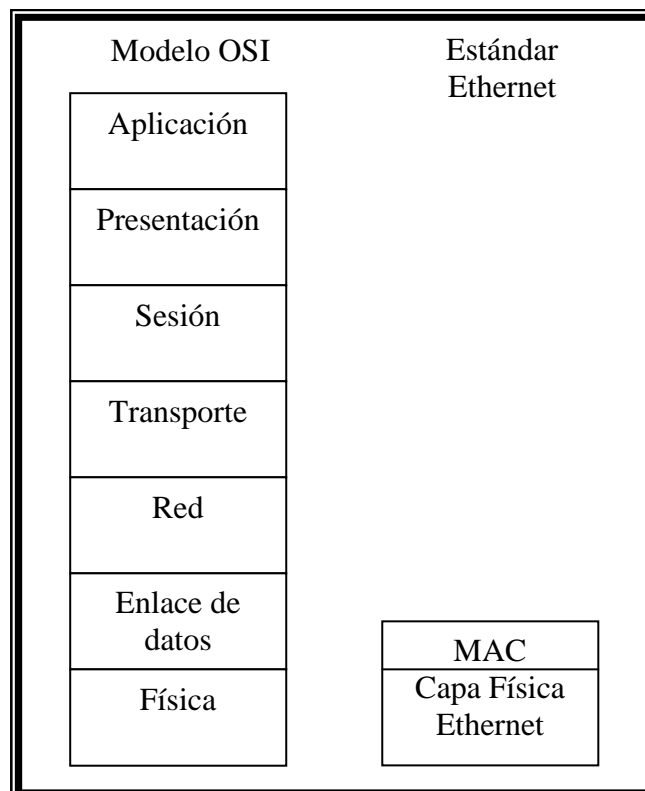
Figura 2.1 Modelo OSI y Ethernet
