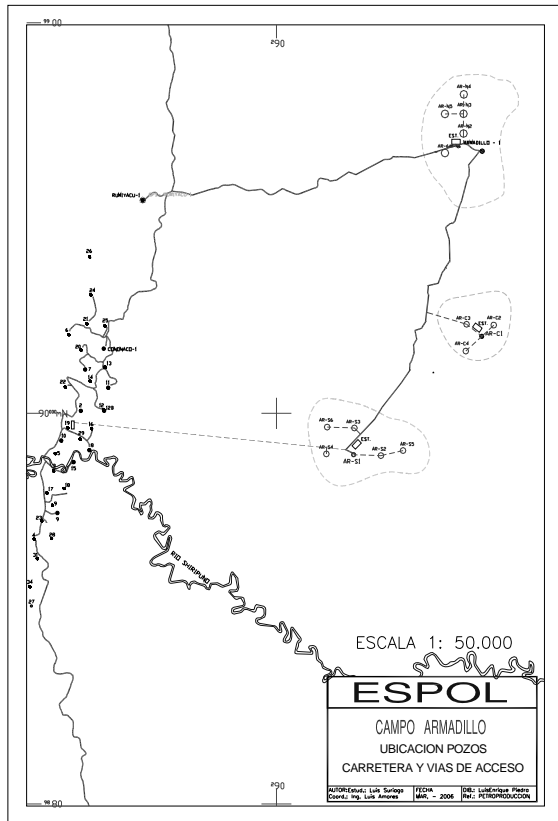
Figura 1. Ubicación de Pozos en el Campo Armadillo
