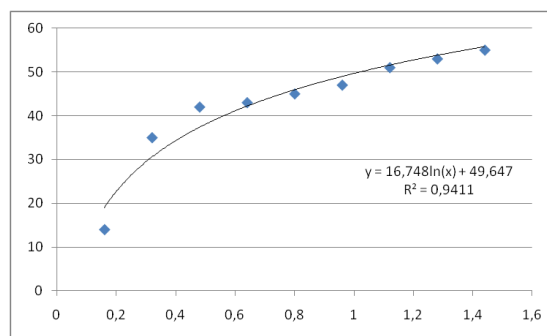
Figura 3. Curva especie – área, bosque muy húmedo pre-montano en Guasaganda.
