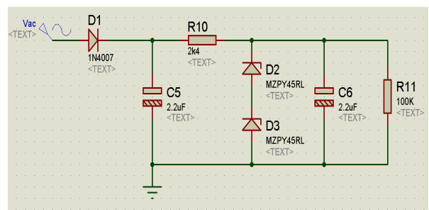
Figura 7 Fuente del fototubo
