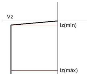
Figura 8 Curva inversa del zener
