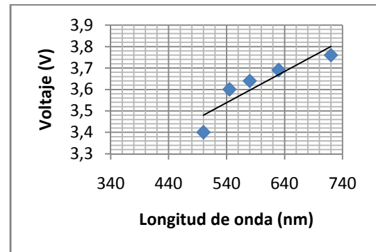
Figura 9 Relación lineal entre voltaje y longitud de onda
