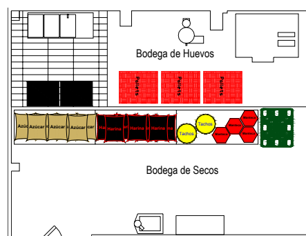
Figura 4.57 Plano Bodegas Externas propuesto
