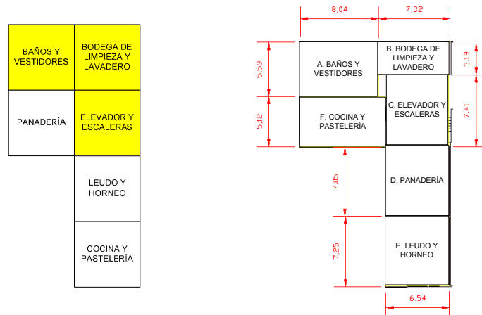
Figura 4.12 Ajuste a dimensiones reales Distribución 3 Planta alta
