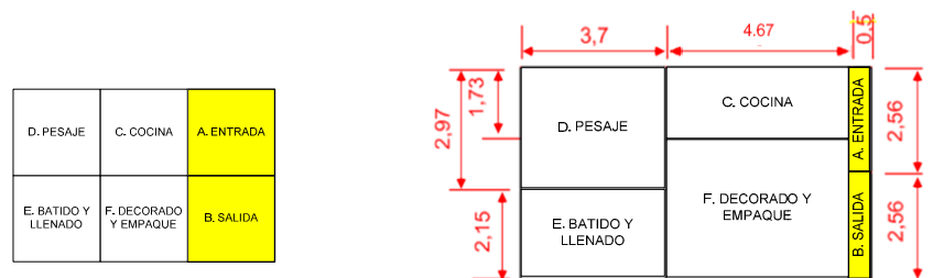
Figura 4.37 Ajuste de dimensiones reales Distribución 1 Pastelería
