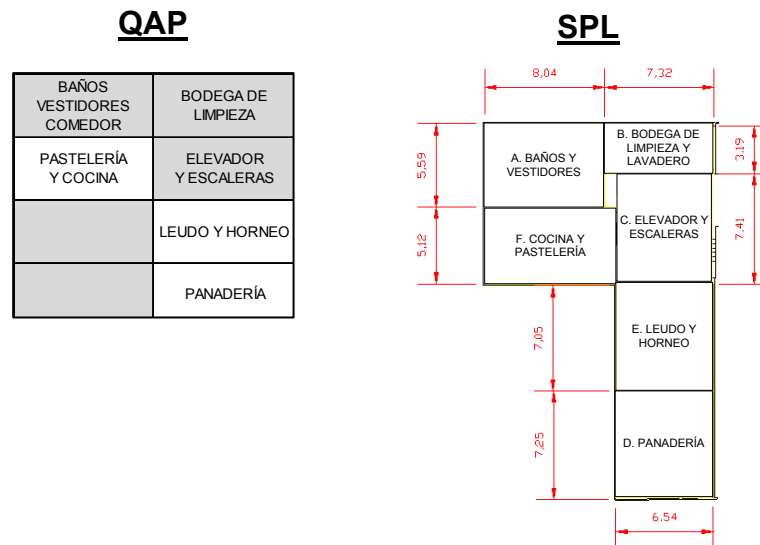
Figura 4.13 Comparación entre método QAP y SPL Planta Alta
