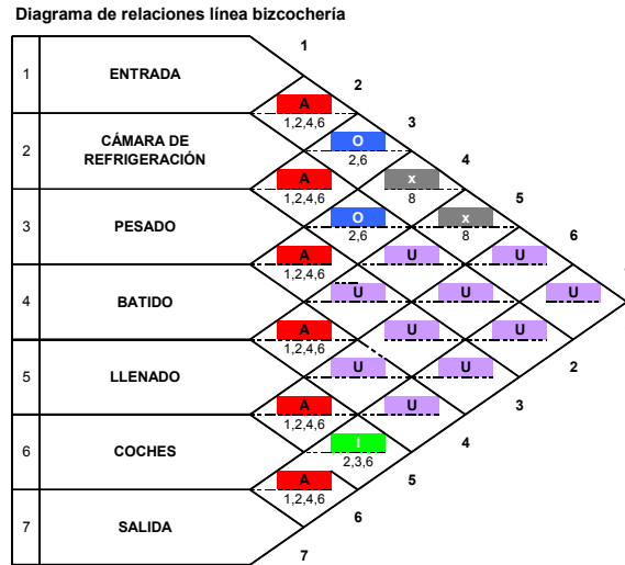
Figura 4.16 Diagrama de relaciones Bizcochería
