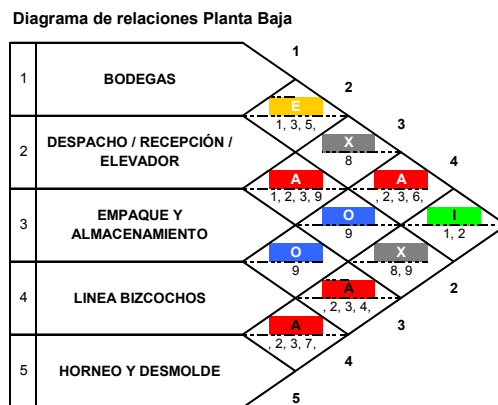
Figura 4.3 Diagrama de relaciones Planta baja
