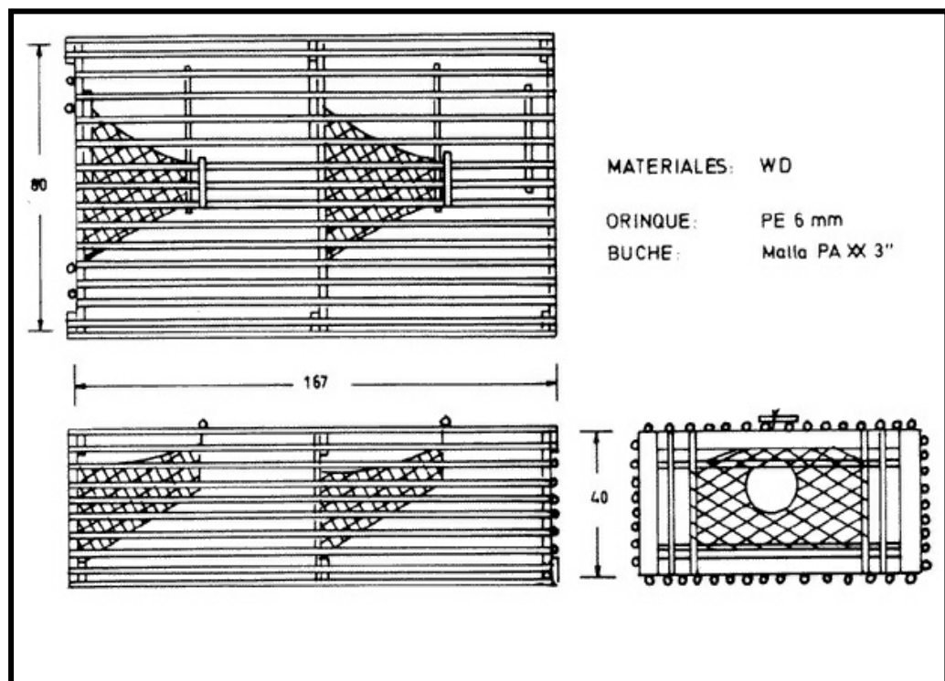
Fuente: www.bibliotecadigital.mx . Figura 6. Arte de pesca tipo trampa.
