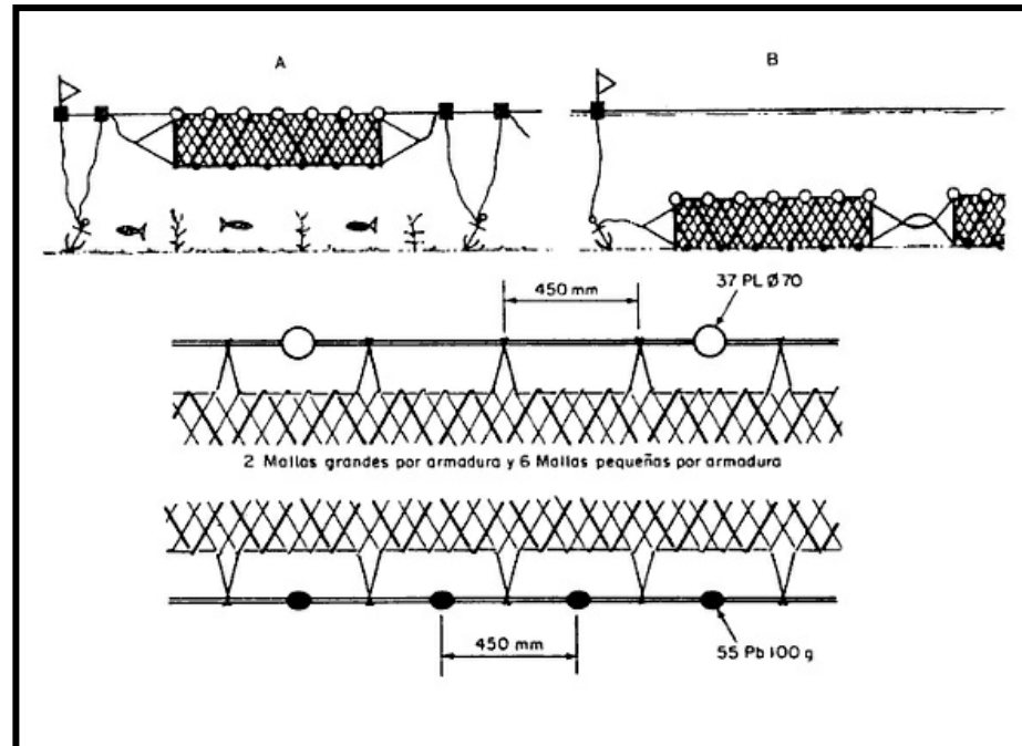
Figura 4. Arte de pesca tipo trasmallo.
