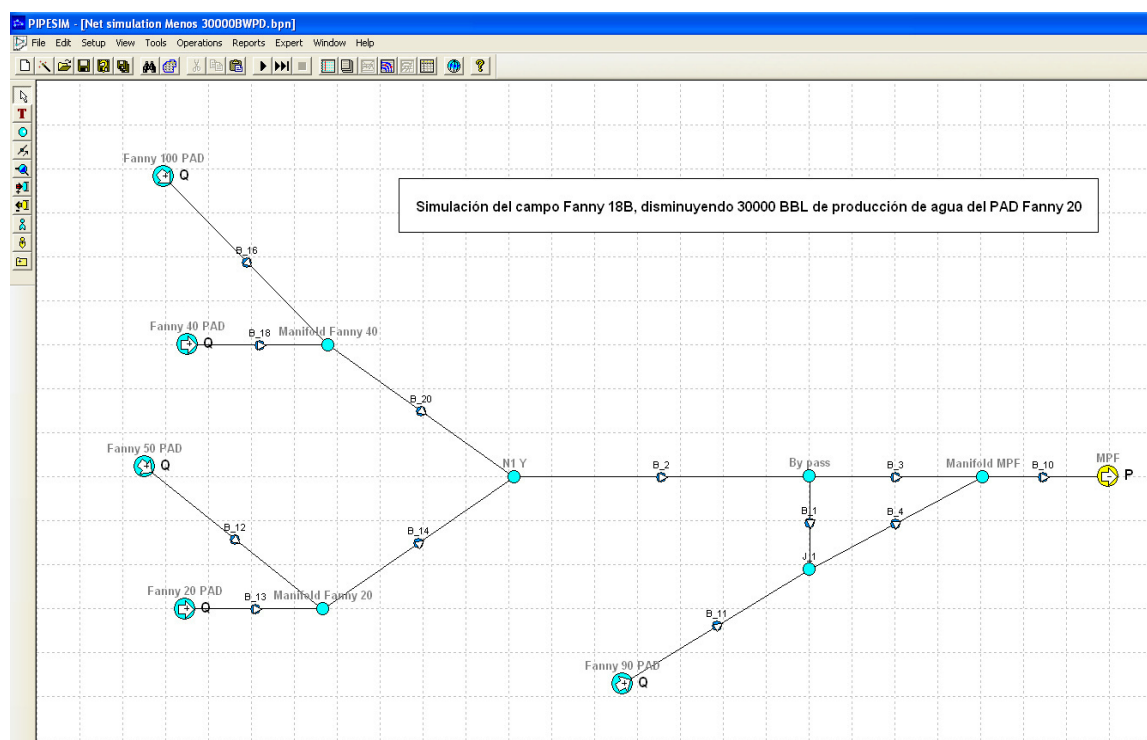
Figura 4-21: Modelo de simulación usando el Software Pipesim Nodal Analysis, logrando disminuir los 30000BWPd que se enviaban desde la plataforma Fanny 20 hasta MPF
