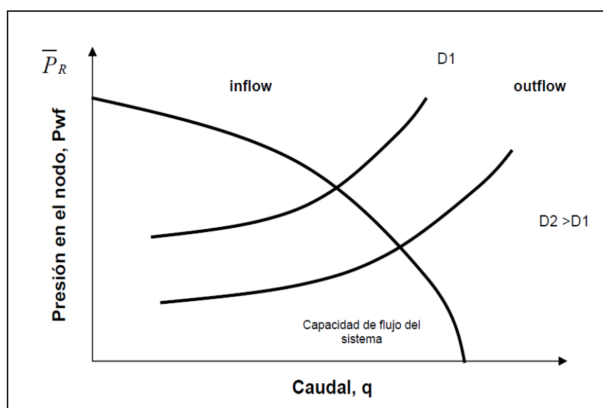
Figura 4-5. Efecto del cambio en los diámetros del tubing sobre la capacidad de flujo.
