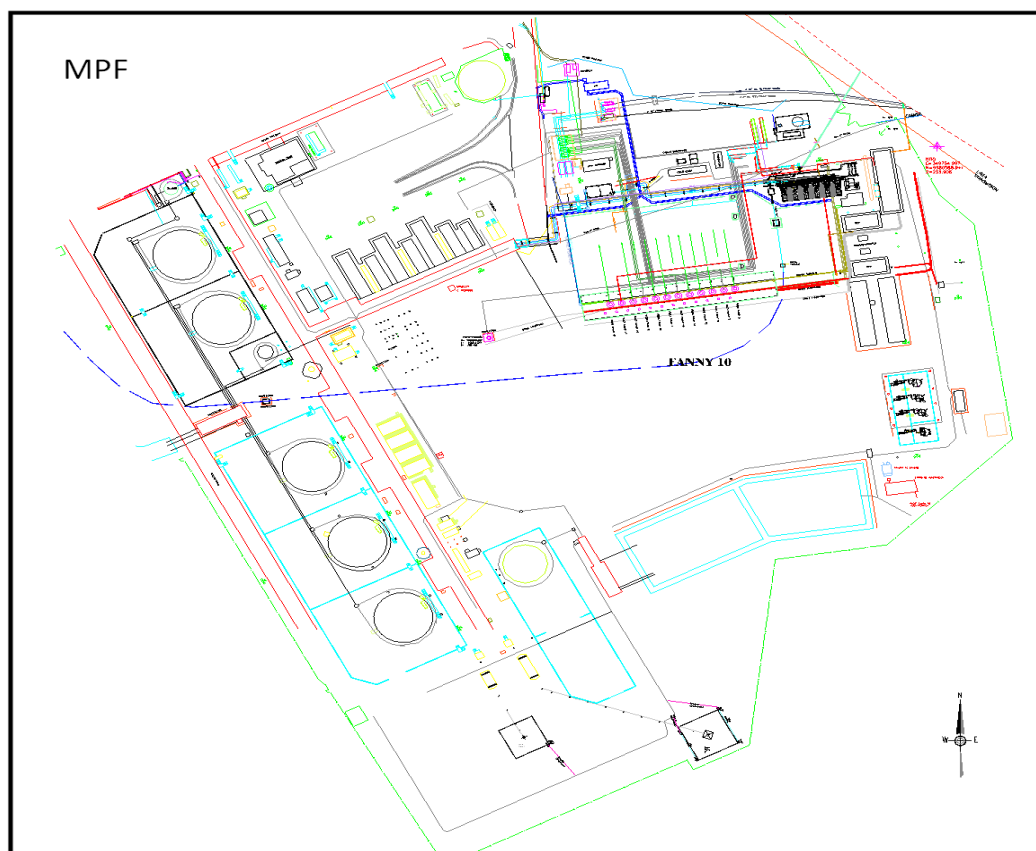
Figura 3-12: Esquema de MPF Facilidades centrales de Producción del Campo Fanny 18B.
