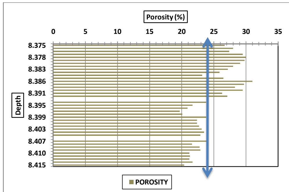
Figura 2-3 Grafico Profundidad vs Porosidad.
