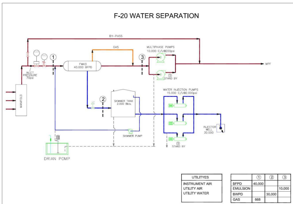
Fig.4-20: Esquema detallado que resulta de la simulación al Incrementar un sistema de producción-inyección en el Well Pad Fanny 20
