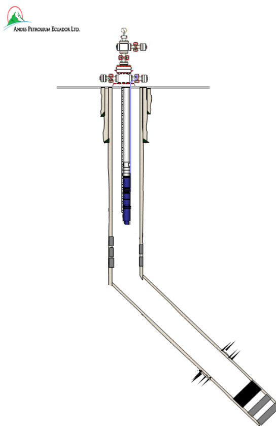
Figura 3-3: Esquema de un Pozo Direccional.
