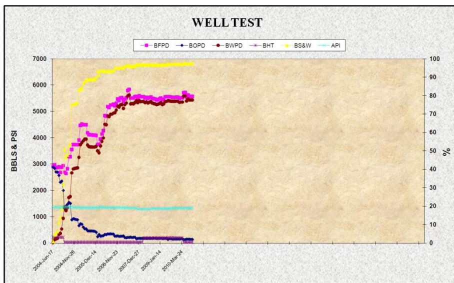
Figura 3-20: Historial de producción Pozo Fanny 18B 31. Fuente: Ingeniería de Producción Andes Petroleum Ecuador Ltd.
