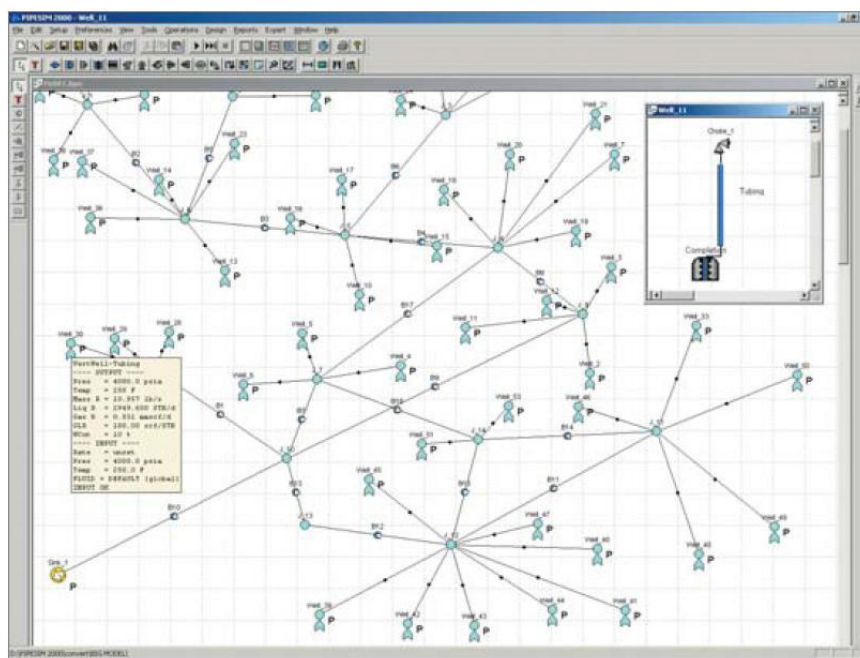
Figura 3-11: La capacidad de PIPESIM puede ampliarse para modelar sistemas complejos desde el yacimiento hasta las instalaciones de superficie con el módulo Network Analysis.
