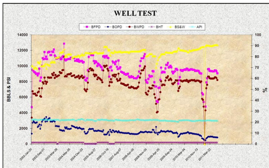
Figura 3-18: Historial de producción del Pozo Fanny 18B 24 H. Fuente: Ingeniería de Producción Andes Petroleum Ecuador Ltd.
