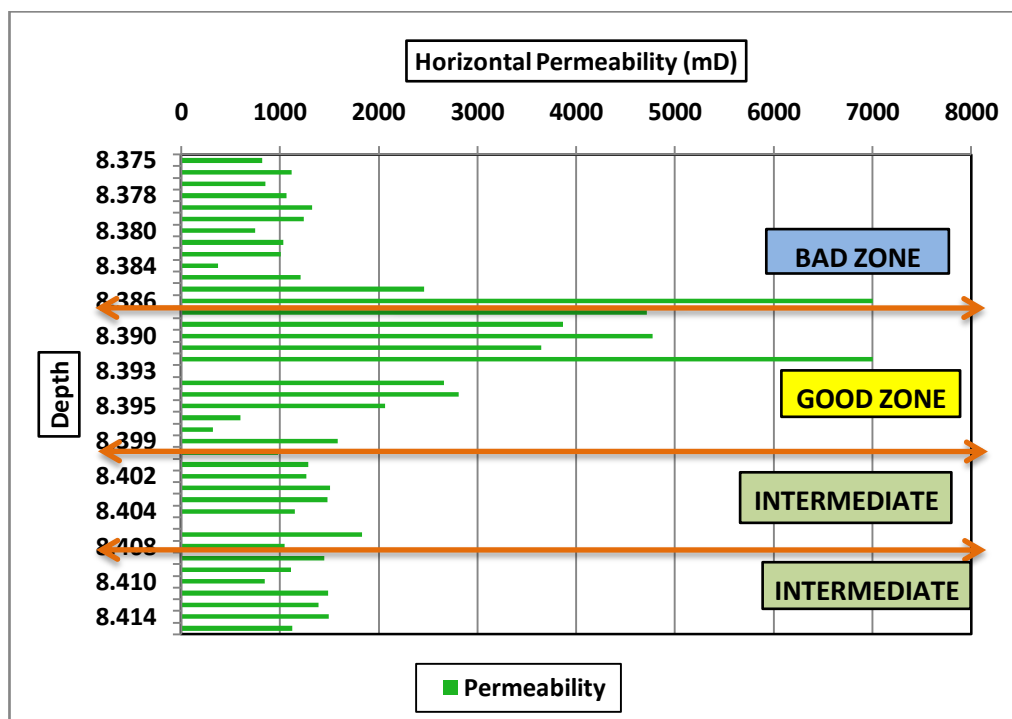
Figura 2-4: Grafico Profundidad vs Permeabilidad Horizontal. Fuente: Ingeniería de Yacimientos Andes Petroleum Ecuador Ltd.
