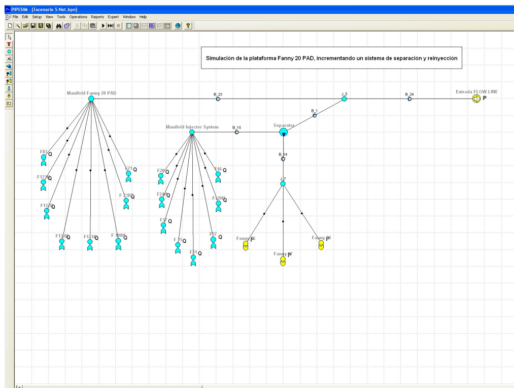
Figura 5-2: Simulación con el Software Pipesim Nodal Analysis de la plataforma Fanny 20, incrementando un sistema de producción-inyección.
