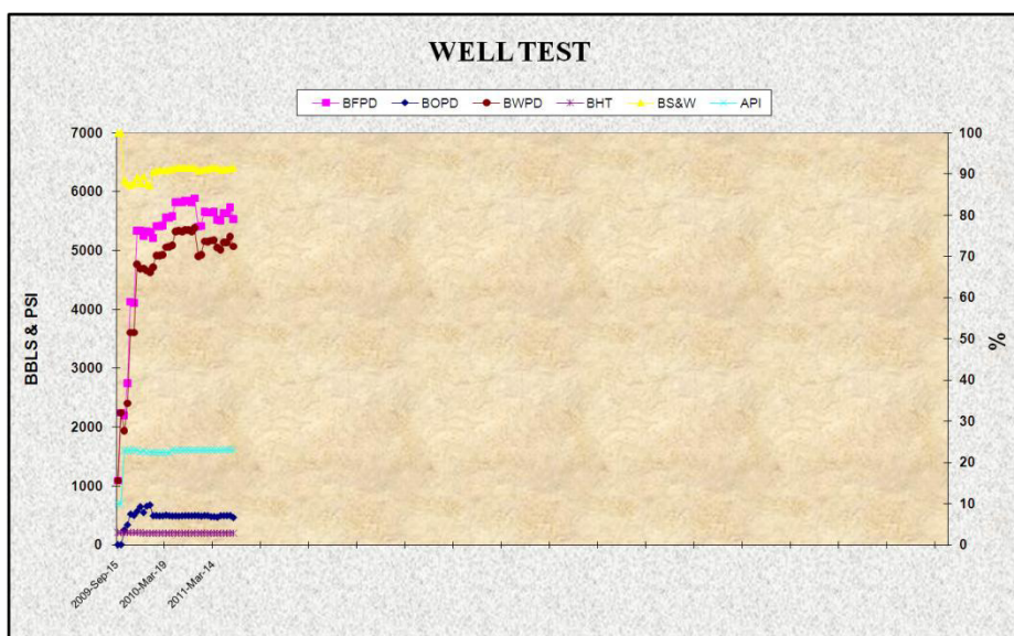
Figura 3-27: Historial de producción del Pozo Fanny 18B 121 H. Fuente: Ingeniería de Producción Andes Petroleum Ecuador Ltd.
