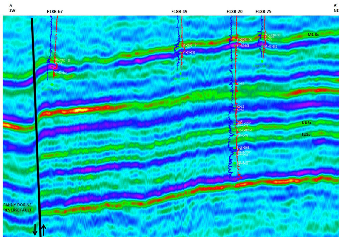
Figura 2-10: Sección sísmica transversal de la arena U inferior del Campo Fanny
