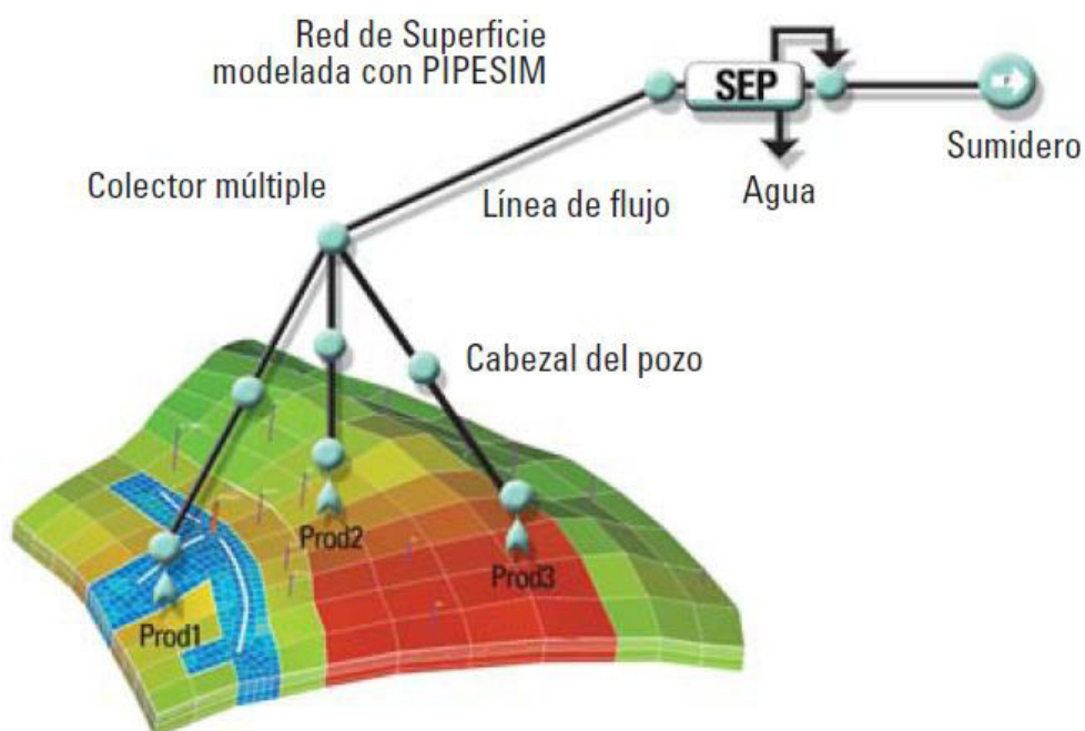
Figura 3-10: Ilustración gráfica de cómo se une el análisis nodal de fondo con las redes de producción en superficie.
