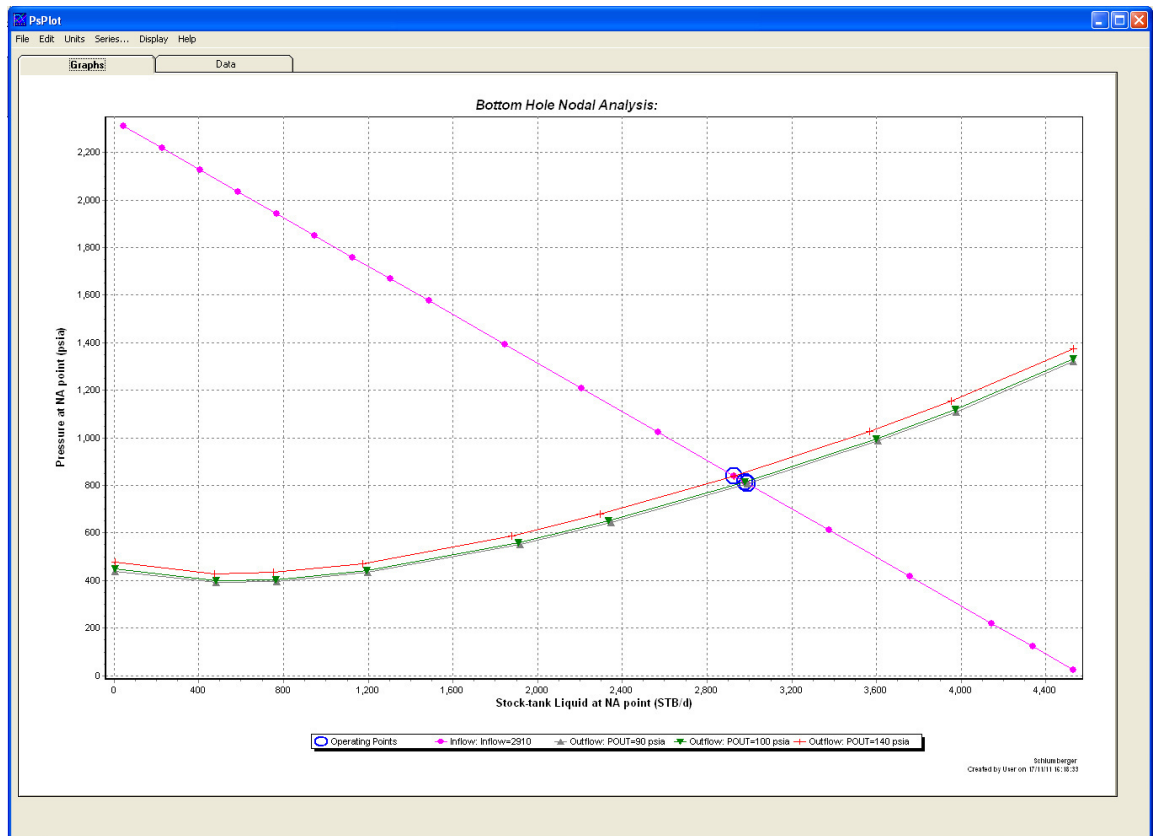
Figura 4-15: Sensibilidades a través de las curvas de comportamiento de afluencia del pozo variando P_{wh}
