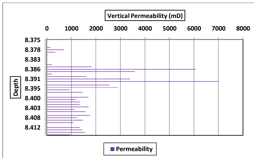
Figura 2-7: Grafico Profundidad vs Permeabilidad vertical.
