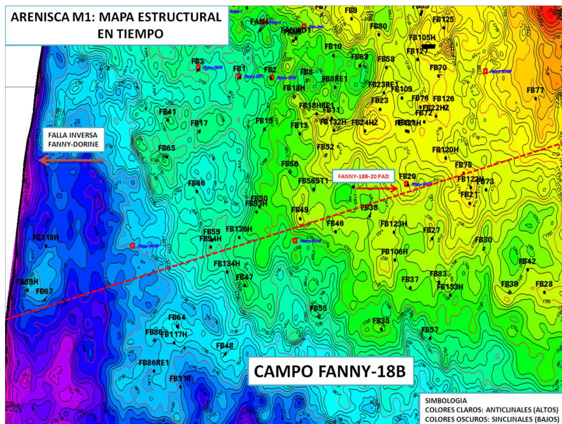
Figura 2-9: Mapa estructural del campo Fanny 18B
