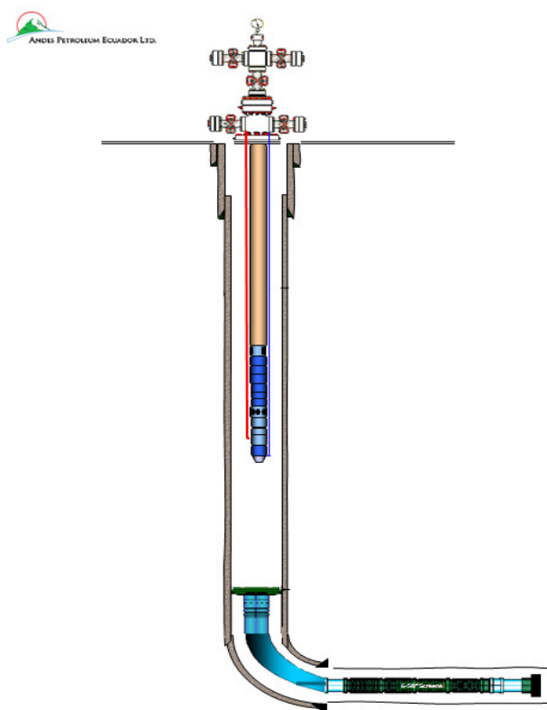
Figura 3-5: Esquema de un Pozo Horizontal.
