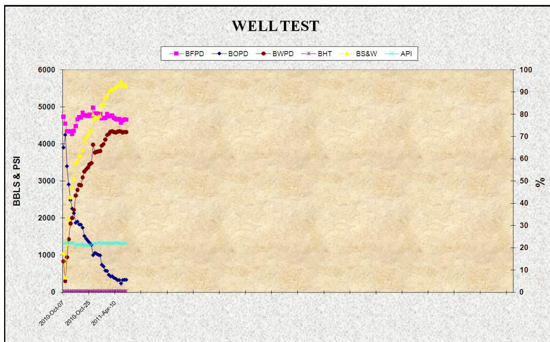
Figura 3-30: Historial de producción del Pozo Fanny 18B 133 H. Fuente: Ingeniería de Producción Andes Petroleum Ecuador Ltd.
