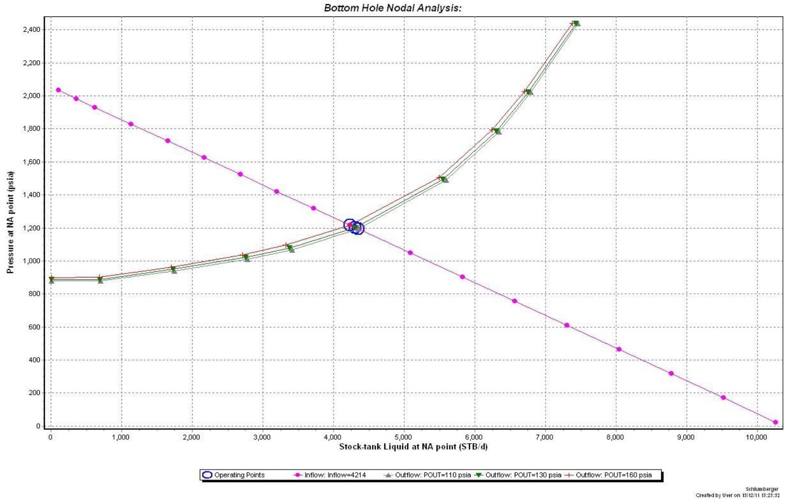
Figura D15: Análisis de sensibilidad del pozo Fanny 18 B 132H
