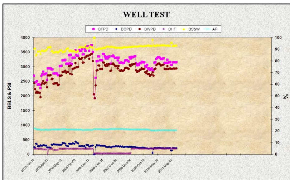
Figura 3-21: Historial de producción del Pozo Fanny 18B 37. Fuente: Ingeniería de Producción Andes Petroleum Ecuador Ltd.
