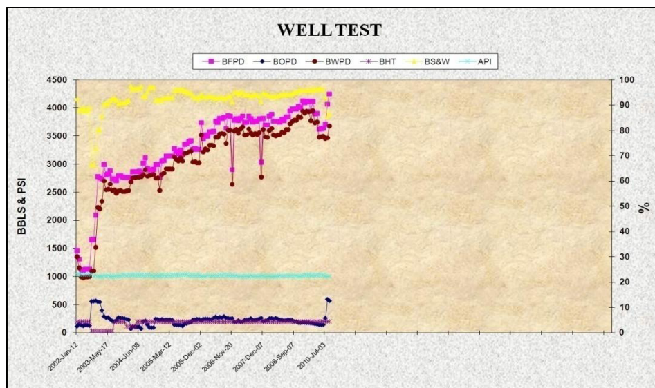
Figura 3-16: Historial de producción del Pozo Fanny 18B 21 Fuente: Ingeniería de Producción Andes Petroleum Ecuador Ltd.
