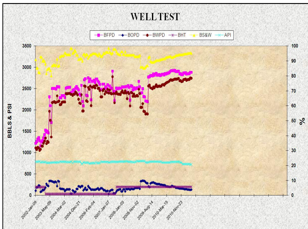
Figura 3-15: Historial de producción del Pozo Fanny 18B 20. Fuente: Ingeniería de Producción Andes Petroleum Ecuador Ltd.
