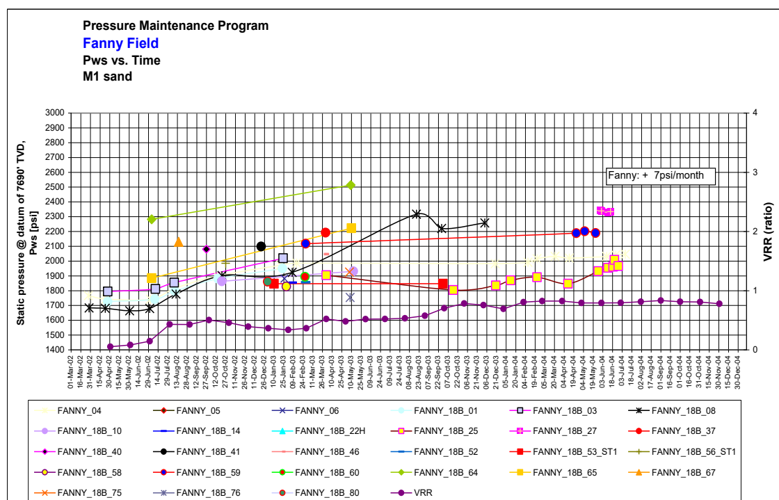
Figura 2-11: Histórico de Presión del Campo Fanny, yacimiento M-1
