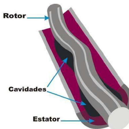
Figura 3-7: Representación gráfica de los componentes principales de la Bomba de Cavidades Progresivas.
