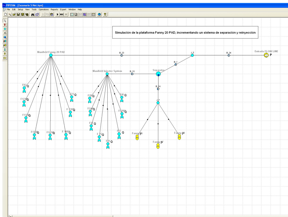
Figura 4-19: Simulación con el Software Pipesim Nodal Analysis de la plataforma Fanny 20, incrementando un sistema de producción-inyección.
