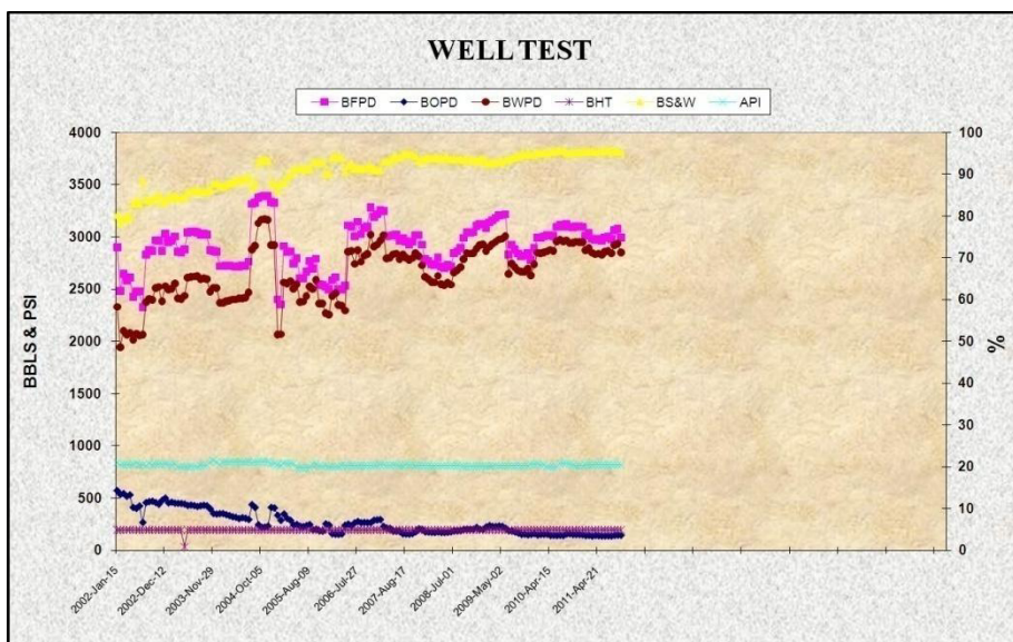
Figura 3-22: Historial de producción del Pozo Fanny 18B 46. Fuente: Ingeniería de Producción Andes Petroleum Ecuador Ltd.
