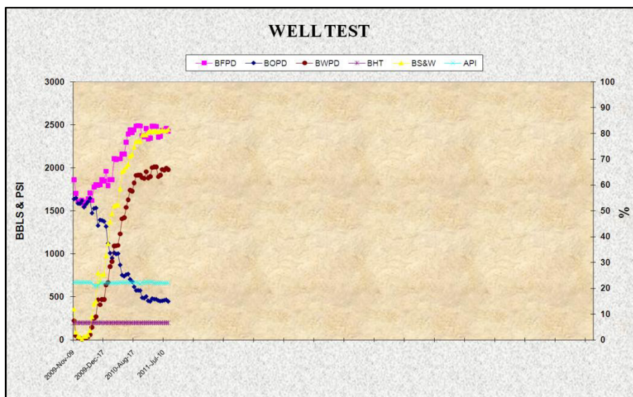
Figura 3-28: Historial de producción del Pozo Fanny 18B 123 H. Fuente: Ingeniería de Producción Andes Petroleum Ecuador Ltd.
