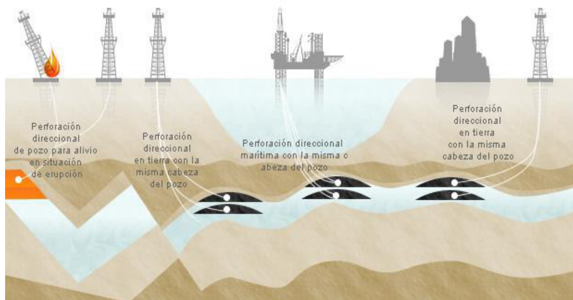
Figura 3-4. Representación gráfica de los beneficios de contar con pozos direccionales
