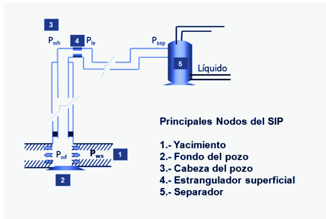
Figura 1-1. Componentes principales para el análisis nodal.
