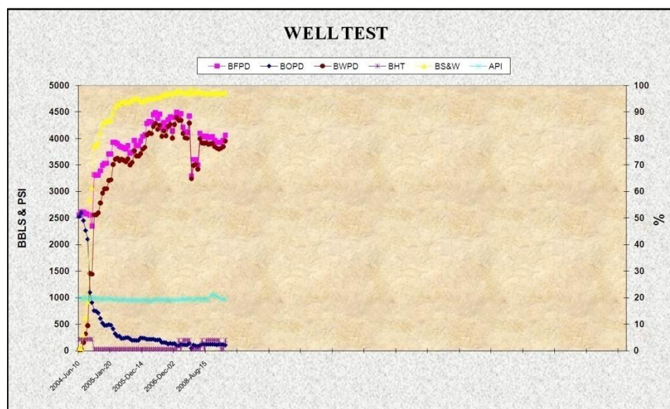
Figura 3-17: Historial de producción del Pozo Fanny 18B 23 RE Fuente: Ingeniería de Producción Andes Petroleum Ecuador Ltd.
