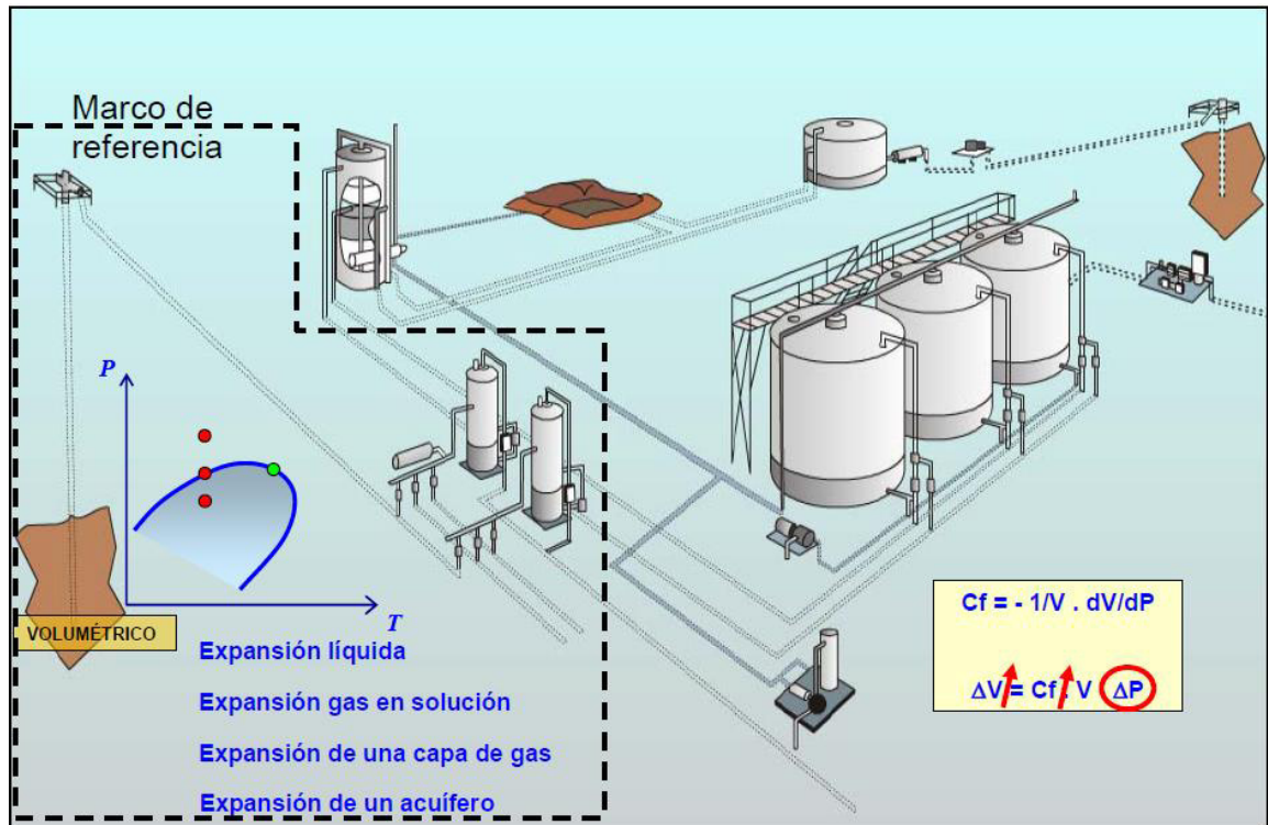
Figura 1-2. Marco de referencia donde se aplicará la metodología de optimización.
