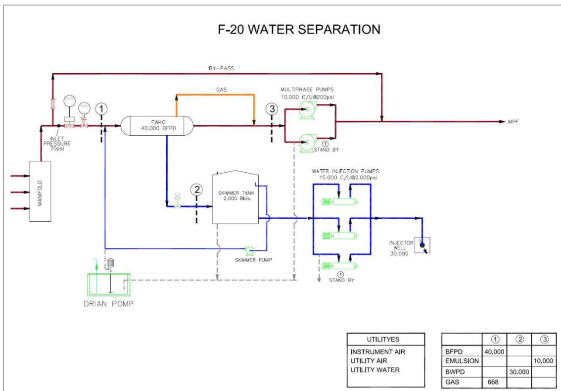
Fig.5-1: Esquema detallado que resulta de la simulación al Incrementar un sistema de producción-inyección en el Well Pad Fanny 20
