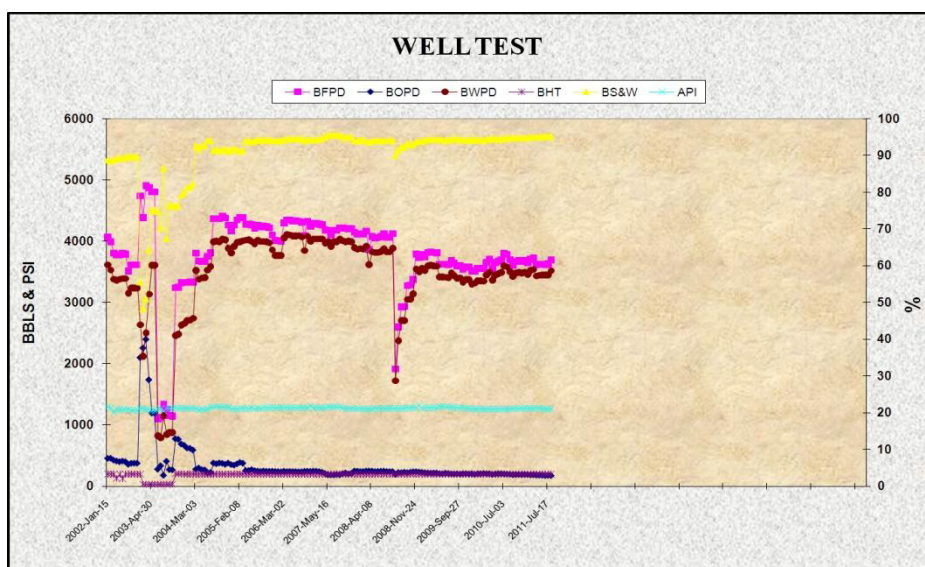
Figura 3-23: Historial de producción del Pozo Fanny 18B 57. Fuente: Ingeniería de Producción Andes Petroleum Ecuador Ltd.
