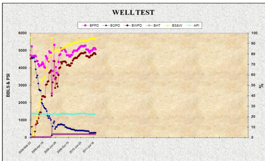
Figura 3-26: Historial de producción del Pozo Fanny 18B 120 H. Fuente: Ingeniería de Producción Andes Petroleum Ecuador Ltd.
