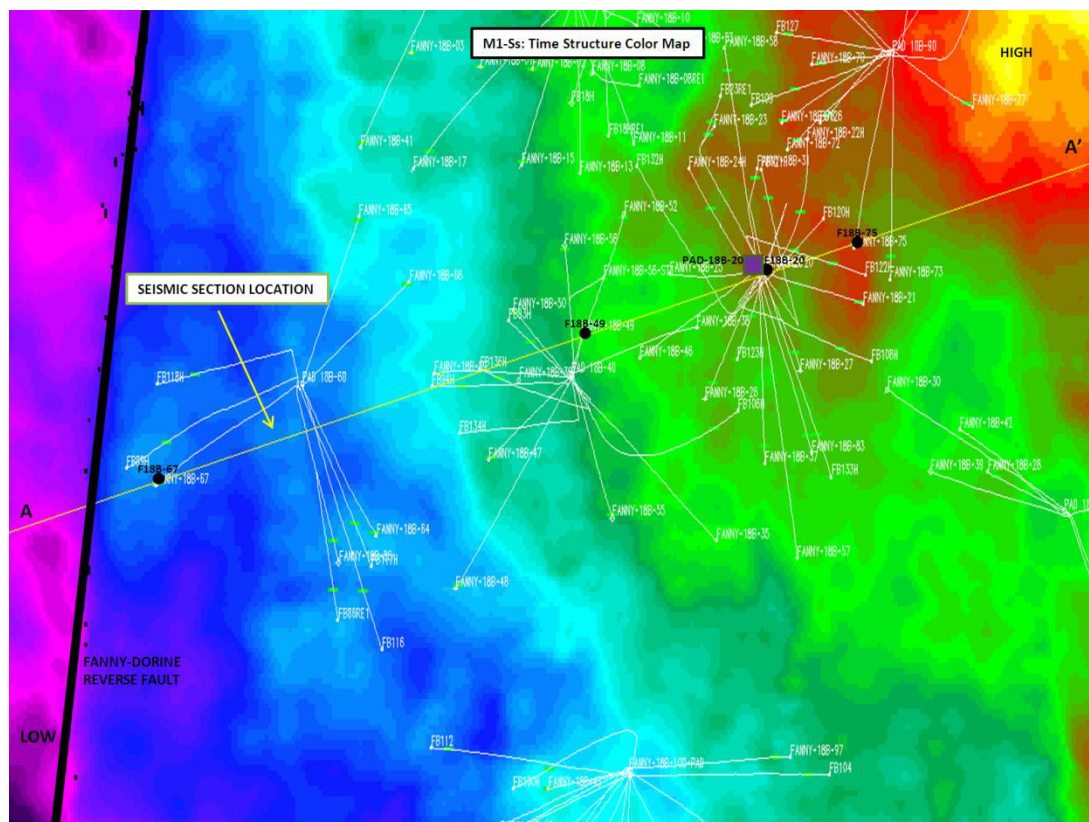
Figura 2-8: Interpretación sísmica del campo Fanny 18B
