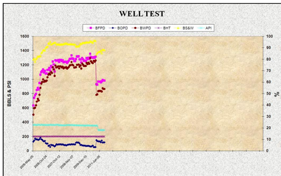
Figura 3-24: Historial de producción del Pozo Fanny 18B 83. Fuente: Ingeniería de Producción Andes Petroleum Ecuador Ltd.
