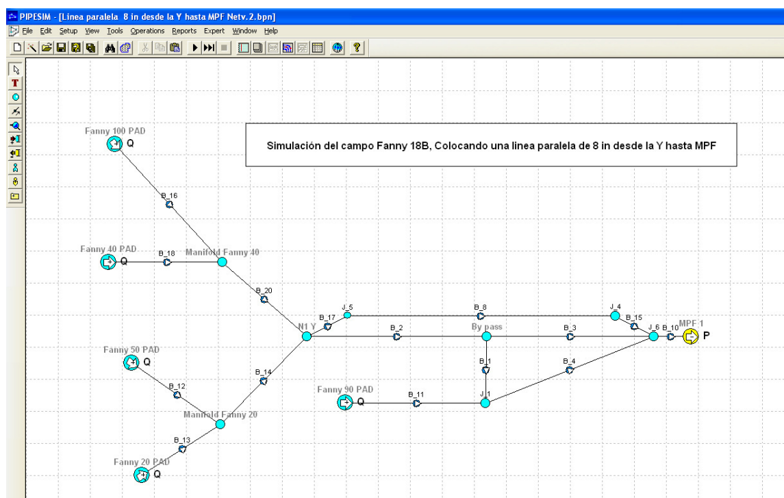
Figura 4-22: Simulación del comportamiento de las redes de flujo y la producción de fluido cuando se coloca una línea paralela desde la Y hasta MPF
