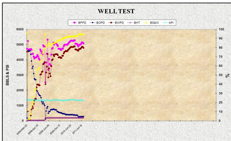
Figura 3-25: Historial de producción del Pozo Fanny 18B 108 H. Fuente: Ingeniería de Producción Andes Petroleum Ecuador Ltd.
