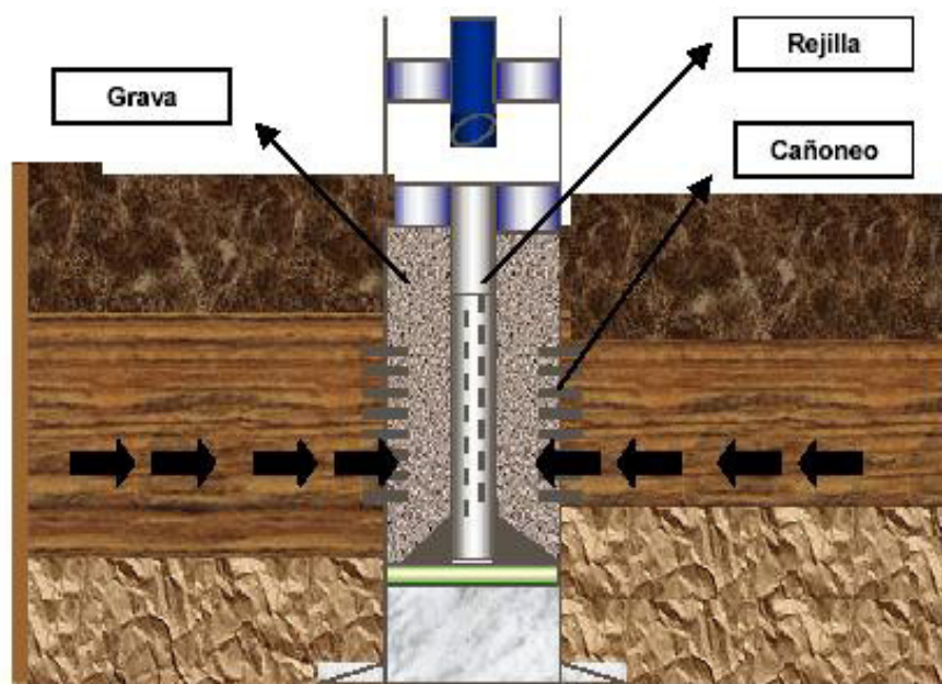
Figura 3-1. Esquema de un Empaque con Grava en Hoyo Revestido.
