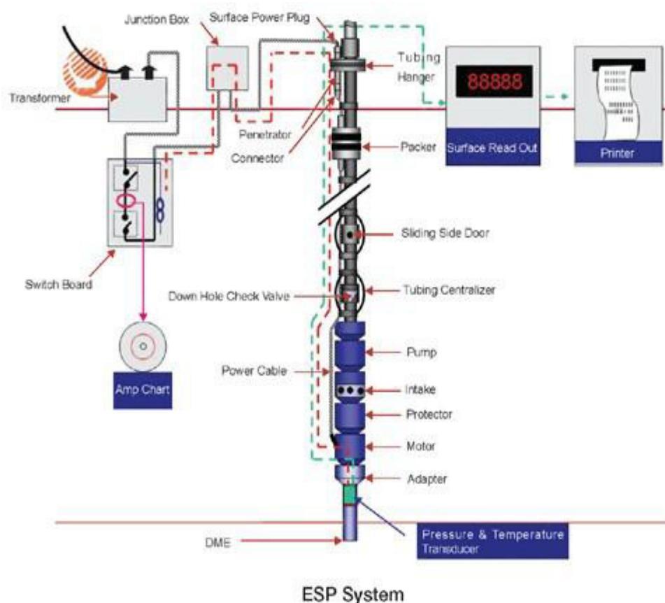
Figura 3-9: Componentes del equipo ESP
