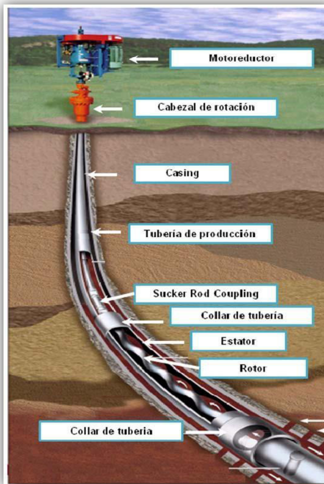
Figura 3-8: Representación grafica de una Completación de producción con Bomba de Cavidades Progresivas.
