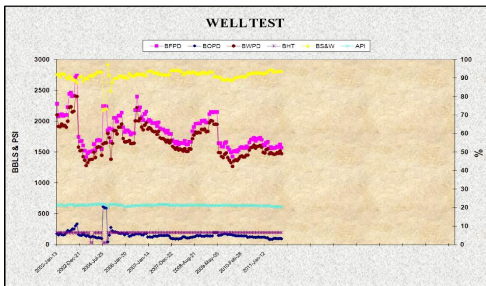
Figura 3-19: Historial de producción del pozo Pozo Fanny 18B 25. Fuente: Ingeniería de Producción Andes Petroleum Ecuador Ltd.
