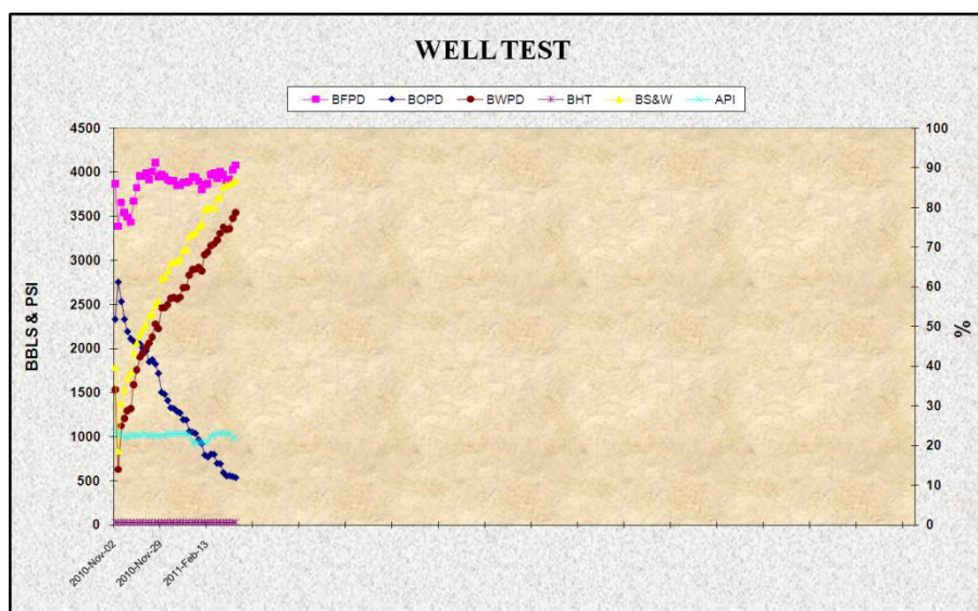
Figura 3-29: Historial de producción del Pozo Fanny 18B 132 H. Fuente: Ingeniería de Producción Andes Petroleum Ecuador Ltd.
