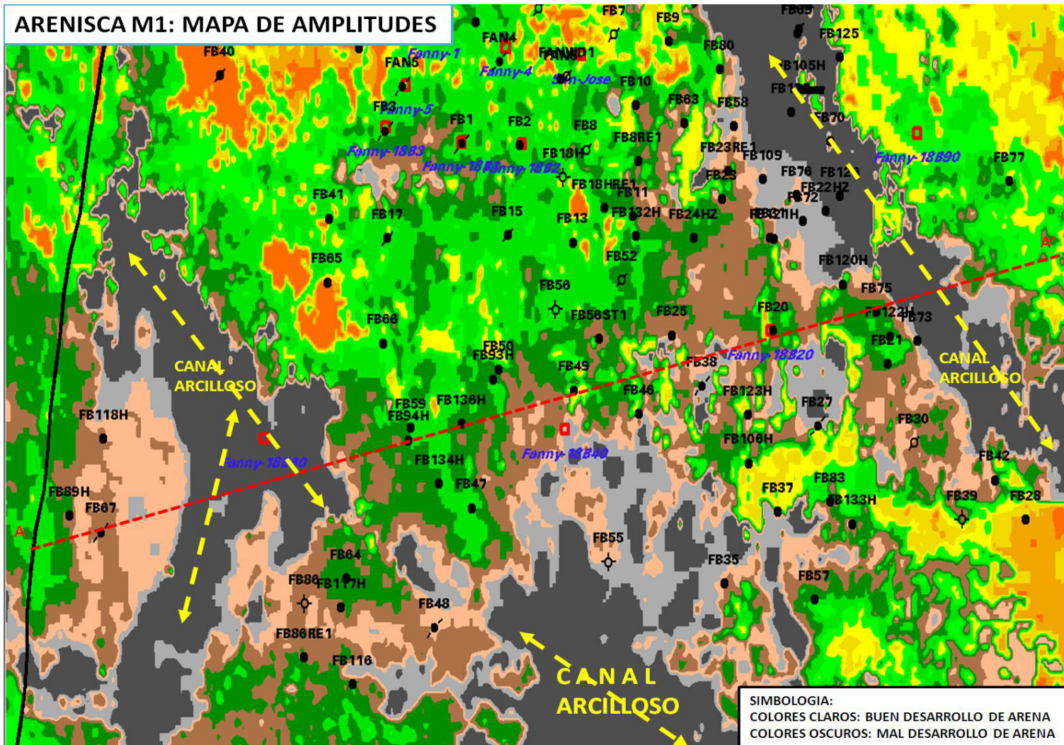
Figura A-II: Mapa de amplitudes de la arenisca M1
