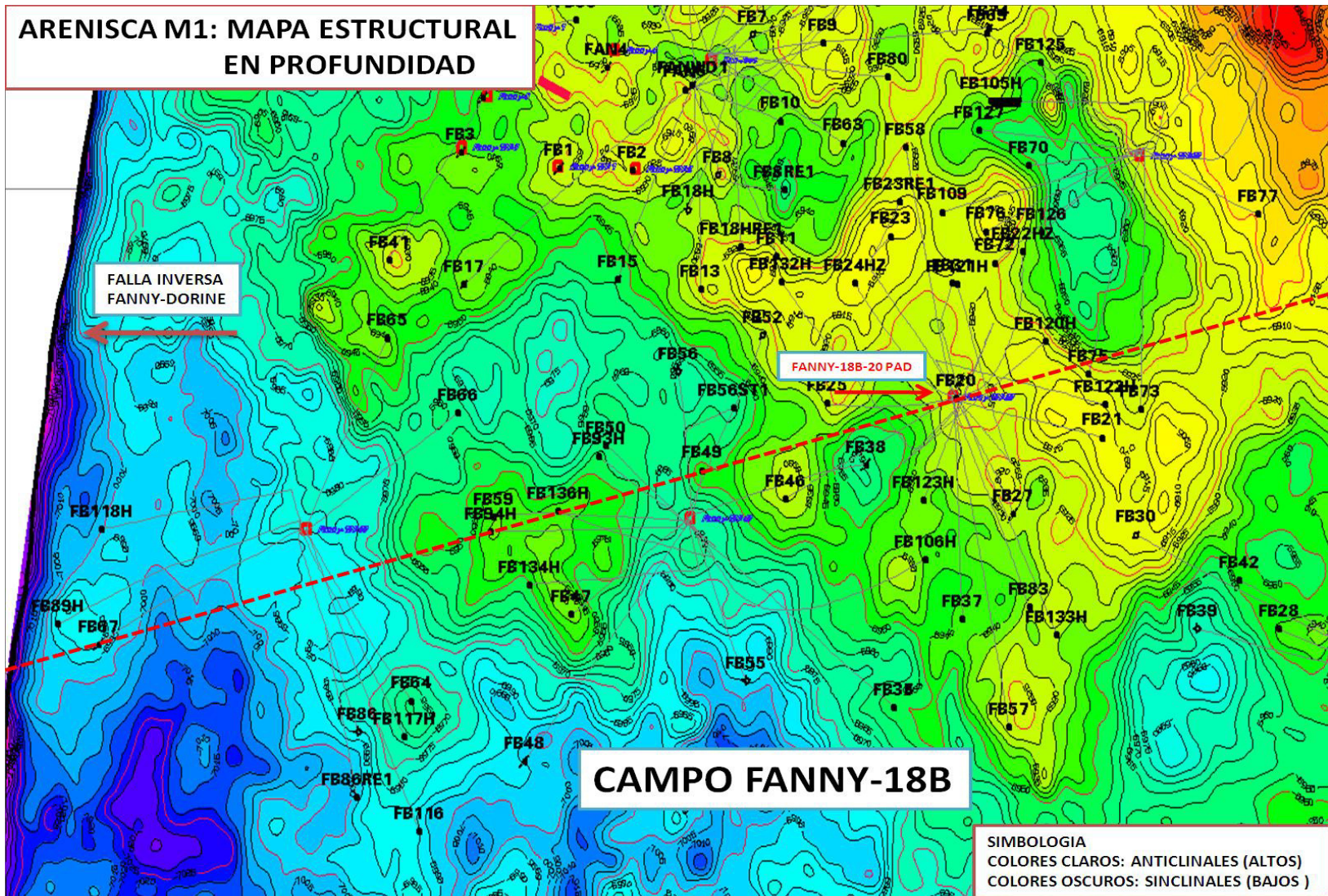
Figura A-II: Mapa estructural en profundidad de la arenisca M1
