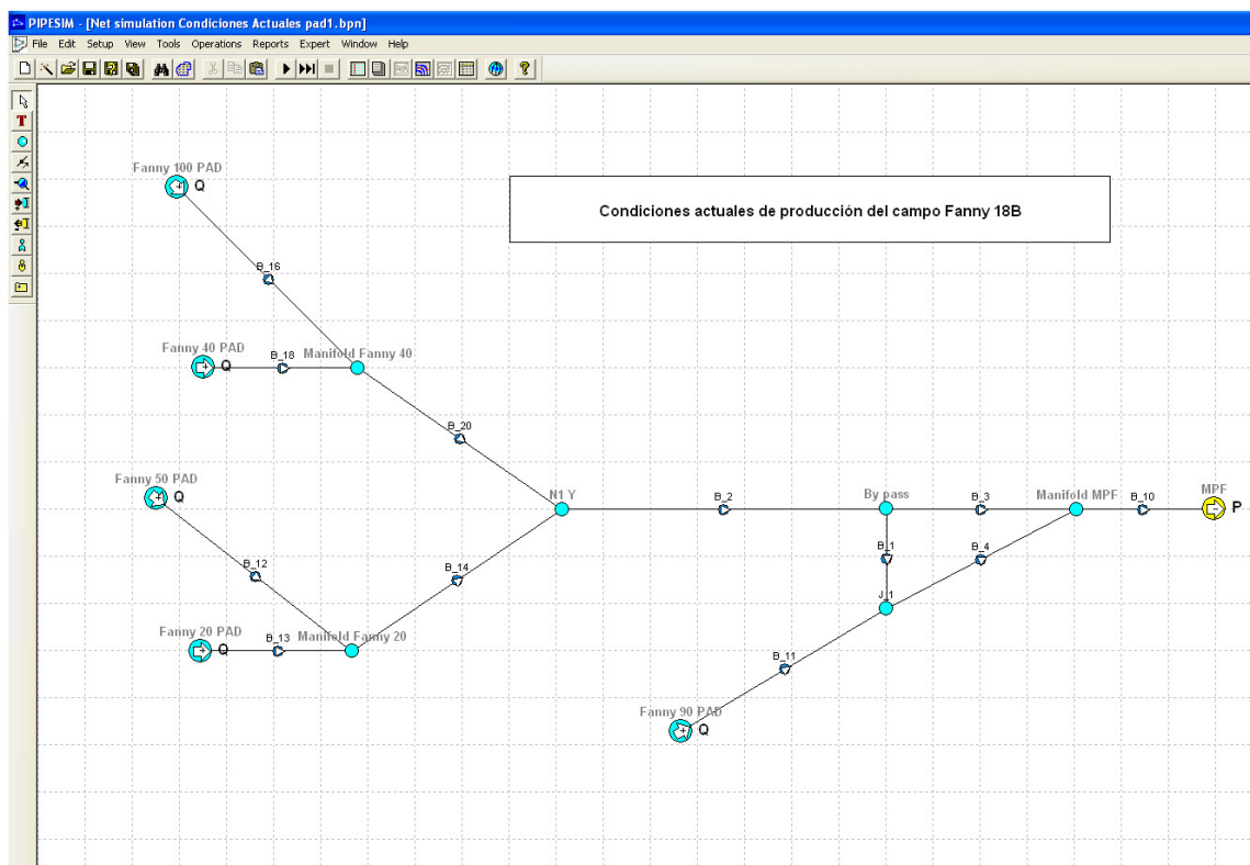
Figura 4-20: Modelo de simulación a condiciones actuales del campo Fanny 18B, usando el Software Pipesim Nodal Analysis
