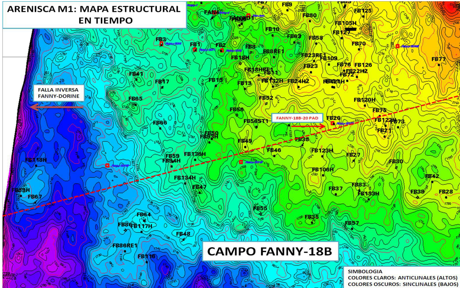
Figura A-I: Mapa estructural en tiempo de la arenisca M1
