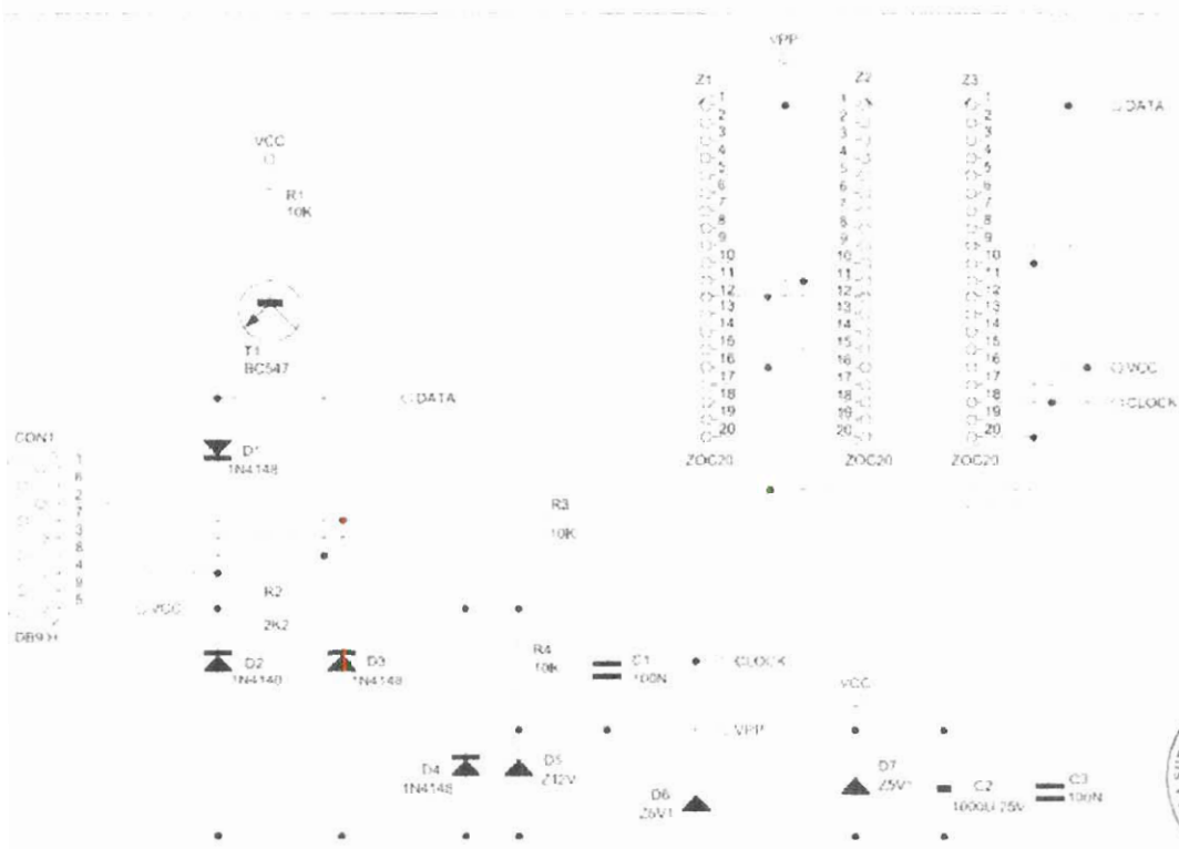
Fig13. Dispositivo Grabador de Pícs
