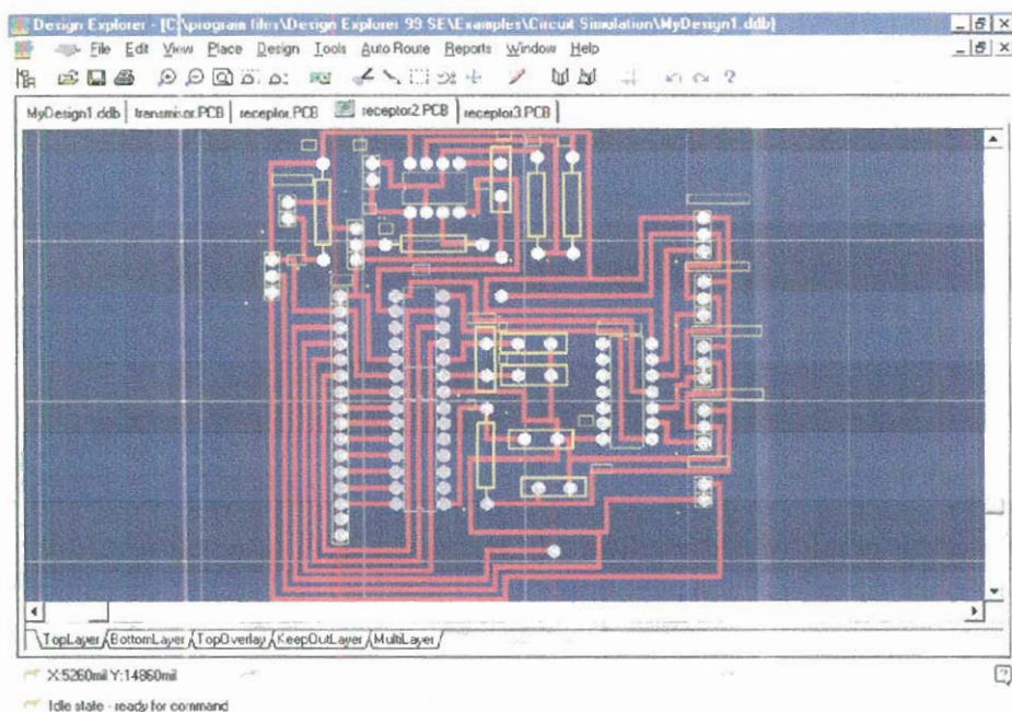
Fig12. Pantalla PROTEL
