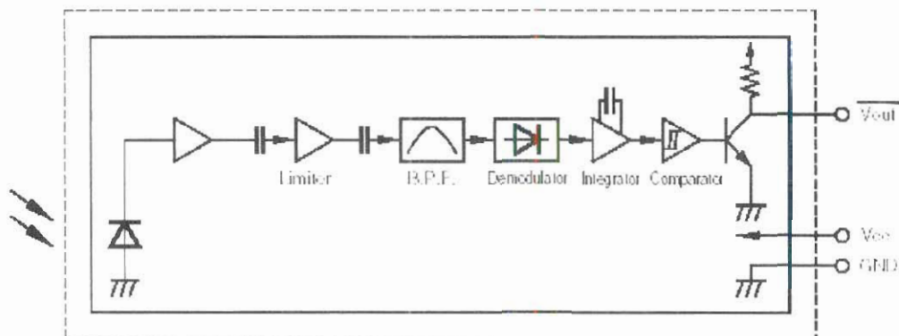
Fig2. Diagrama de Bloques Módulo Receptor Infrarrojo
