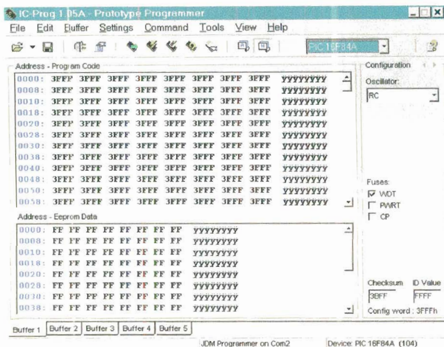
Fig11. Pantalla ICPROG
