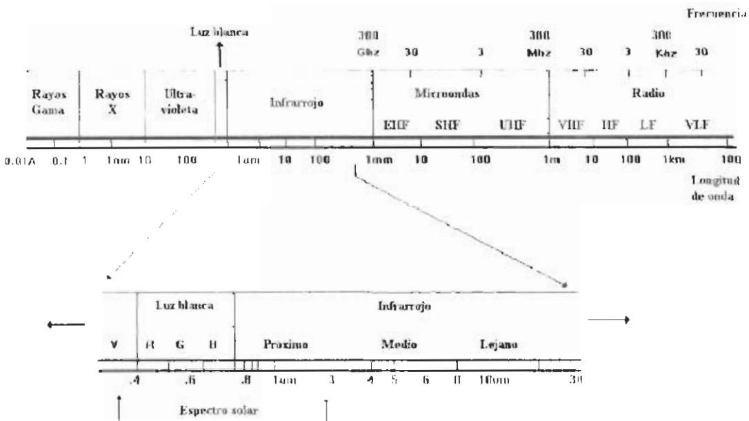
Fig1. Espectro Electromagnético
