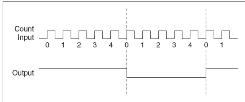
Figura 32.- Salida de un canal seteado en modo Toggle, Reset On
