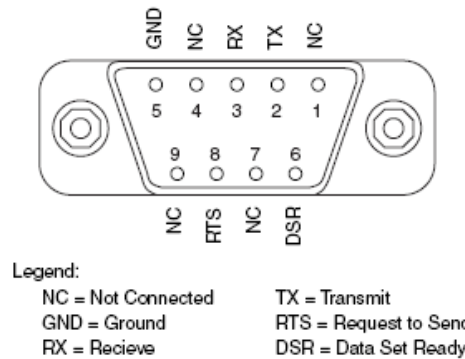
Figura 13.- Conector RS-232 del cFP-1804
