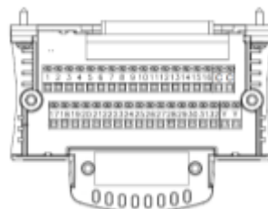
Figura 3.8 Vista interna de un módulo cFP-CB-01 junto a una tabla de asignación de terminales del módulo cFP-AI-100
