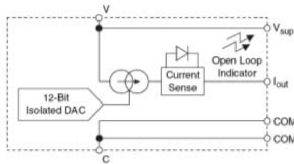
Figura 15.- Circuito de corriente de salida del cFP-AO-200
