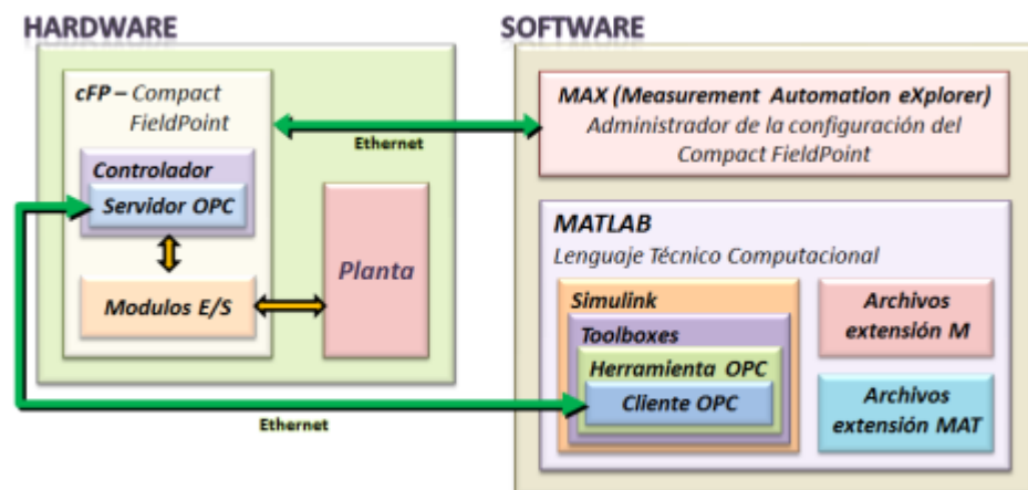
Figura 2.13 Arquitectura de control del proyecto de tesis
