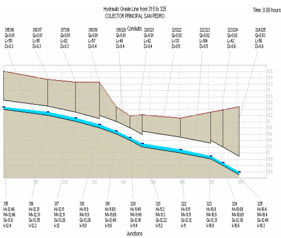
Figura 4. Línea del Gradiente Hidráulico
