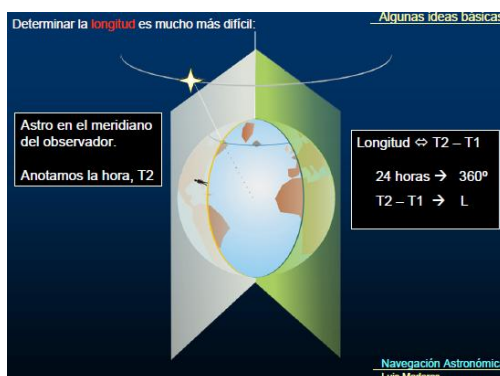
Figura No 12. Determinación de la Longitud Asumida 12
