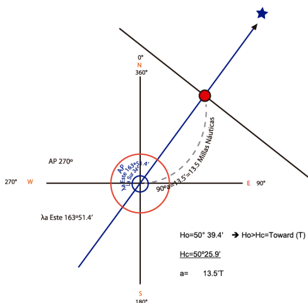
Fig. No 18. Procedimiento de integración de las Determinantes de la Recta de Altura. 19
