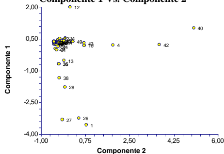
Gráfico 4.1 Análisis por Grupo de Edades Área 2 – Año 2003 Representación de las Enfermedades Componente 1 Vs. Componente 2
