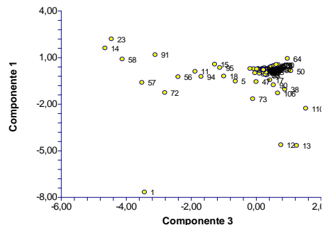
Gráfico 4.2 Análisis por Grupo de Edades Área 2 – Año 2003 Representación de las Enfermedades Componente 1 Vs. Componente 3
