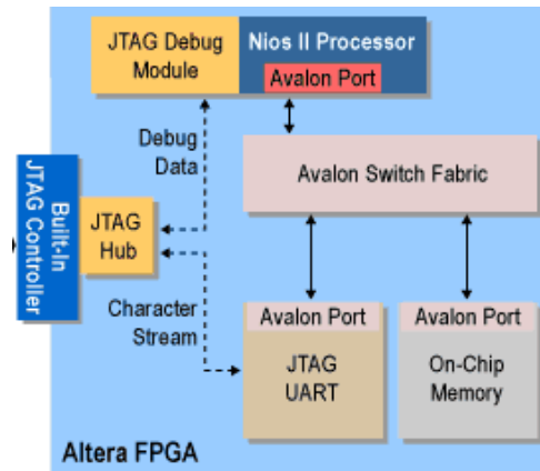
Figura 3. Sistema Elemental con NIOS II System [3]
