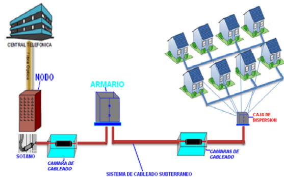
Figura 5 Red de Planta Externa
