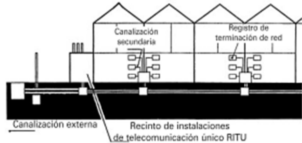
Figura 9 Instalación de las Cajas de Dispersión
