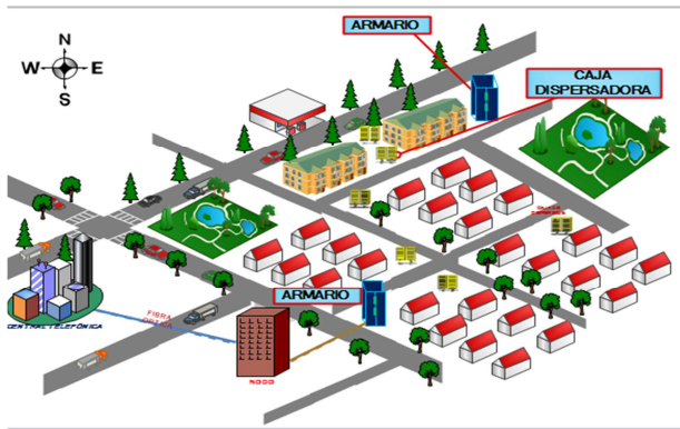
Figura 3 Diseño de Planta Externa en Urbanización
