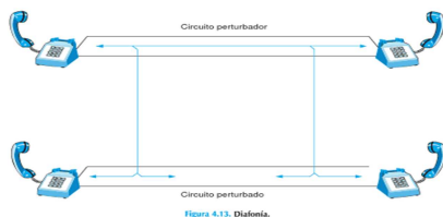
Figura 16 Diafonía
