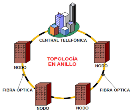
Figura 4 Red Telefónica -Topología Anillo
