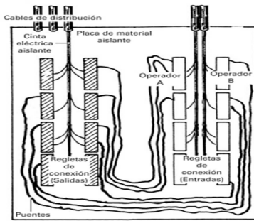
Figura 6 Distribución en Armario
