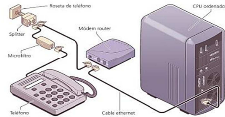
Figura 2 Conexión ADSL
