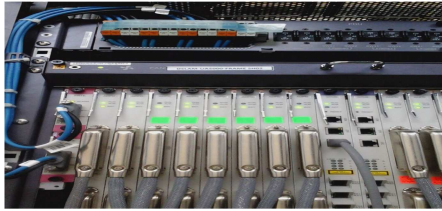
Figura 10 Dslam Huawei MA5600
