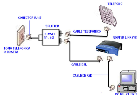
Figura 8 Diseño en el Interior del Abonado
