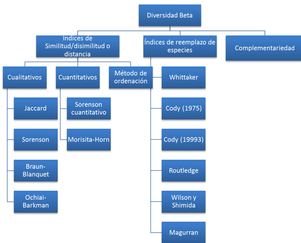
Figura7: Esquema de los Índices de Diversidad Beta. (Fuente: Hallfter & Moreno, 2001)
