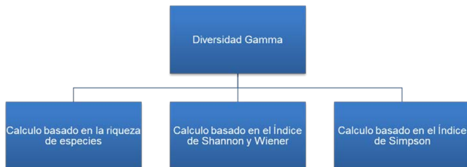
Figura8: Esquema de los Índices del Diversidad Gamma(Fuente: Hallfiter & Moreno,2001)
