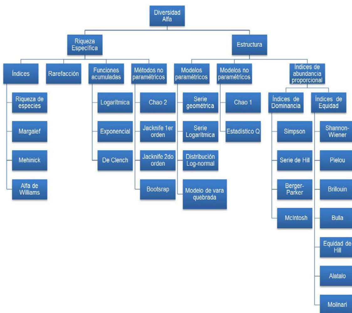
Figura6: Esquema de los Índices de Diversidad Alfa. (Fuente:Hallfiter & Moreno,2001)
