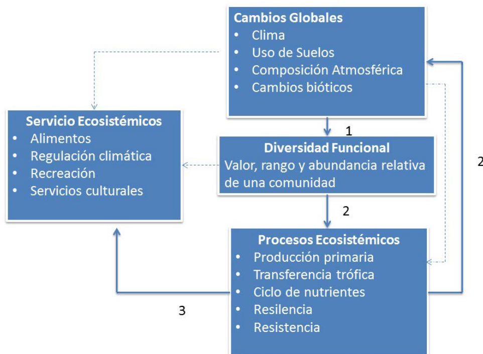
Figura 9: Diversidad Funcional en respuesta a los cambio globales y Servicios Ecosistémicos (Fuente: Díaz et al., 2007 b)
