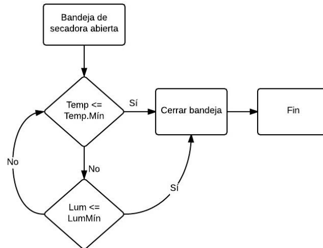
Figura 3.10 Diagrama de cerrado de bandeja en moda automático
