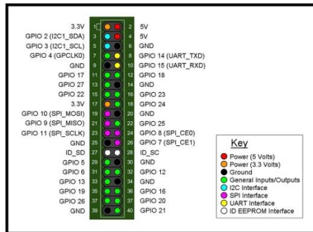
Figura 4.4 Diagrama de Pines GPIO de Raspberry Pi
