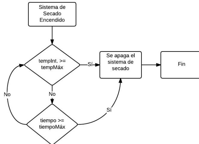
Figura 3.6 Diagrama de apagado de secadora en automático
