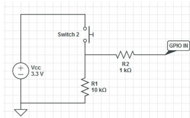
Figura 4.5 Diagrama de botoneras de control
