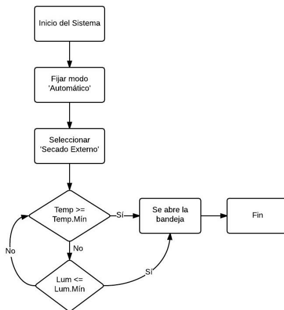
Figura 3.8 Diagrama de apertura de bandeja en modo automático
