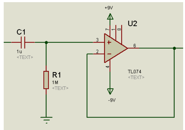
FIGURA 5. Filtro pasa-alto.
