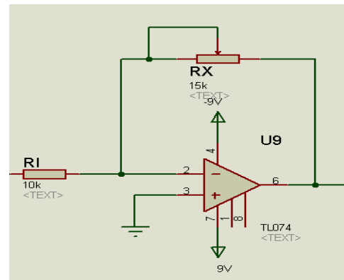
FIGURA 8. Amplificador inversor.
