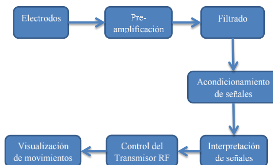
FIGURA 3. Diagrama de bloques del dispositivo EOG
