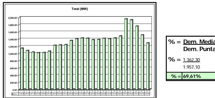
FIGURA 4.2: Demanda del bloque de demanda media
