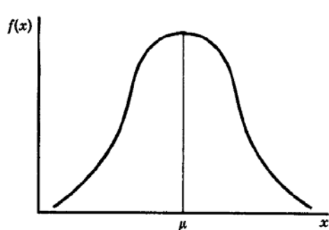
FIGURA 2.5: Distribucion normal
