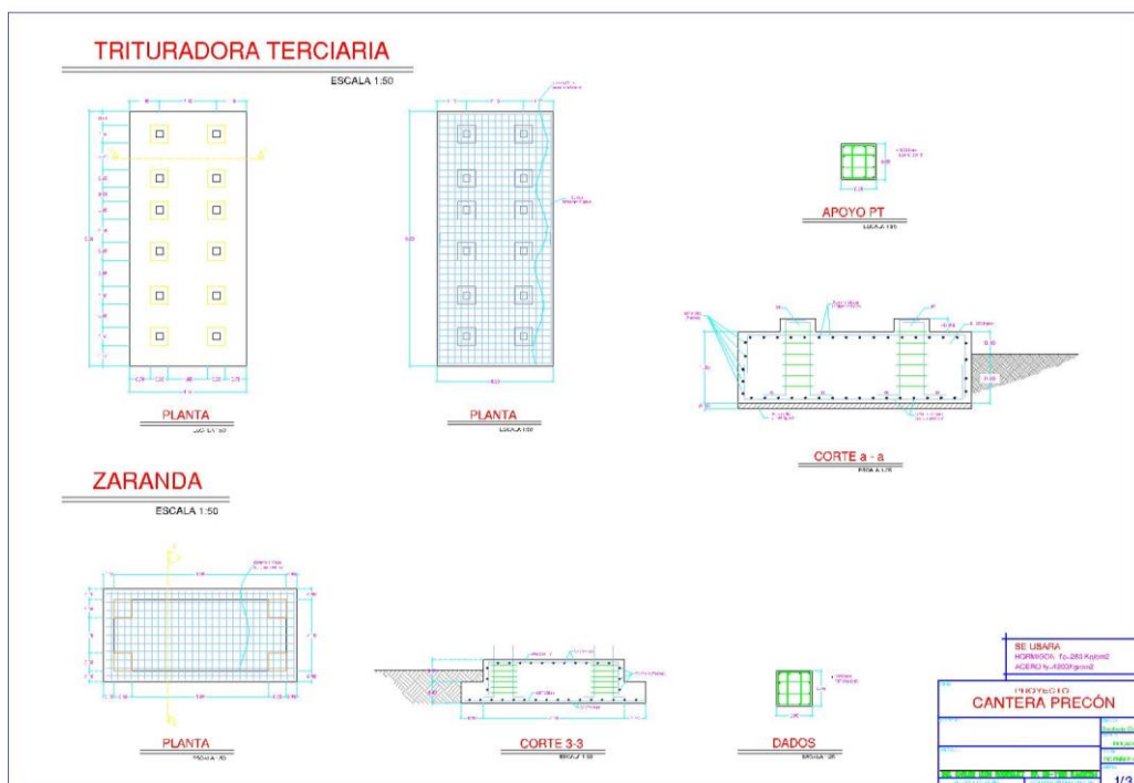
PLANO 3.4.- Plano de cimentación de la sección terciaria.
