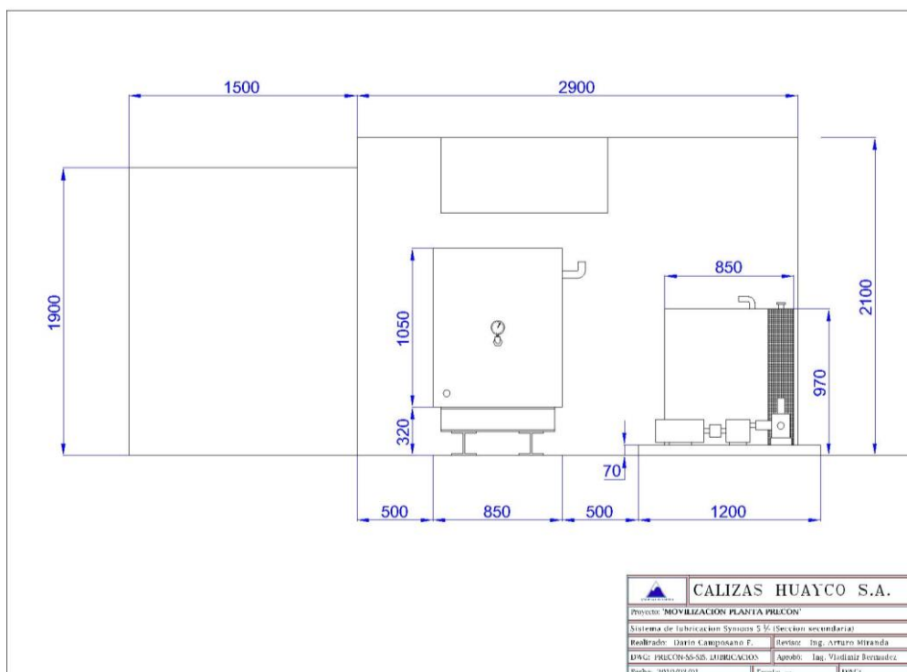
PLANO 3.10.- Vista frontal del diseño del sistema de enfriamiento del Cono 5 1/2.
