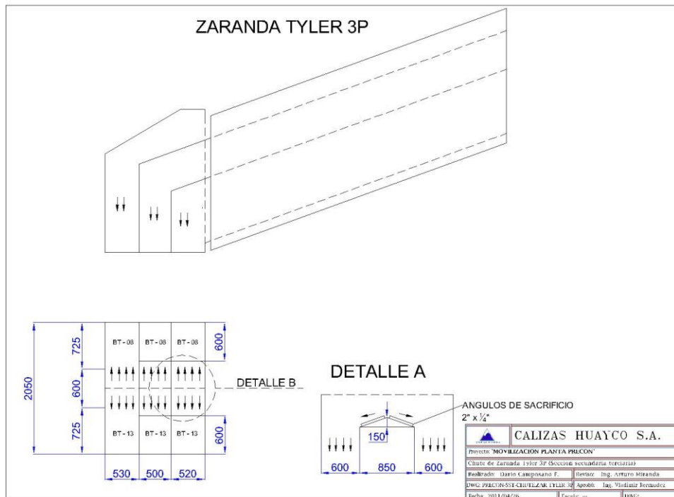
PLANO 3.7.- Chute de salida de zaranda Tyler 3P
