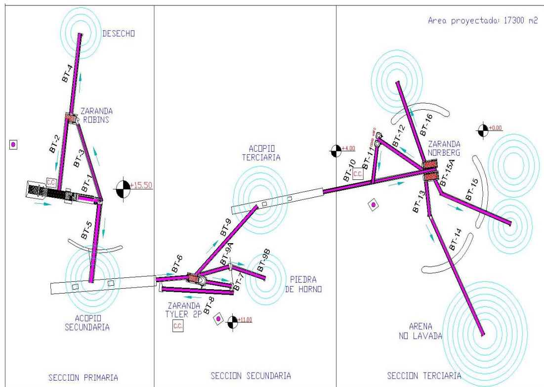
FIGURA 2.9.- Implantación de la Planta a trasladar.
