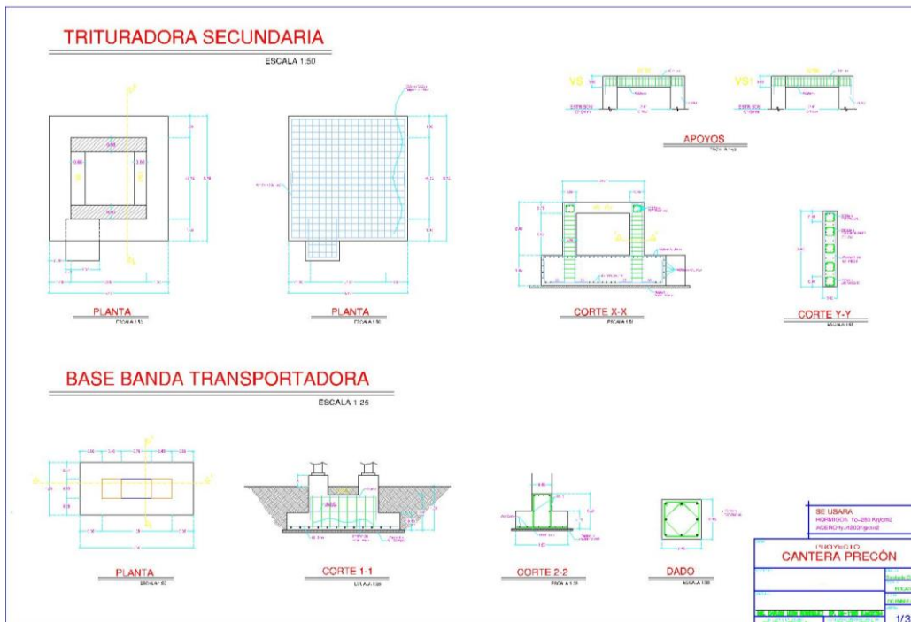
PLANO 3.2.- Plano de cimentación de la sección secundaria.
