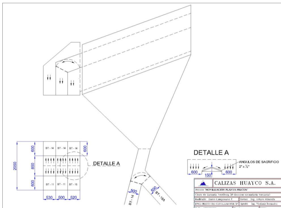
PLANO 3.8.- Chute de salida de zaranda Nordberg, para producto final.
