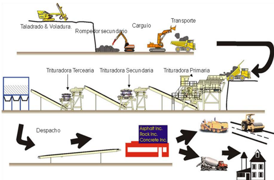
FIGURA 1.4.- Esquema de ciclo de desarrollo de la caliza desde el yacimiento hasta su uso. (Manual Metso)
