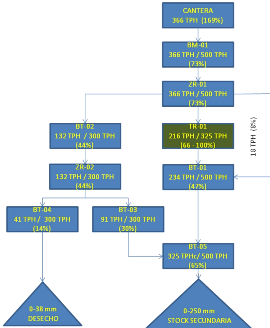
FIGURA 3.6.- Diagrama de cargas de la Sección Primaria de la Planta.
