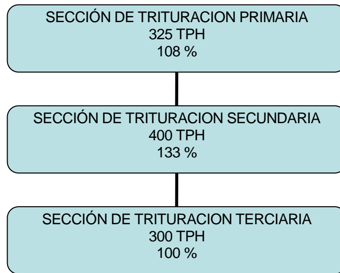
FIGURA 2.11.- Balance de cargas de la Planta a trasladar.
