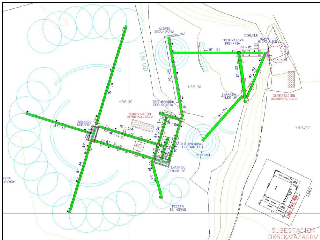
FIGURA 3.4.- Layout para el montaje de la Planta de Agregados.
