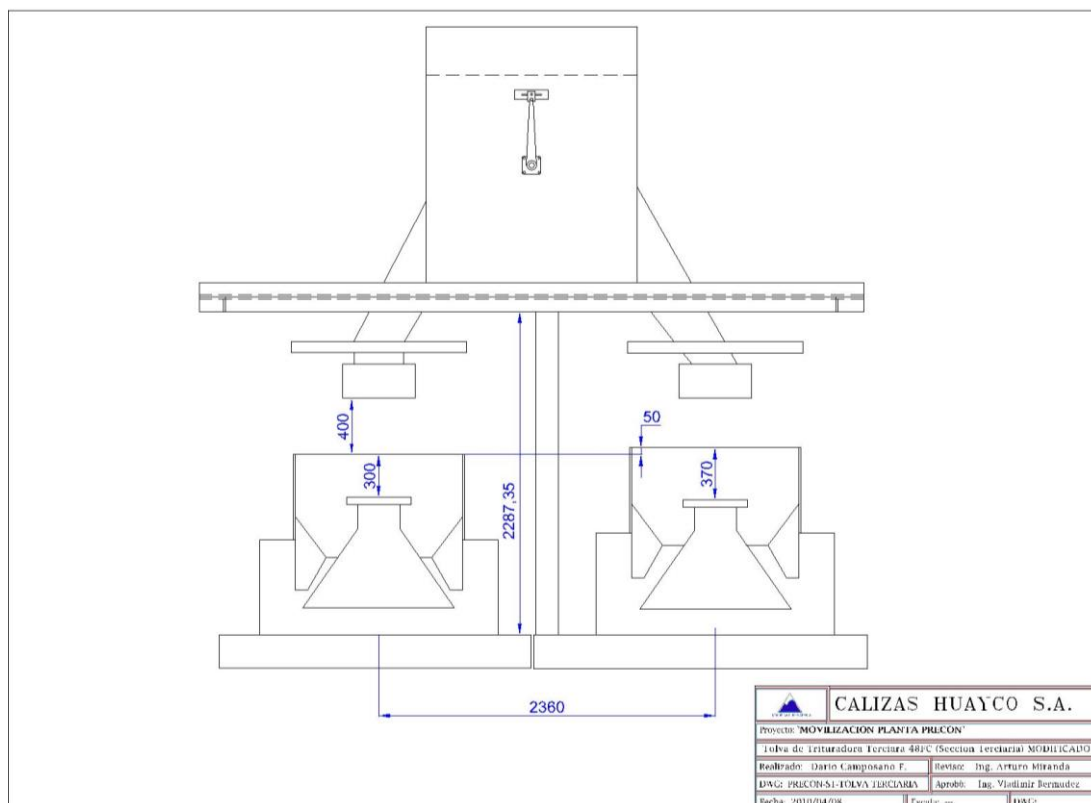
PLANO 3.12.- Vista frontal del nuevo diseño de chute de recepción de material para alimentar trituradoras terciarias 48FC.
