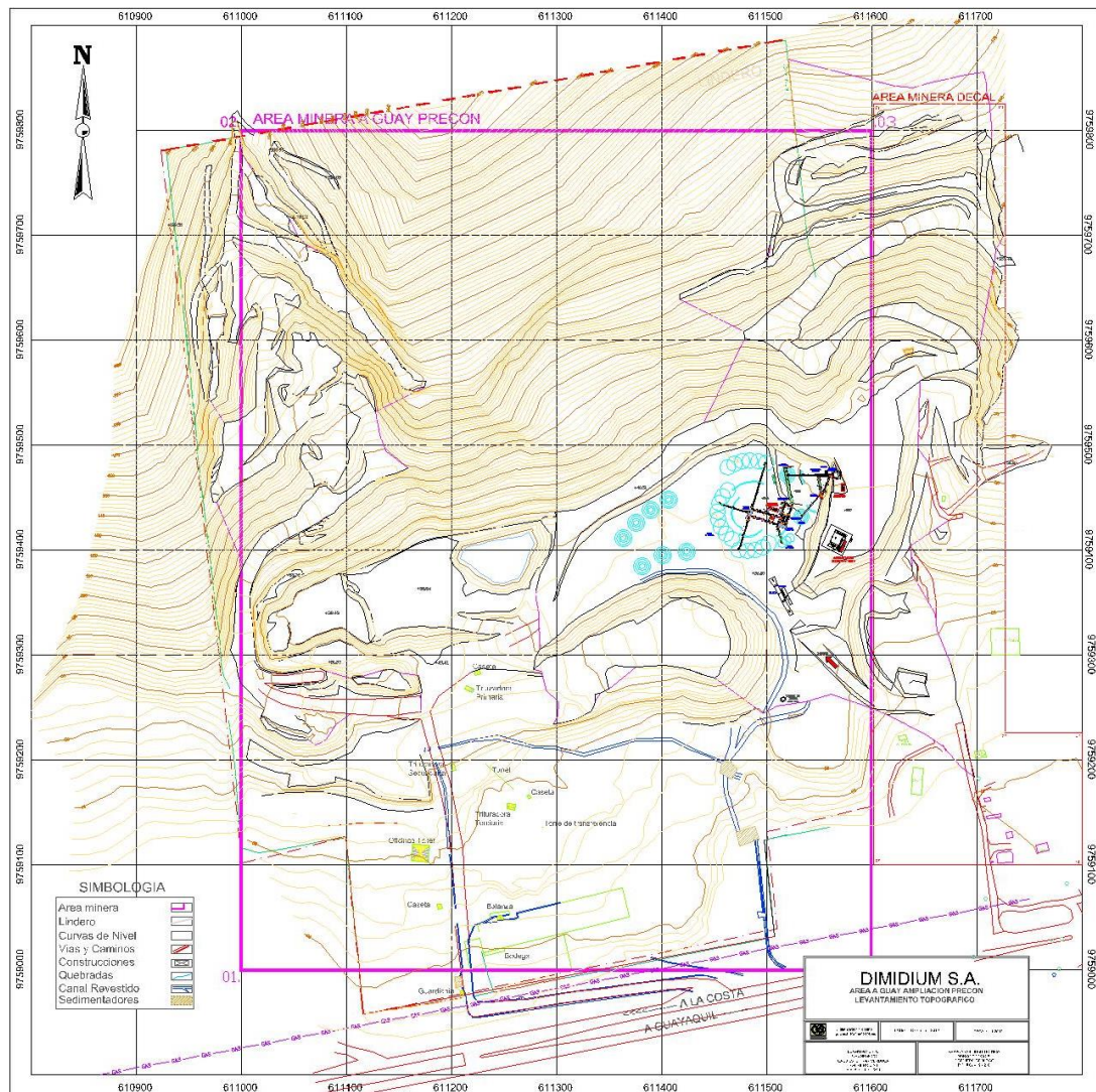
FIGURA 3.2.- Plano topográfico con implantación de Planta.
