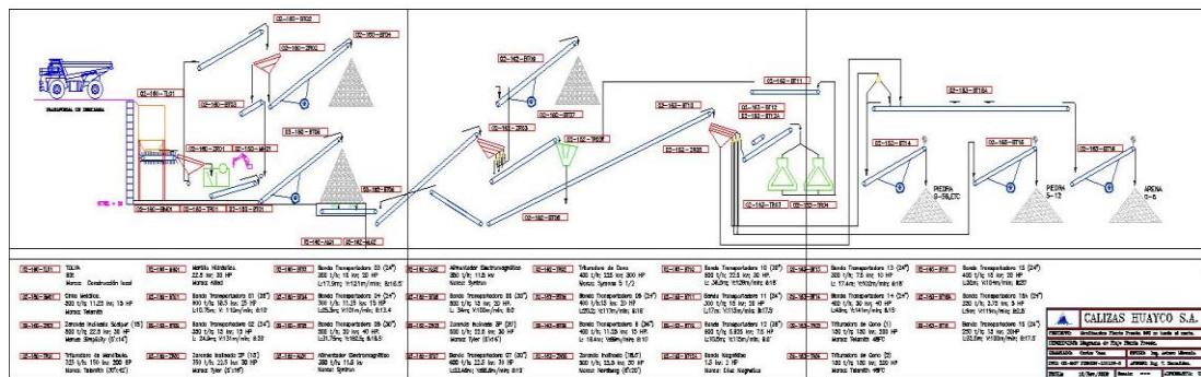
FIGURA 3.3.- Diagrama de flujo
