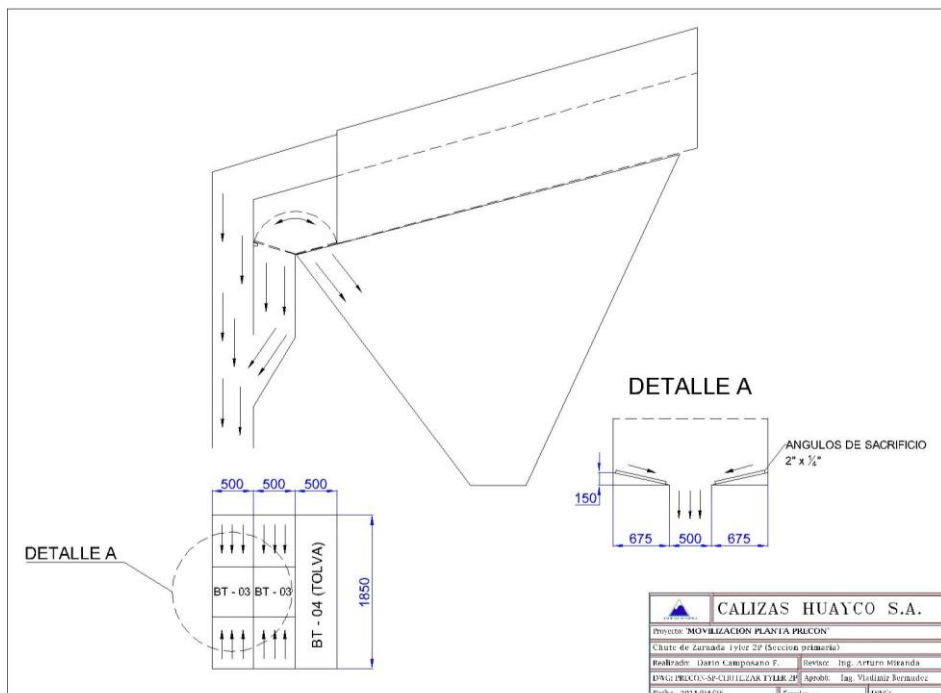
PLANO 3.5.- Chute de salida de la zaranda Tyler 2P
