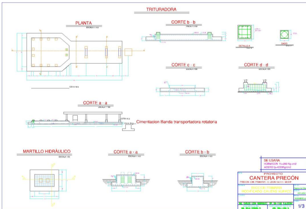
PLANO 3.1.- Plano de cimentación de la sección primaria.
