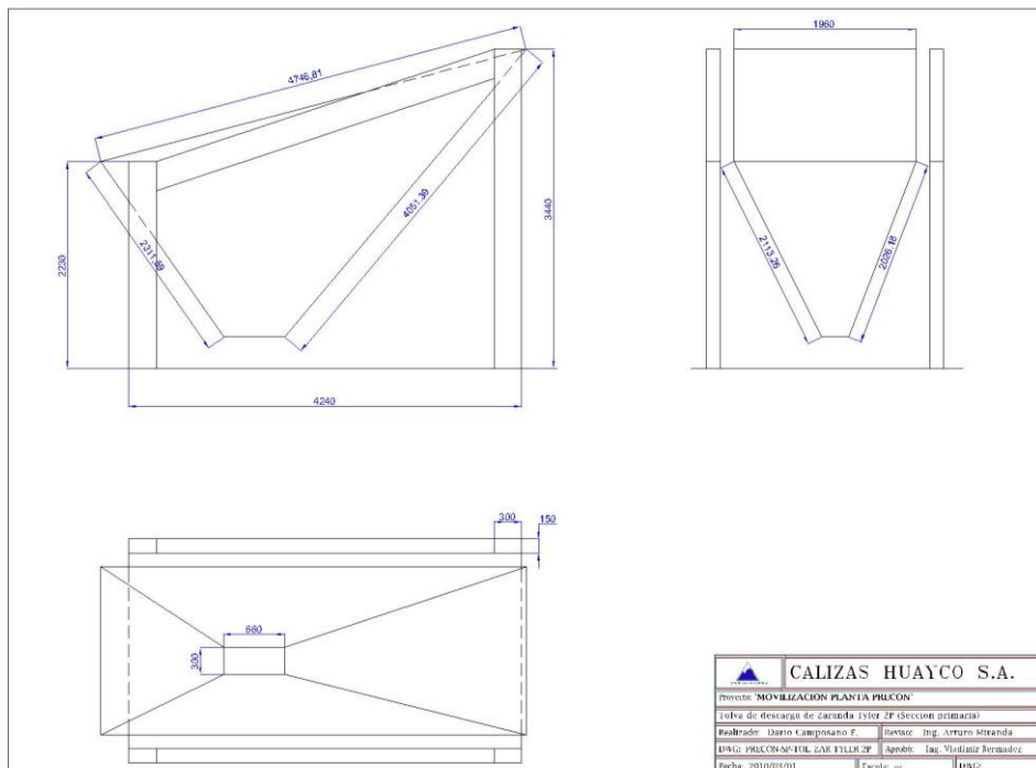
PLANO 3.6.- Tova de zaranda Tyler 2P.
