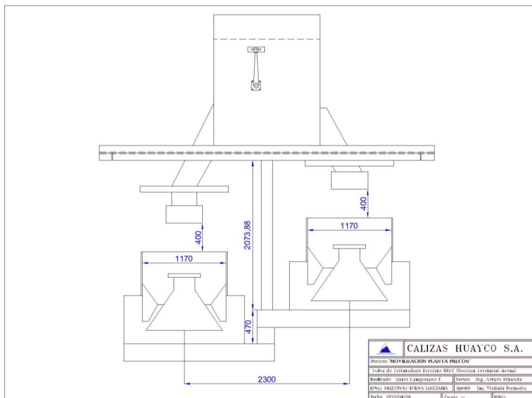
PLANO 3.11.- Vista frontal del chute de recepción de material para alimentar trituradoras terciarias 48FC.
