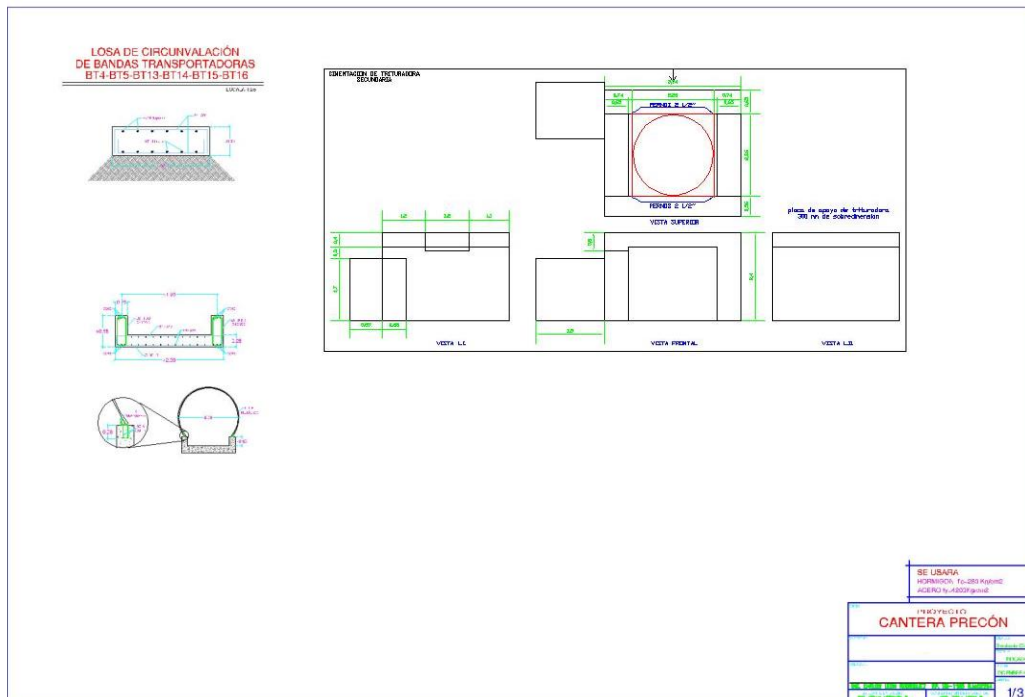
PLANO 3.3.- Plano de cimentación de túnel en la sección secundaria.
