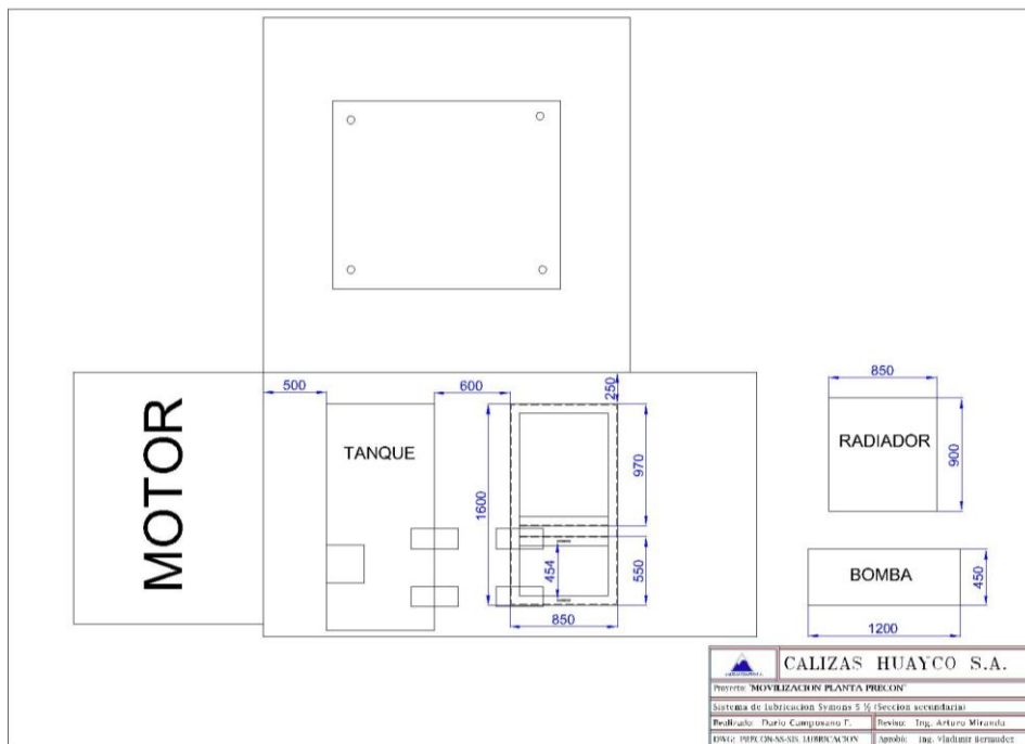
PLANO 3.9.- Vista superior del diseño del sistema de enfriamiento del Cono 5 1/2.
