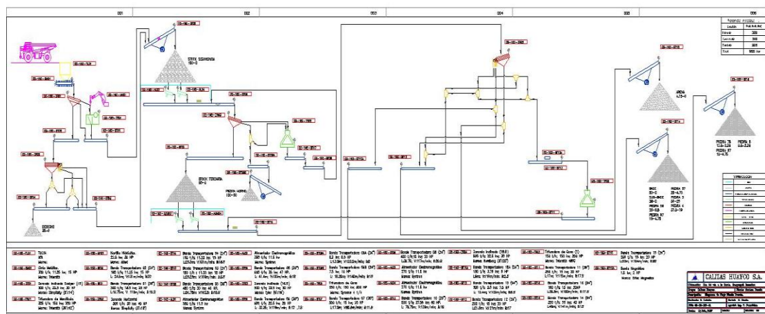
FIGURA 2.10.- Diagrama de Flujo de la Planta a trasladar.
