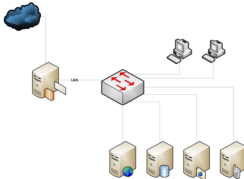
Figura 2.1 Topología de red actual
