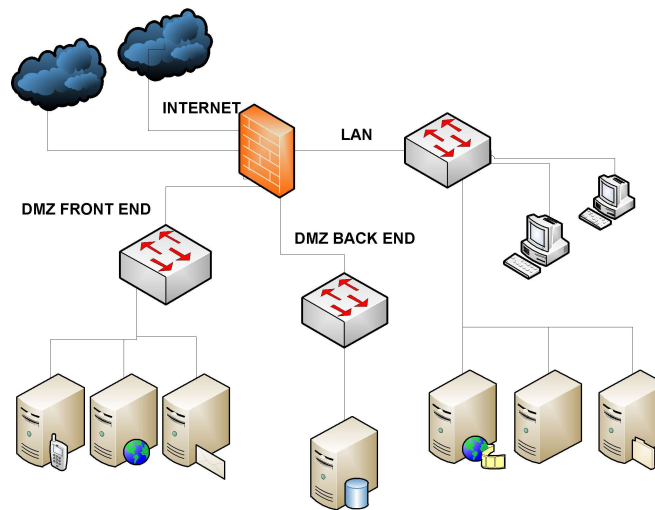
Figura 2.7 Topología de red final
