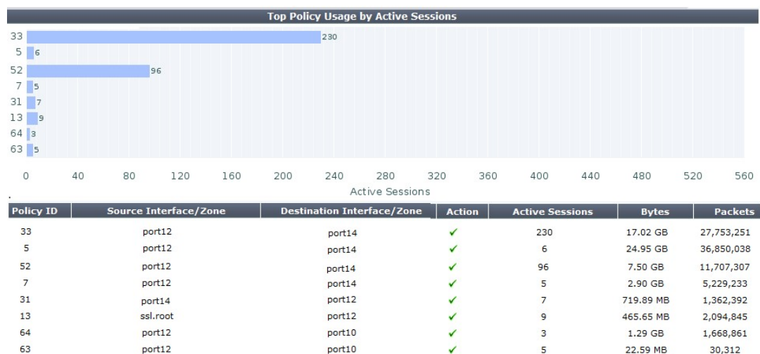
Figura 9.6 Monitoreo de interfaces WAN en failover
