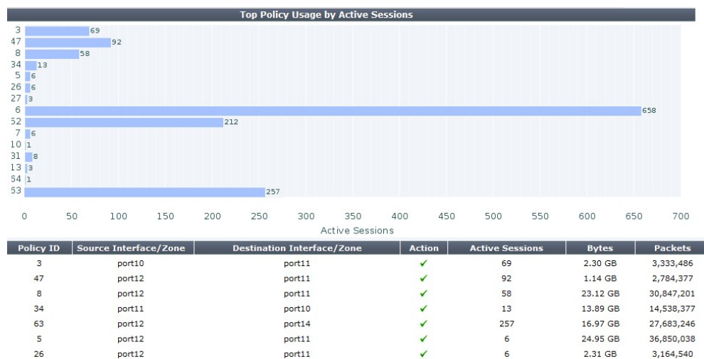
Figura 9.5 Monitoreo de uso de interfaces WAN
