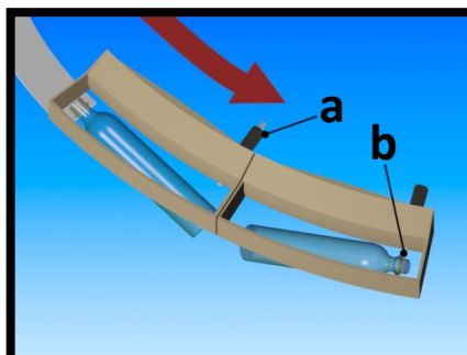
FIGURA 3.9 SISTEMA DE CAÍDA DE LAS BOTELLAS AL EMBUDO
