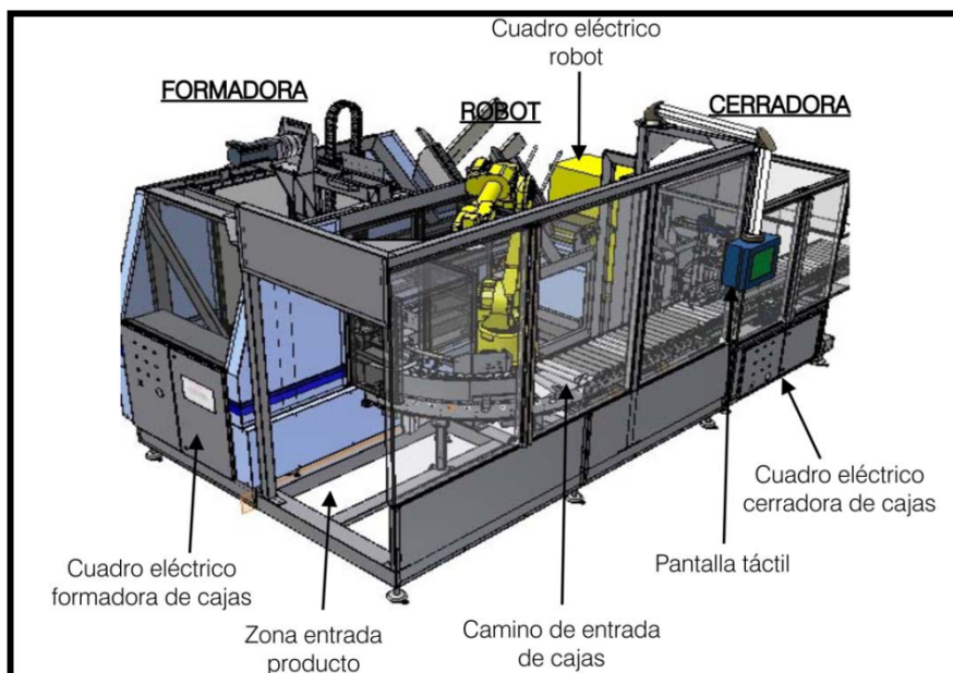
FIGURA 3.23 MULTIBOX
