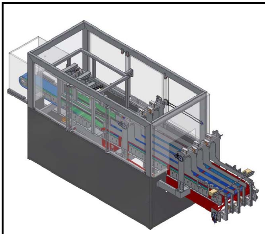
FIGURA 3.22 DISTRIBUIDOR
