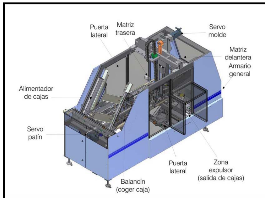
FIGURA 3.25 FORMADORA
