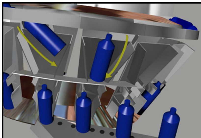
FIGURA 3.8 ZONA DE CAIDA A LOS EMBUDOS
