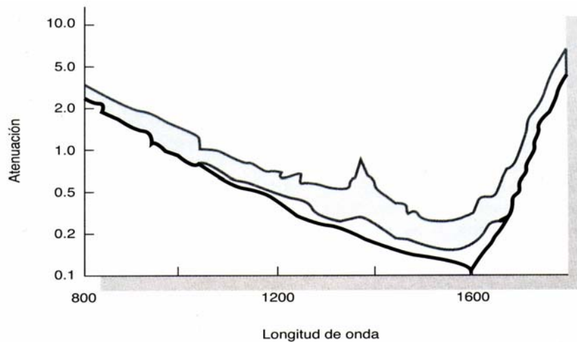
Figura 6.4 Atenuación en una fibra óptica en función de la longitud de onda
