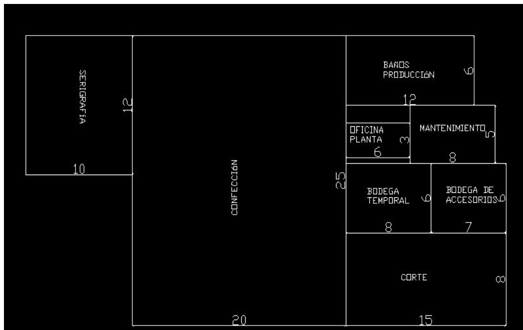
FIGURA 4.31: PLANO PRODUCCIÓN QAP
