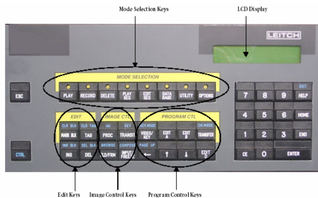
Fig. 4.64. Panel de Control
