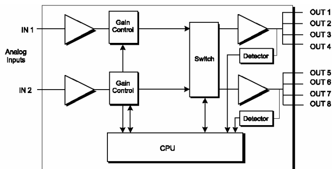
Fig. 4.83. Diagrama Esquemático del ADA – 3981
