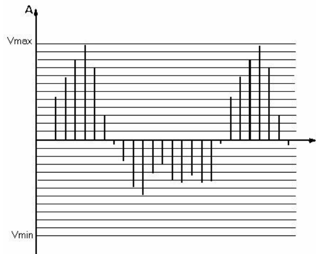
Fig. 1.14 Cuantificación de una señal muestreada
