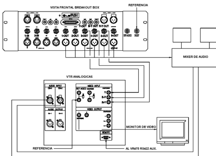
Fig. 4.37. Conexión entre Break – Out – Box y VTR (extracción video)
