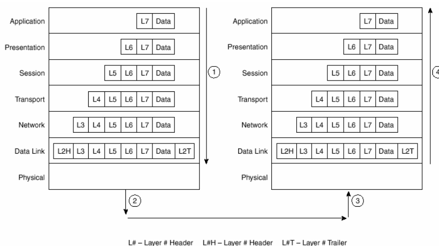
Fig. 2.5 Encapsulamiento de datos en comunicación entre 2 sistemas
