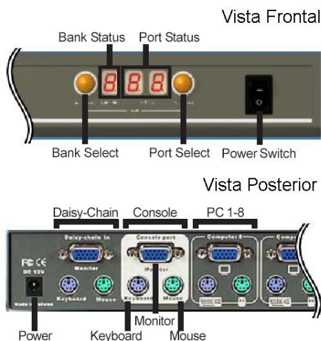
Fig. 4.120. Paneles del DKVM – 8E
