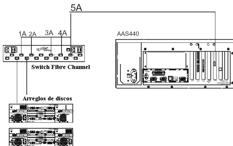
Fig. 4.24. Conexiones entre AAS – 440 y red Fibre Channel
