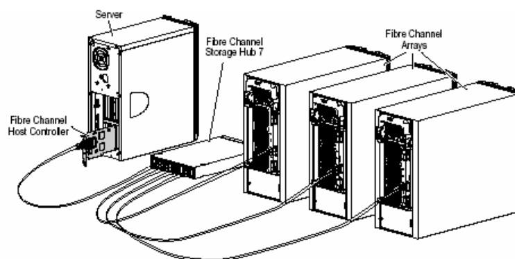
Fig. 2.20 Estructura típica de fibre channel
