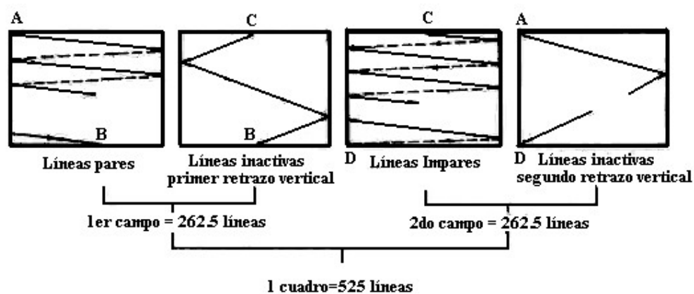
Fig. 1.6 Barrido Interlineado
