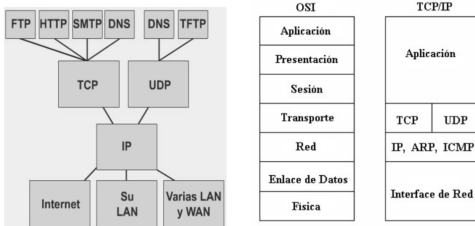
Fig. 2.8 a) Gráficos de protocolo TCP/IP
