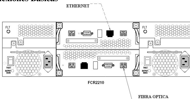
Fig. 4.11. Conexiones del FCR – 2180
