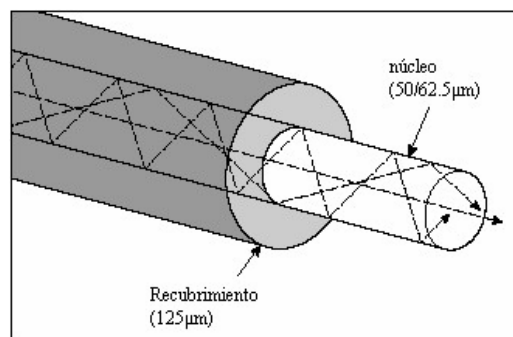
Fig. 2.13 Fibra óptica multimodo
