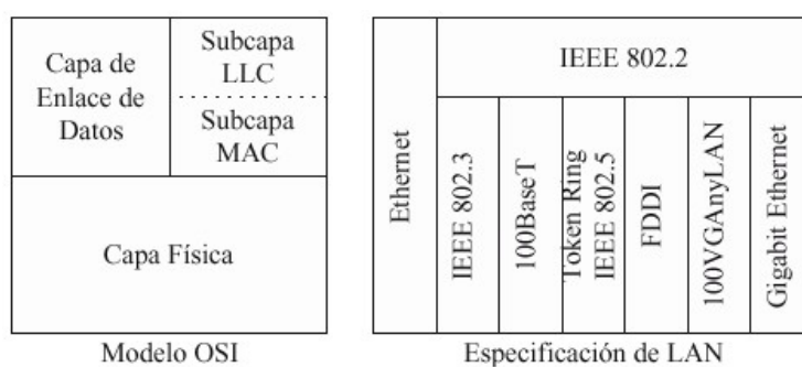
Fig. 2.11 Diferencia entre Ethernet y IEEE 802.3
