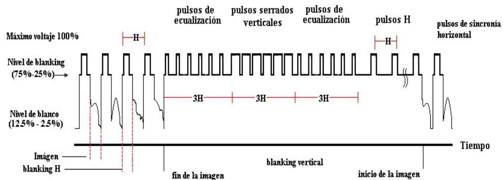
Fig. 1.12 Pulsos de sincronía y blanqueo vertical para sucesivos campos
