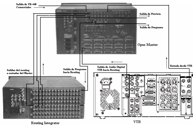
Fig. 4.88. Principales Conexiones del Opus Master
