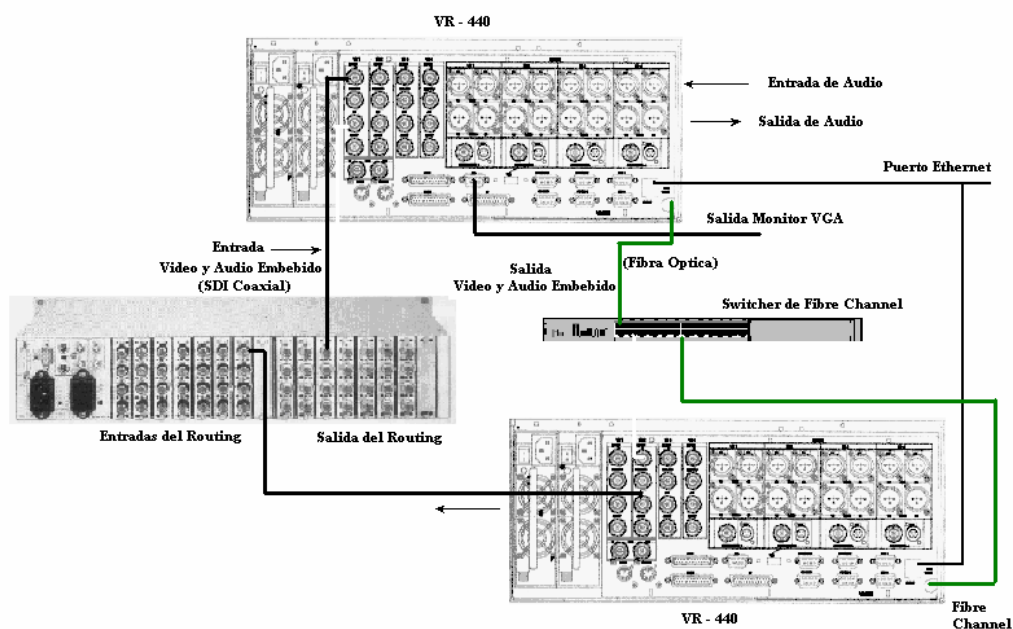
Fig. 4.3. Conexión del VR – 440
