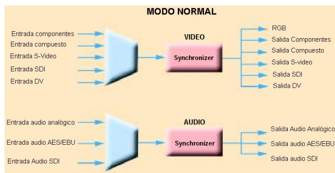
Fig. 4.59. Modo Normal del DPS – 575
