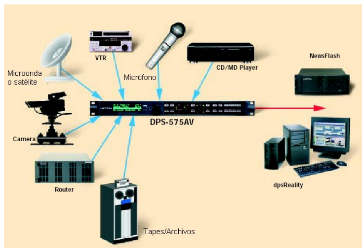
Fig. 4.61. Elementos a conectar con el DPS – 575
