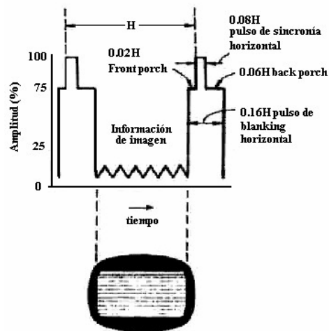
Fig. 1.11 Detalles del Blanking Horizontal y Pulsos de Sincronía
