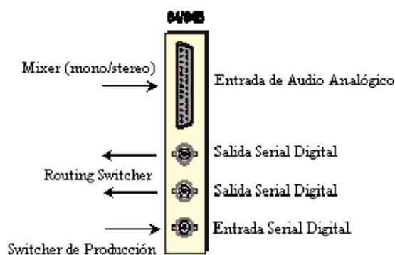
Fig. 4.79. Conexiones del MXA – 6001
