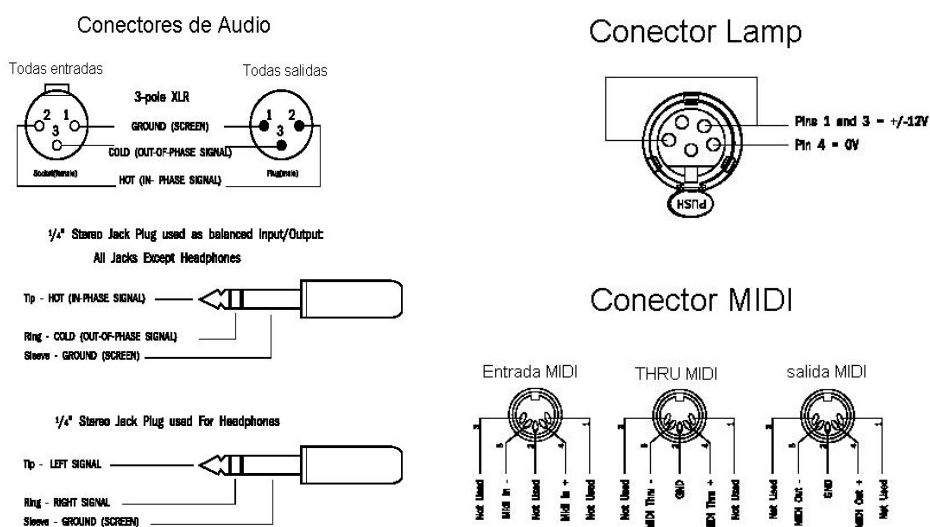
Fig. 4.96. Conectores de Consola Mixer Spirit
