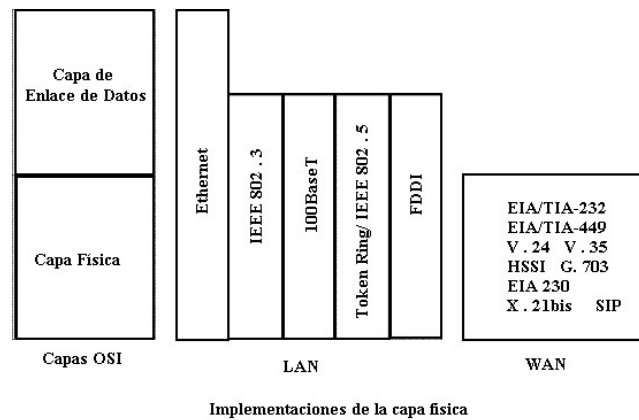
Fig. 2.4 Implementos de la capa fisica
