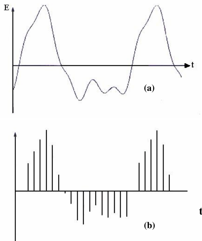
Fig. 1.13 a) Señal analógica b) Resultado del muestreo (PAM)
