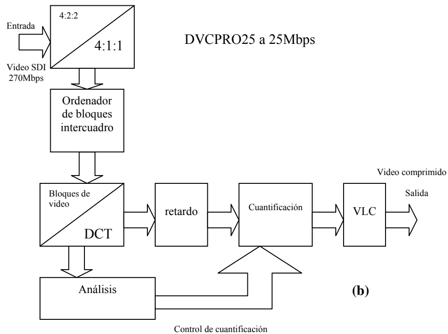
Fig. 1.24 Compresión basada en DV a) DVCPRO50 b) DVCPRO25
