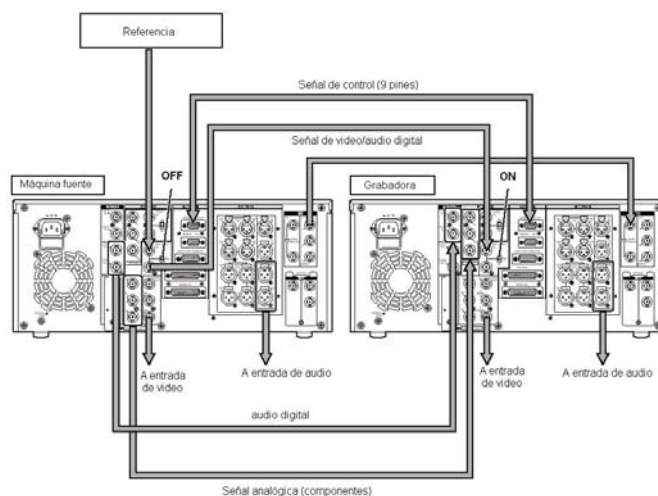
Fig. 4.114. Conexiones Principales de la VTR
