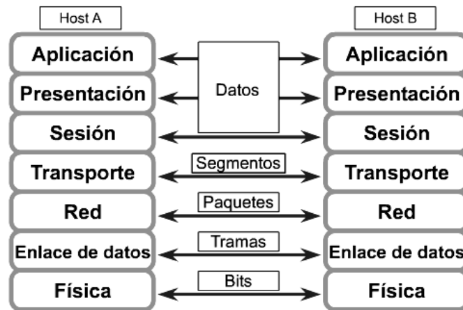
Fig. 2.6 Nombre de los datos en cada capa OSI
