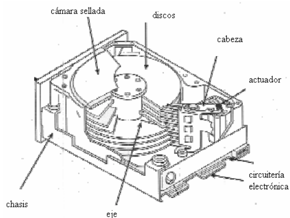
Fig. 3.1. Partes del disco duro
