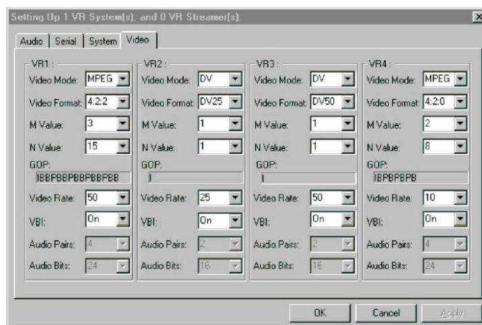
Fig. 4.4. Configuración Inicial del VR – 440
