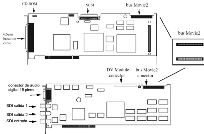
Fig. 4.49 Tarjeta de interfaces y tarjeta controladora SCSI de dps Reality
