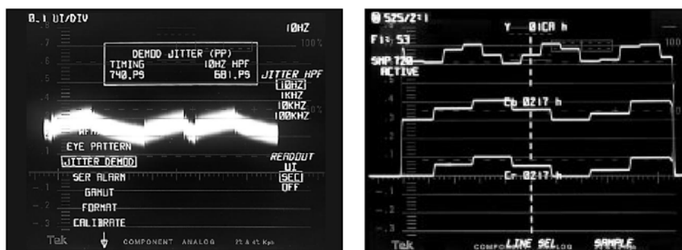
Fig. 4.108. Gráficas del WFM601M
