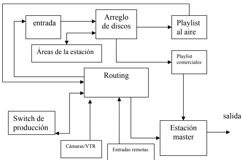
Fig. 4.1 Diagrama de bloques del canal de televisión
