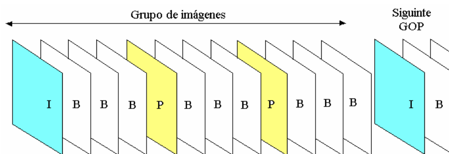
Fig. 1.22 Secuencia de fotogramas (típica) M – PEG2
