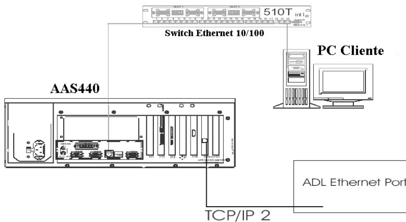
Fig. 4.23. Conexiones entre AAS – 440 y red Ethernet
