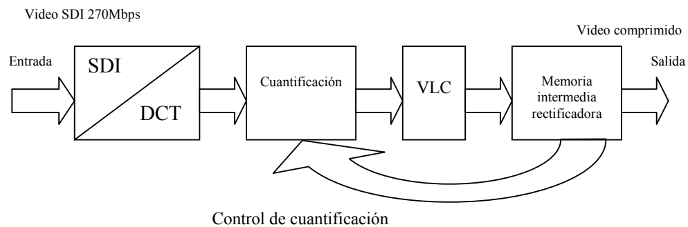
Fig. 1.20 Compresión basada en DCT – Tipo Feedback
