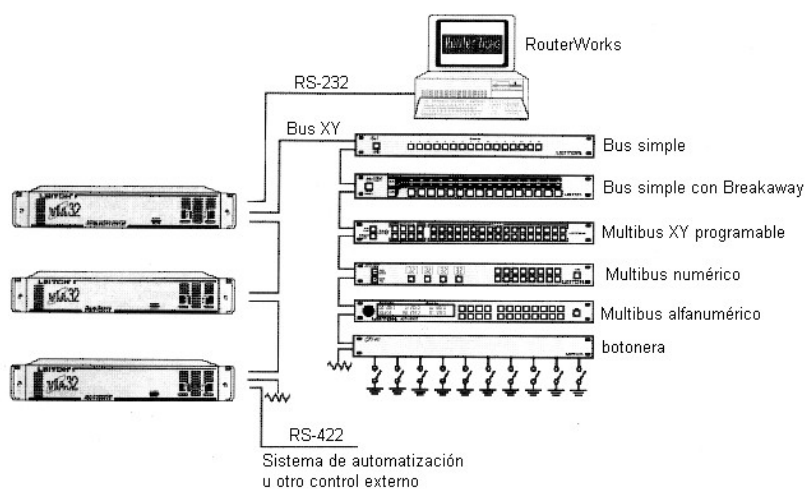
Fig. 4.53. Conexiones entre Routing Switcher
