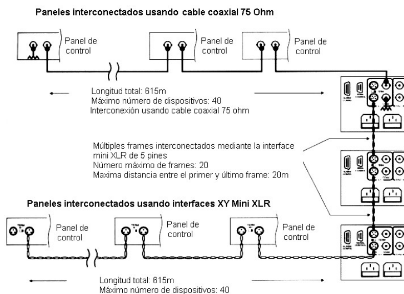
Fig. 4.56. Conexiones Seriales de Botoneras
