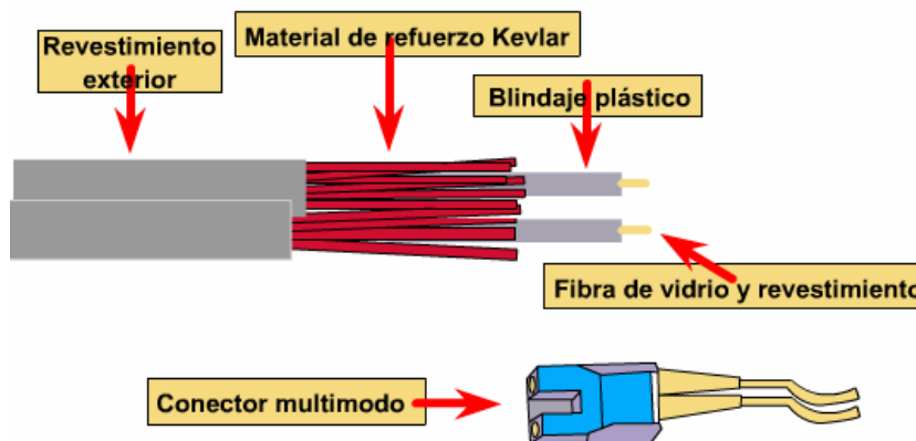
Fig. 6.3. Cable Fibra Óptica
