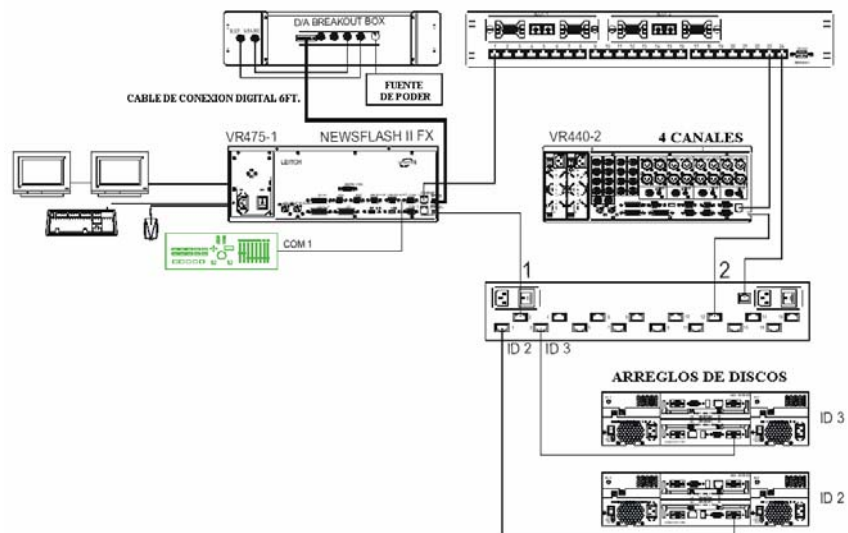
Fig. 4.36. Conexiones del VR - 475
