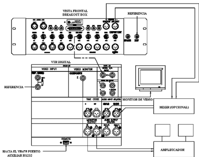
Fig. 4.38. Conexión entre Break – Out – Box y VTR (grabar video)
