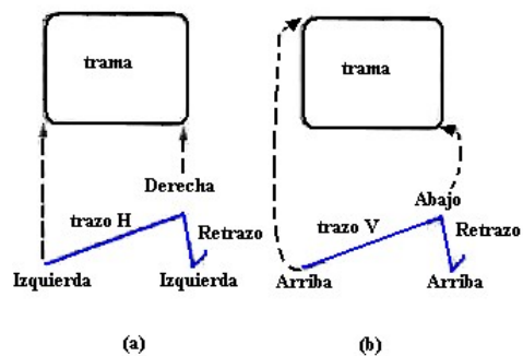
Fig. 1.5 Dirección del Trazo y Retraza en cada Barrido
