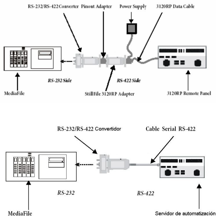
Fig. 4.67 Conexiones entre un Panel Remoto y el Still Store
