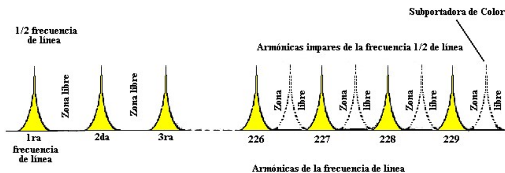
Fig. 1.8 Distribución de Energía dentro del espectro de frecuencias
