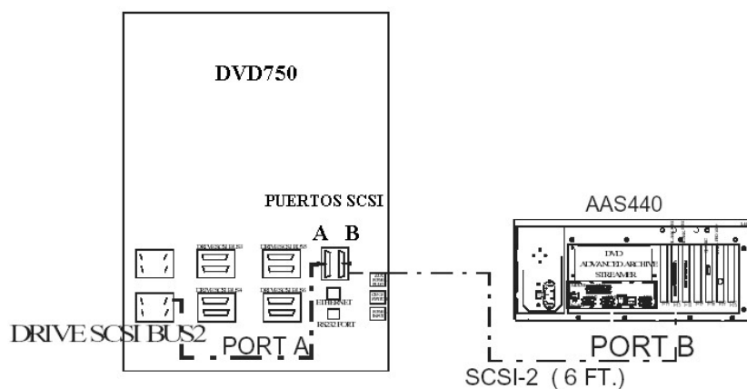
Fig. 4.22. Conexiones entre DVD y AAS – 440
