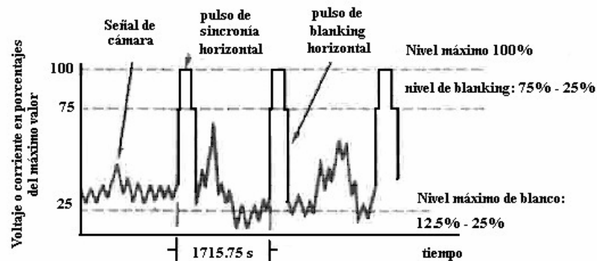
Fig. 1.10 Señal de Video Compuesto para 3 líneas horizontales consecutivas
