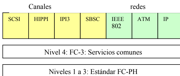
Fig. 2.17 Nivel 5 de fibre channel
