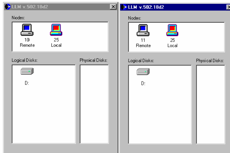
Fig. 4.16. LLM
