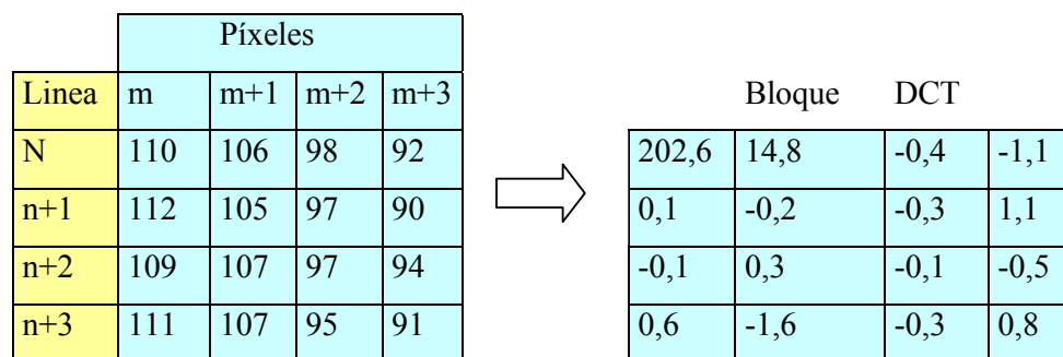
Fig. 1.17 Transformación DCT
