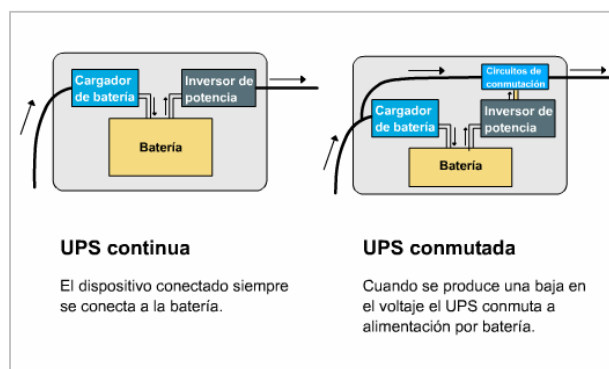
Fig. 6.8. Clases de UPS
