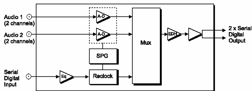
Fig. 4.78. Diagrama Esquemático del MXA – 6001
