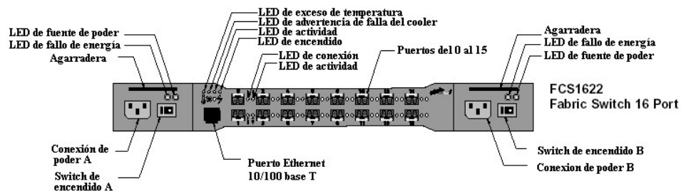
Fig. 4.8. Componentes del FCS - 1622
