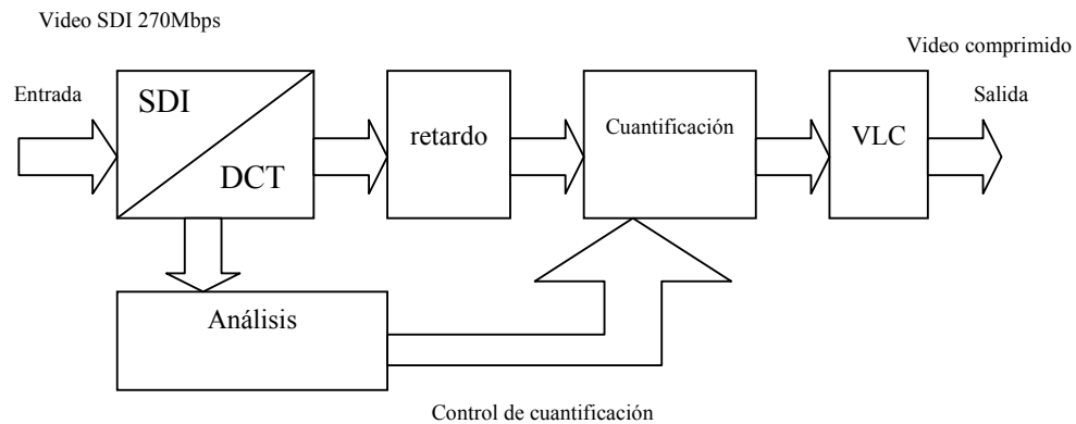
Fig. 1.23 Compresión basada en DCT – Tipo Feed Forward
