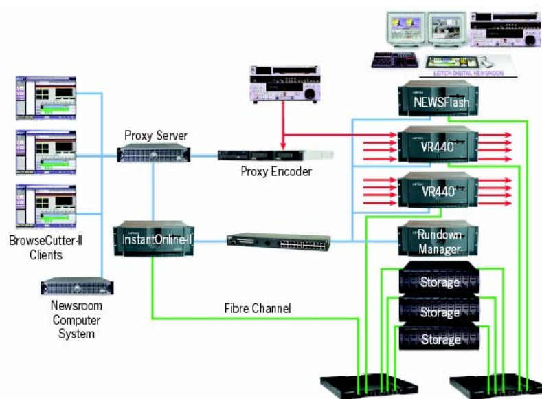
Fig. 4.44. Conexiones y Elementos del BrowseCutter II
