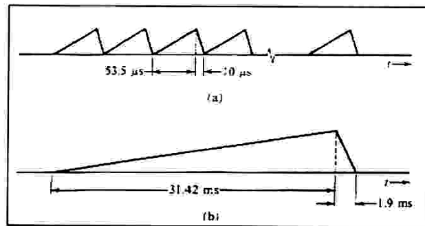
Fig. 1.3 a) Señal de deflexión horizontal b) Señal de deflexión vertical
