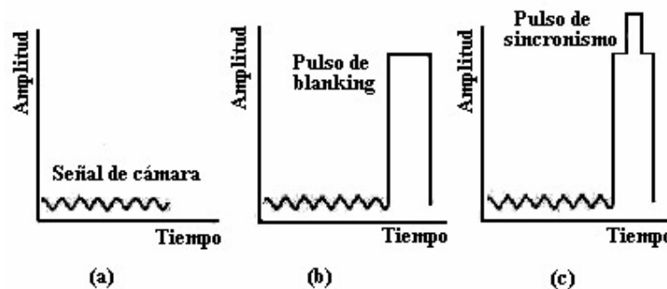
Fig. 1.9 Señal Compuesta
