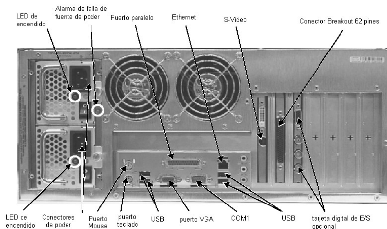
Fig. 4.66. Panel Posterior del Still Store
