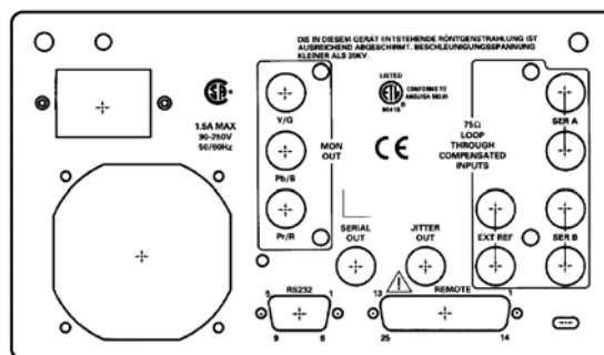
Fig. 4.109. Panel Posterior del WFM601M
