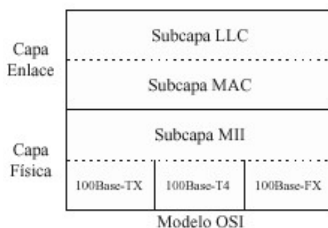
Fig. 2.12 Ubicación de la subcapa MII en el modelo OSI
