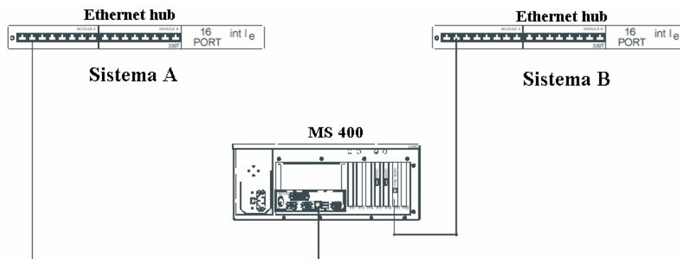
Fig. 4.14. Conexiones del MS – 400 con un Switch
