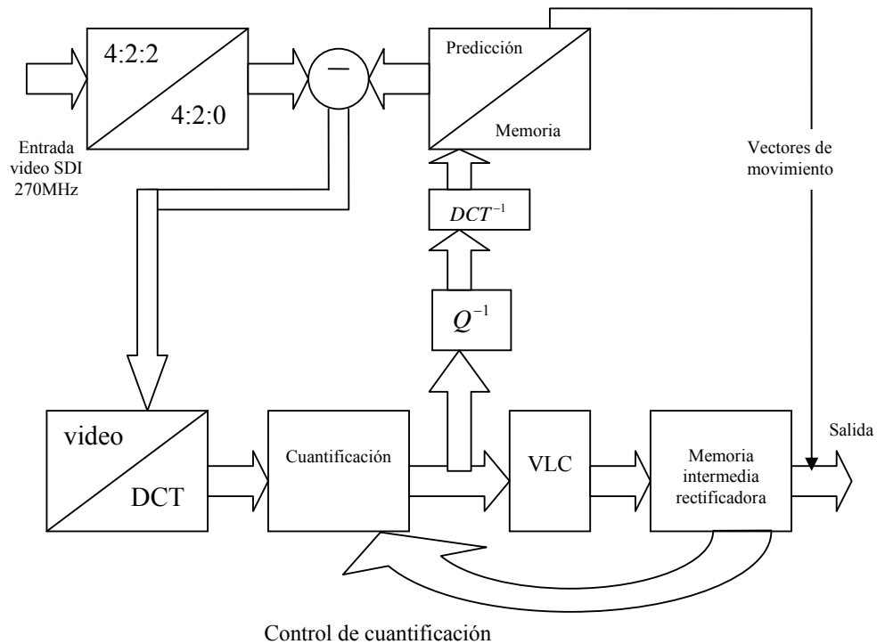
Fig. 1.21 Esquema de compresión M – PEG2 (simplificado)
