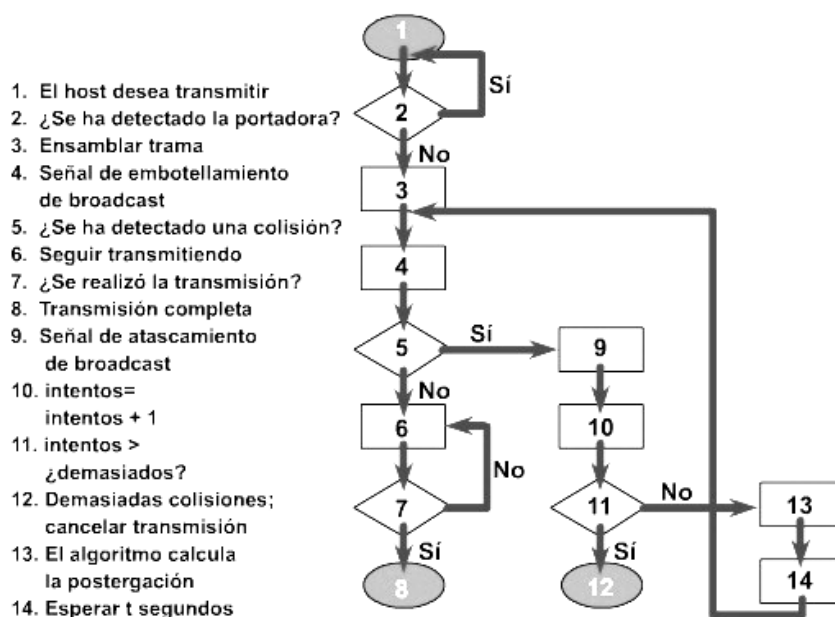
Fig. 2.10 Proceso CSMA/CD
