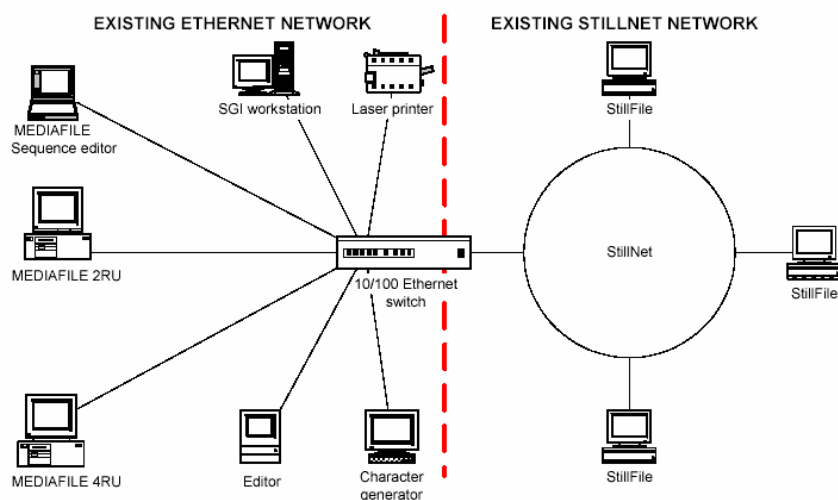
Fig. 4.62. Conexiones en Red del Still Store
