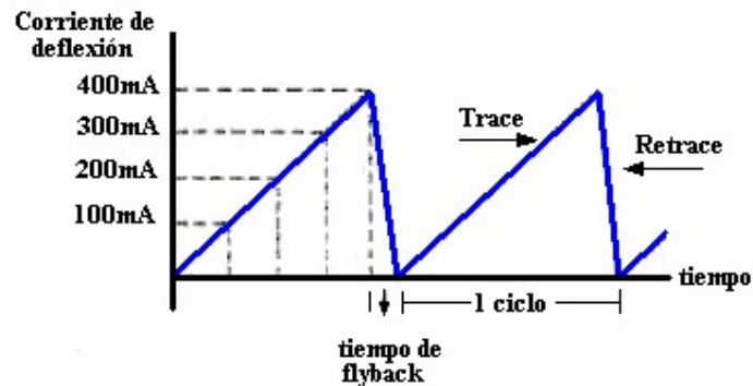
Fig. 1.4 Forma de Onda durante un Barrido
