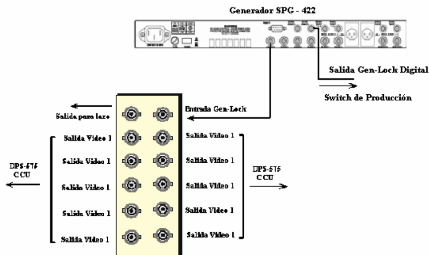
Fig. 4.106. Conexiones de Gen Lock
