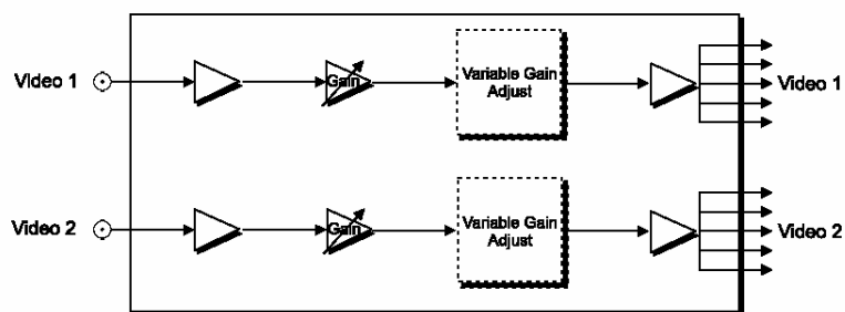
Fig. 4.82. Diagrama Esquemático del VDA – 6001
