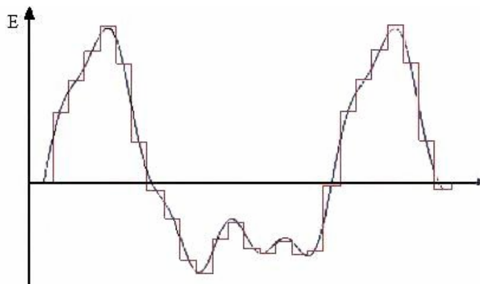
Fig. 1.15 Señal decodificada. Se observa el efecto diente de sierra
