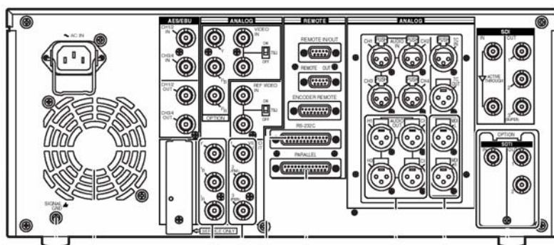
Fig. 4.115. Panel Posterior AJ – SD930
