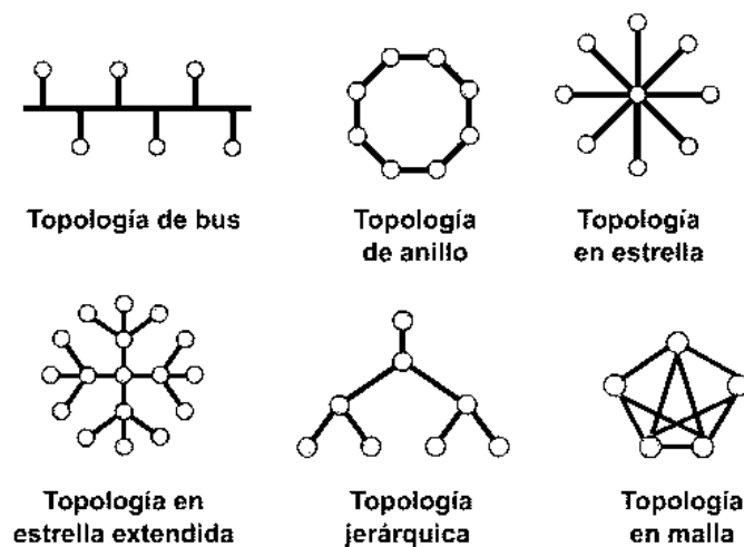
Fig. 2.9. Topologías Físicas
