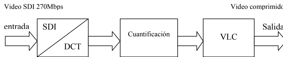
Fig. 1.19 Compresión basada en DCT – M – JPEG
