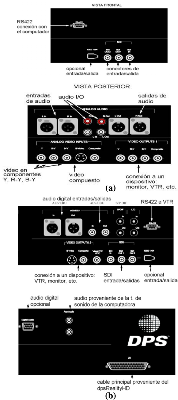
Fig. 4.50. Conexiones del Break – Out – Box a) Video b) Audio
