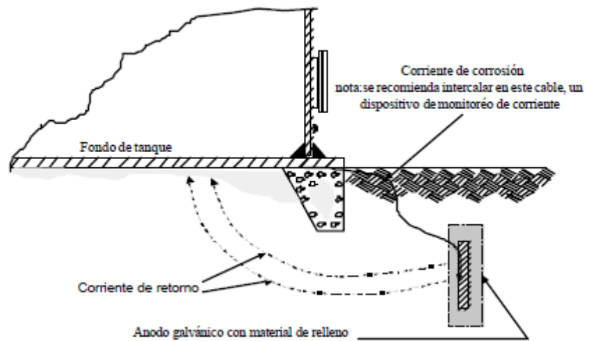
FIGURA 3.30 PROTECCION CATODICA CON ANODOS DE SACRIFICIO
