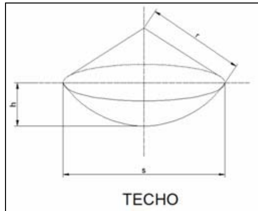
FIGURA 3.7 SEGMENTO CIRCULAR
