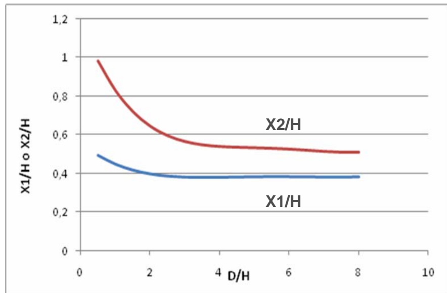
FIGURA 3.3 CENTROIDE DE LA FUERZA SÍSMICA
