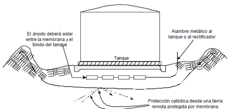
FIGURA 2.1 MEMBRANA IMPERMEABLE DEBAJO DE TANQUE DE ALMACENAMIENTO
