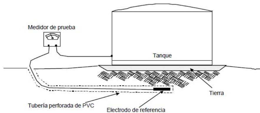
FIGURA 3.34 TUBERIA PERFORADA PARA EL ELECTRODO DE REFERENCIA
