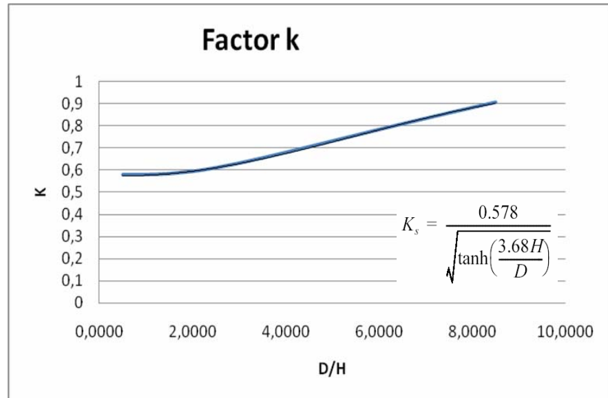
FIGURA 3.6 VALOR DEL FACTOR K
