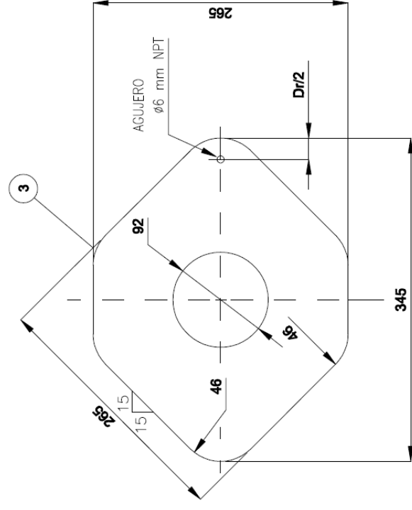
PLACA DE REFUERZO
