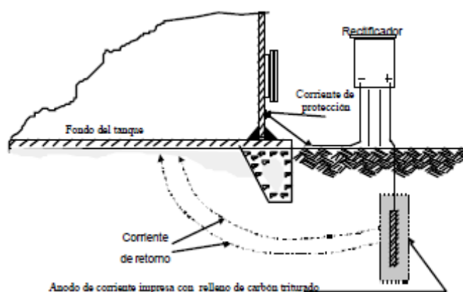
FIGURA 3.31 PROTECCION CATODICA CON CORRIENTE IMPRESA
