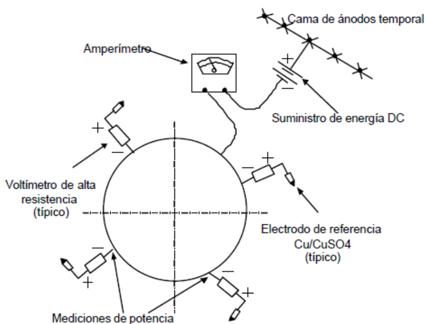
FIGURA 3.32 CONFIGURACION PARA UNA PRUEBA DE REQUERIMIENTO DE CORRIENTE
