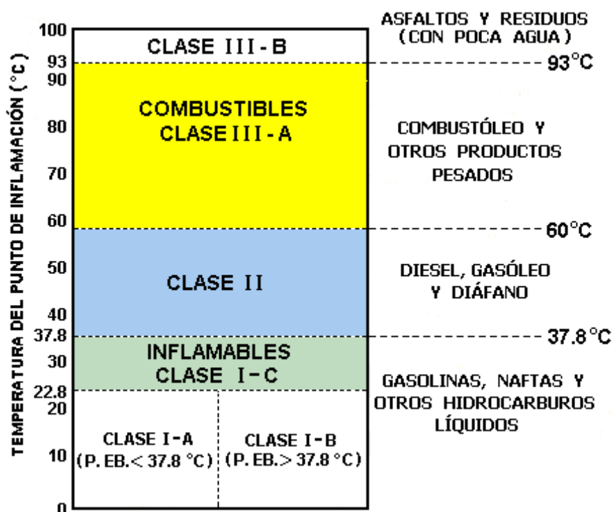
FIGURA 2.2 CLASIFICACION LIQUIDOS
