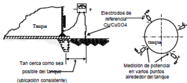
FIGURA 3.33 ESQUEMA DE MEDICION DE POTENCIAL
