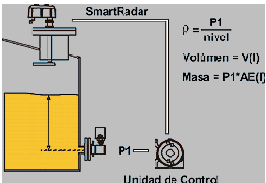
FIGURA 3.29 SISTEMA INTERCONECTADO DE RADAR
