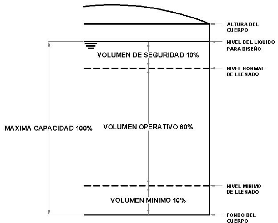
FIGURA 1.1 NIVELES Y VOLUMENES DE TANQUE DE ALMACENAMIENTO.
