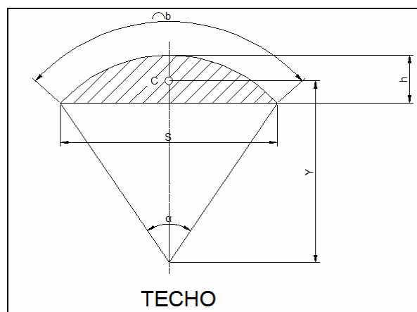
FIGURA 3.5 CENTROIDE DE UN SEGMENTO DE CIRCULO
