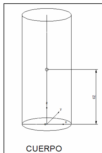
FIGURA 3.4 CENTROIDE DE CILINDRO
