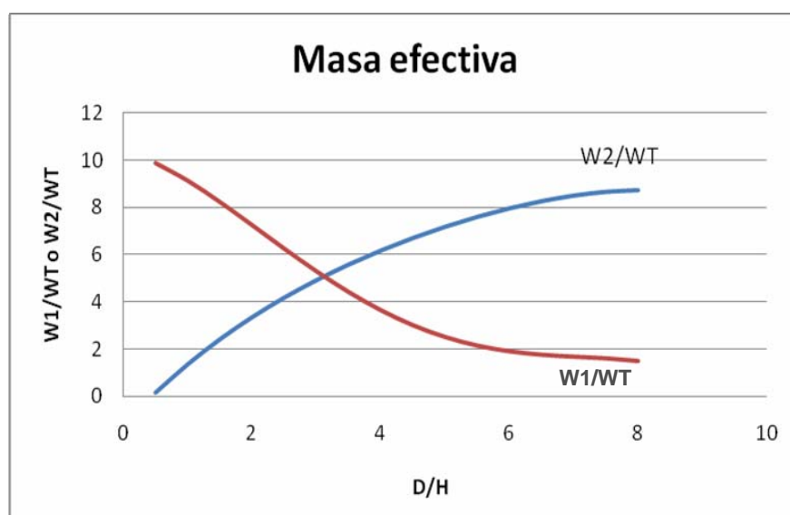
FIGURA 3.2 MASA EFECTIVA
