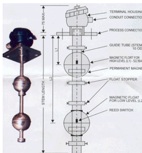
FIGURA 3.26 INTERRUPTOR DE NIVEL
