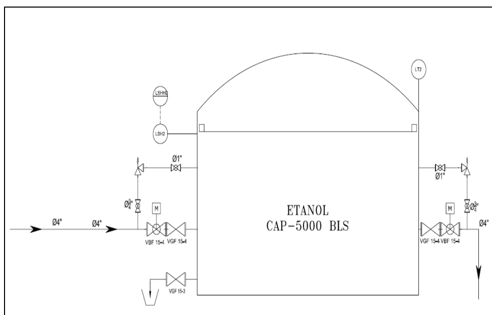
FIGURA 3.1 DIAGRAMA DE FLUJO DE TANQUE DE ALMACENAMIENTO
