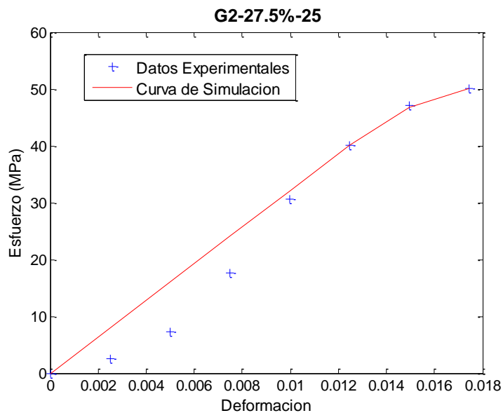
FIGURA 4.27. CURVAS ESFUERZO VS DEFORMACIÓN CON 27.5% DE ZEOLITA A 25 DÍAS DE CURADO
