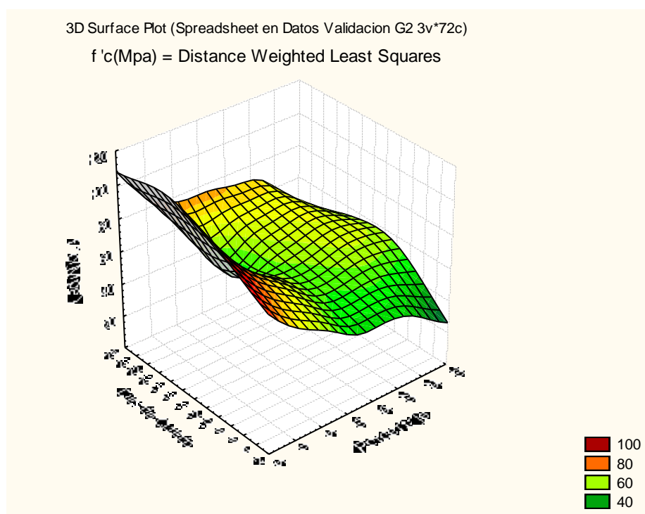
FIGURA 4.10. GRÁFICO DEL ESFUERZO ÚLTIMO VS. DÍAS DE CURADO Y PORCENTAJE DE ZEOLITA PARA DATOS DE VALIDACIÓN.
