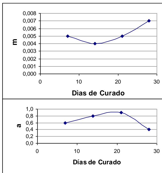
FIGURA 4.11. CURVAS DE a Y m A DIFERENTES DÍAS DE CURADO CON 25% DE ZEOLITA
