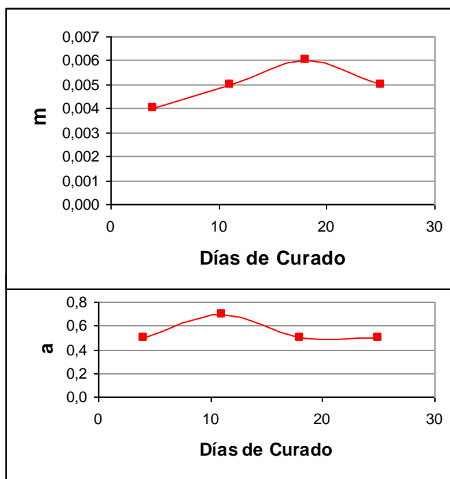
FIGURA 4.23. CURVAS DE a Y m A DIFERENTES DÍAS DE CURADO CON 27.5% DE ZEOLITA
