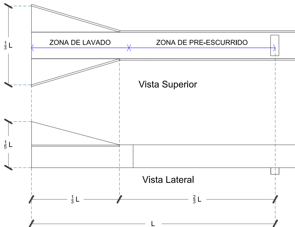
FIGURA 2.1. CARACTERÍSTICAS DE FORMA DEL EQUIPO DE LAVADO
