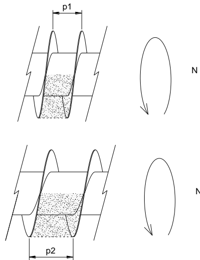
FIGURA 2.4. EFECTO DEL PASO HELICOIDAL EN EL LAVADO
