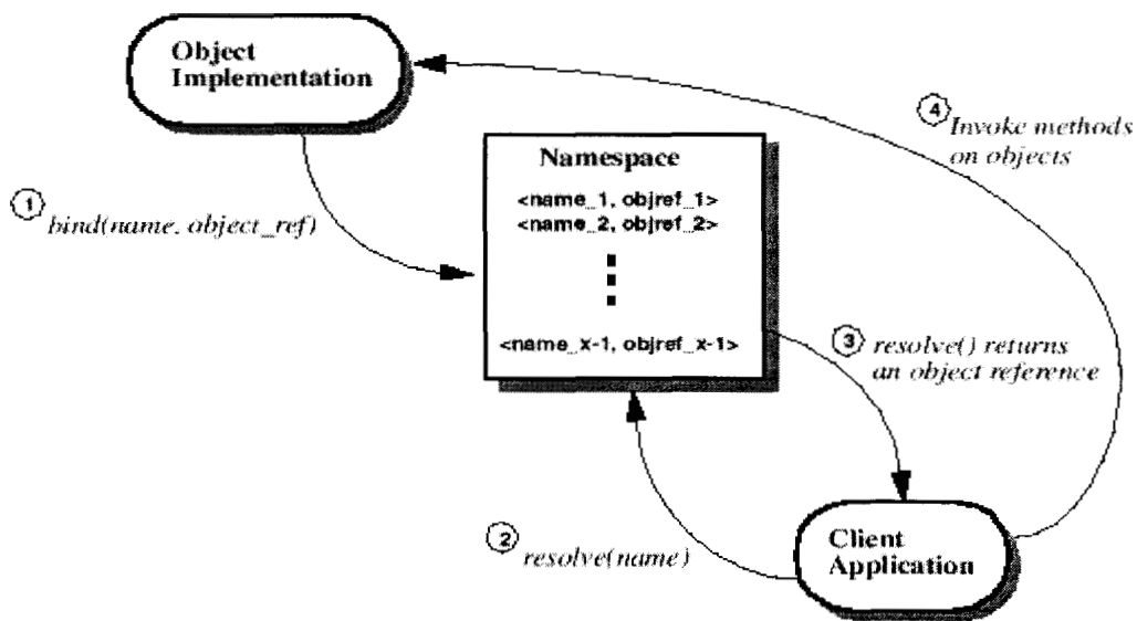
Figura 5: Enlazando, resolver y usar nombre de objetos para un nombre de contexto
