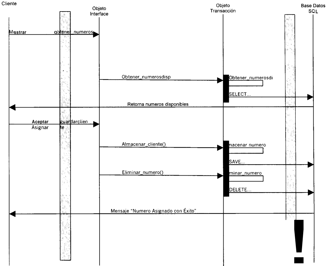
Figura : Asignacion de Numeros Exitosa
