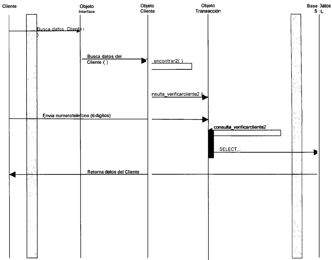
Figura : Verificación de Numeros Exitosa
