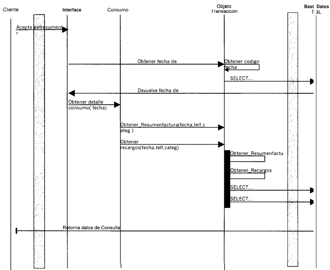
Figura : Consulta Exitosa
