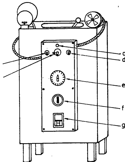
Fig. No 2.7 VISTA FRONTAL DEL PANEL DE CONTROLES
