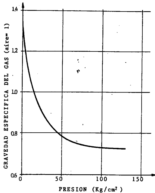
Fig. N° 1.6 VARIACION DE LA GRAVEDAD ESPECIFICA DEL GAS VS PRESION.
