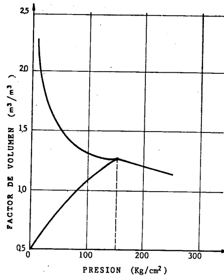
Fig. N° 1.3 VARIACIÓN DEL FACTOR DE VOLUMEN TOTAL DEL PETRÓLEO VS PRESIÓN.
