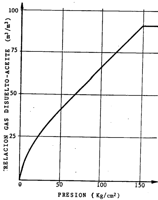
Fig. N° 1.5 VARIACION DE LA RELACION GAS DISUELTO VS. PRESION.
