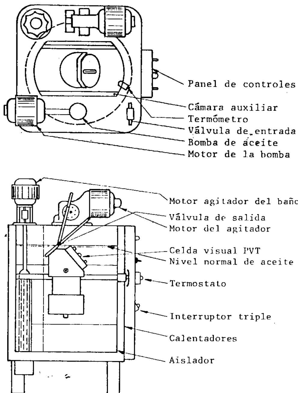
Fig. No 2.2 PARTES Y COMPONENTES DE LA CELDA PVT
