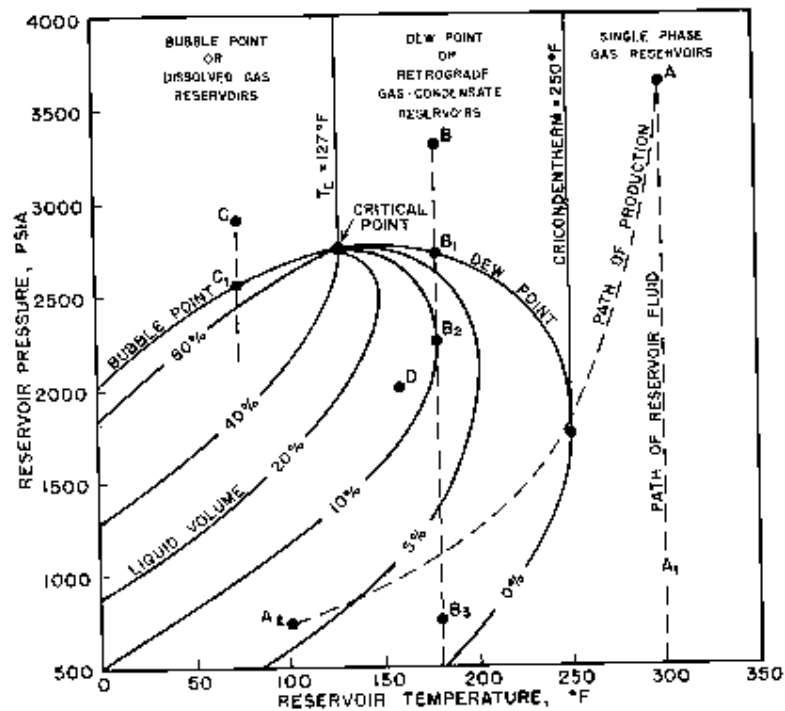
Fig. 1.1 DIAGRAMA DE FASES
