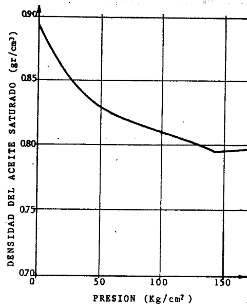
Fig. N° 1.7 VARIACION DE LA DENSIDAD DEL PETROLEO VS PRESION.
