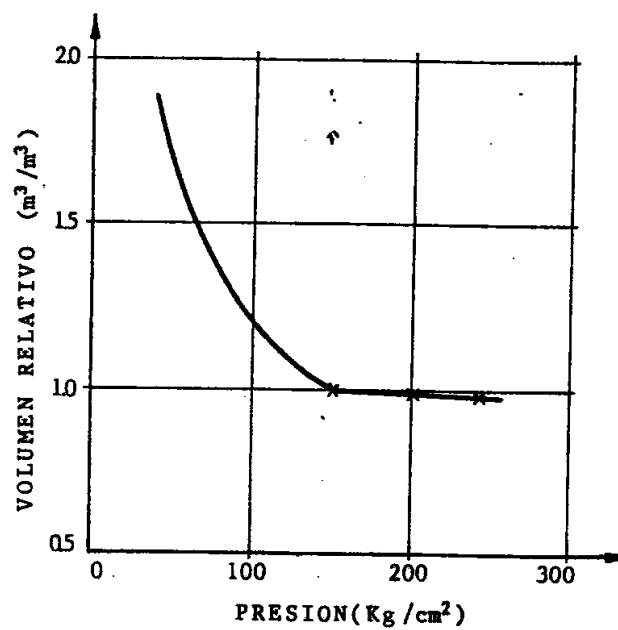
Fig. No 1.2 VARIACIÓN DEL VOLUMEN RELATIVO VERSUS LA PRESION
