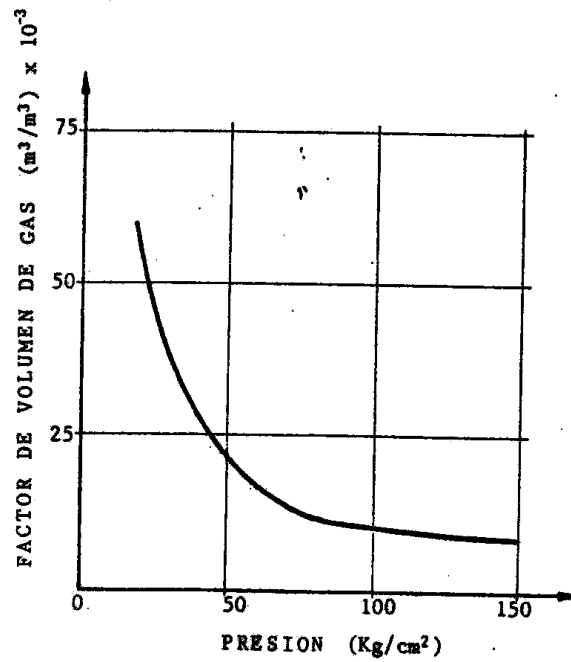
Fig. N° 1.4 VARIACIÓN DEL FACTOR DE VOLUMEN DEL GAS. VS. PRESION.
