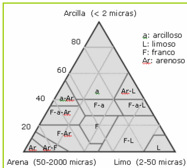
Figura 3-2: Esquema de la clasificación textural del suelo
