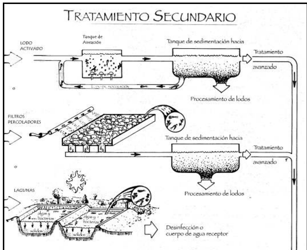
Figura 1.2 Tratamientos Secundarios (3) .
