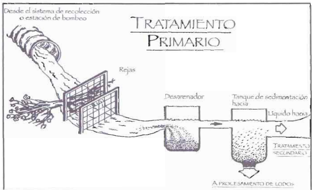
Figura 1.1 Tratamientos Primarios (2) .
