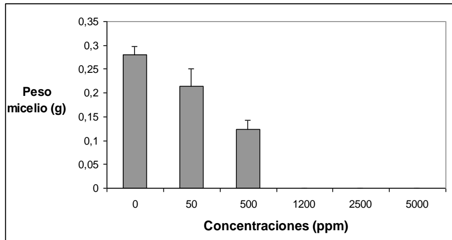
Figura 12. Peso del micelio (g) evaluado a los 15 días ante la presencia de diferentes dosis de Manganese en presentación orgánica
