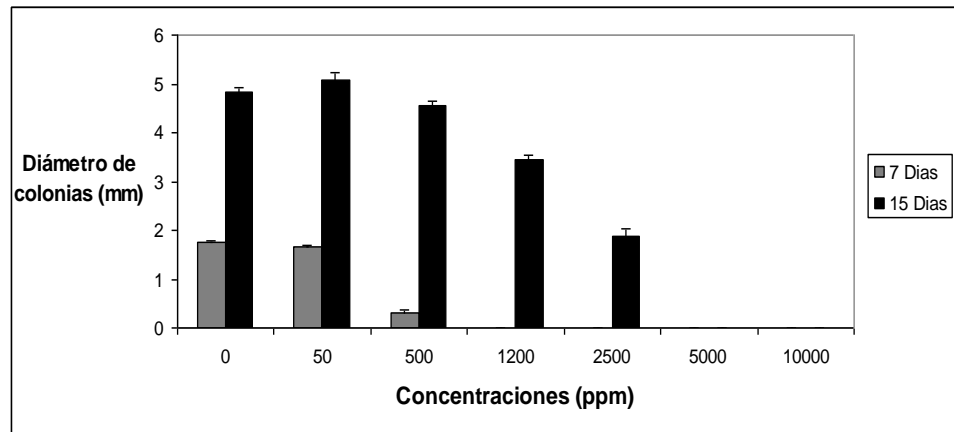
Figura 4. Diámetro de colonias (mm) en evaluaciones realizadas a los 7 y 15 días en presencia de diferentes dosis de Manganeso.
