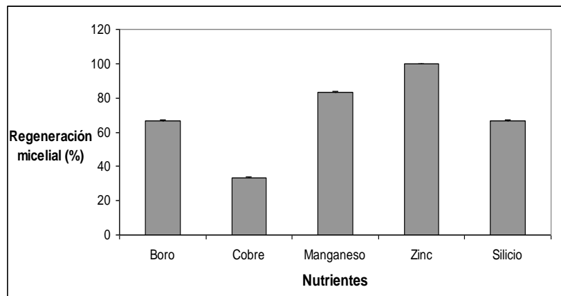
Figura 6. Porcentaje de regeneración de M. fijiensis , ante la aplicación de micro elementos en presentación inorgánica y Silicio.
