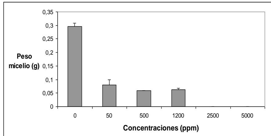
Figura 11. Peso del micelio (g) evaluado a los 15 días ante la presencia de diferentes dosis de Manganese
