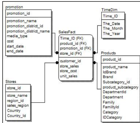
GRÁFICO 5.4. ESQUEMA DE ESTRELLA
