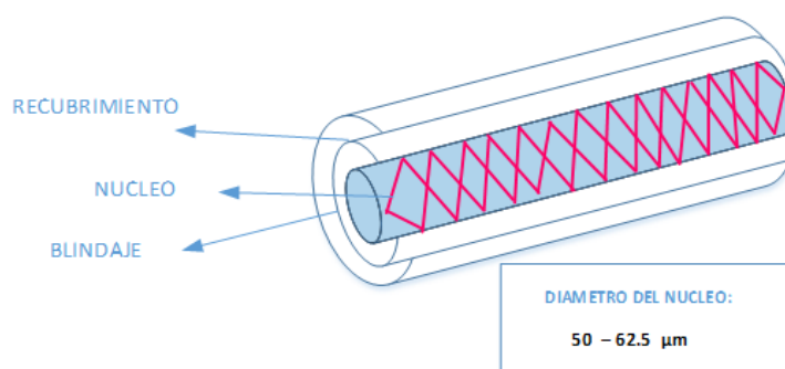
Figura 2.3: Fibra Multimodo
