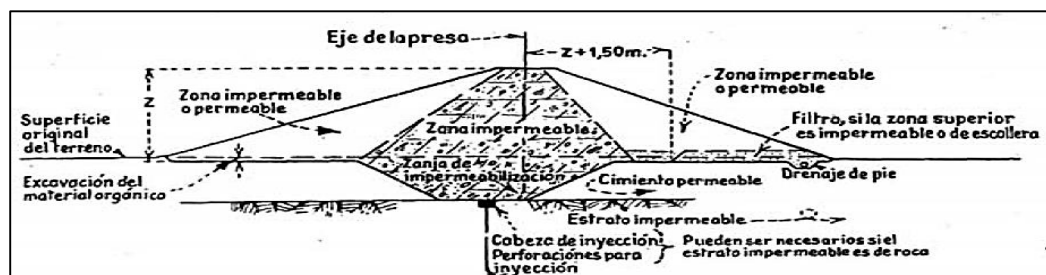
Figura 3.2. Presa Sonada.
