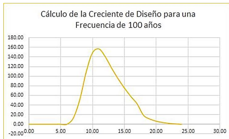
Figura 2.22. Curva Caudal vs Tiempo (SCS). Fuente: Autores, 2016.
