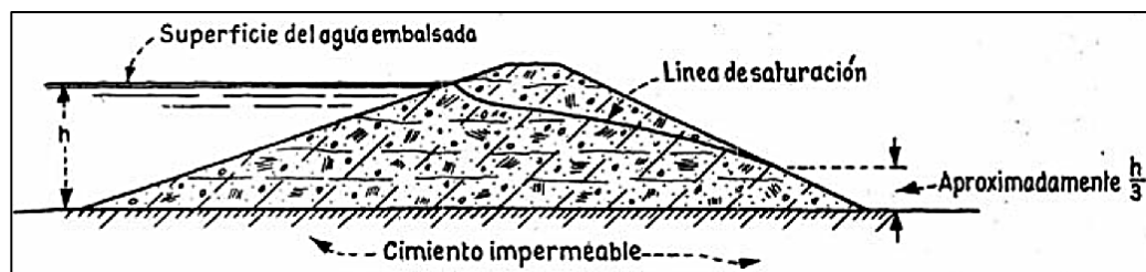
Figura 3.1. Presa homogénea.
