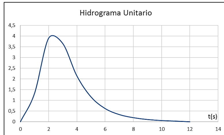
Figura 2.21. Hidrograma Unitario método SCS. Fuente: Autores, 2016.
