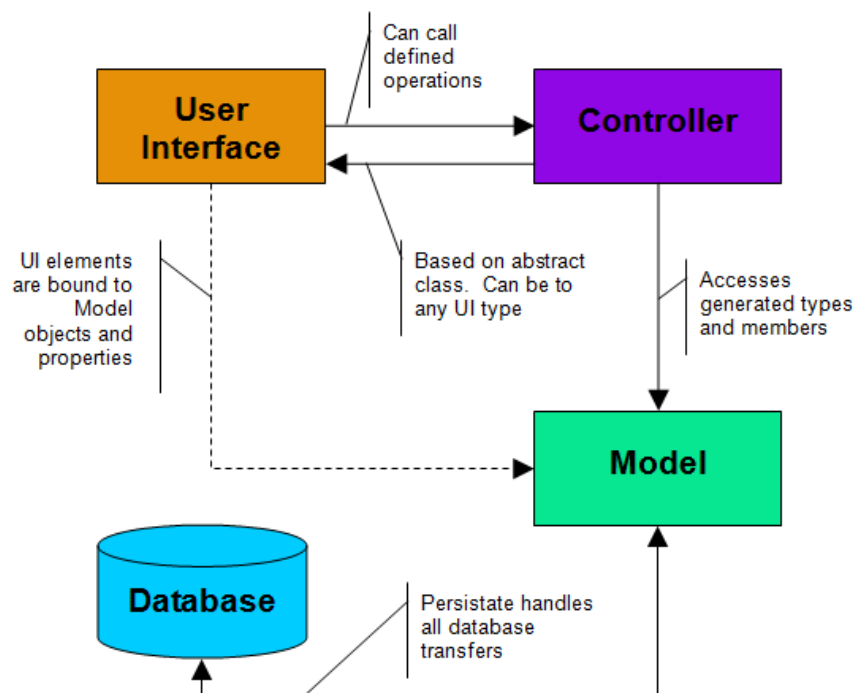
Figura 2.1: Diagrama Aplicación de Escritorio MVC
