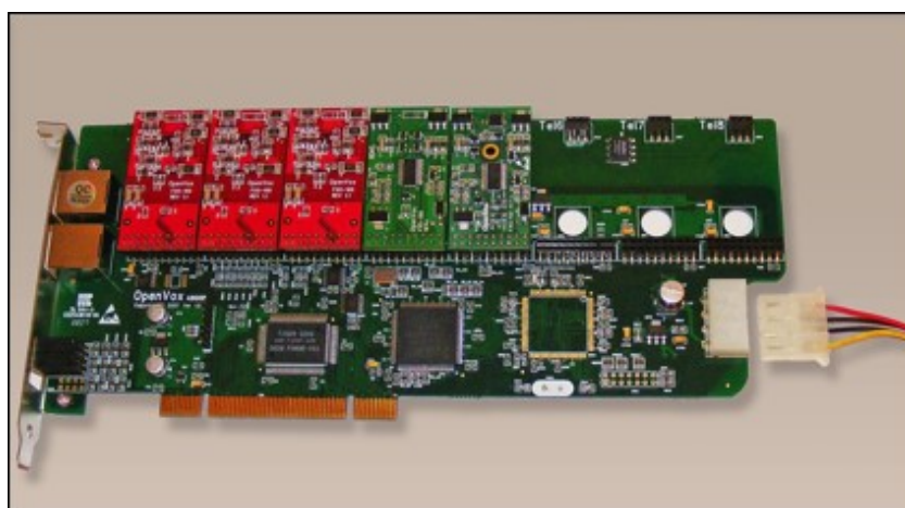
Figura 3.1: Tarjeta telefónica analógica de tipo modular con 3 módulos FXO y 2 FXS instalados
