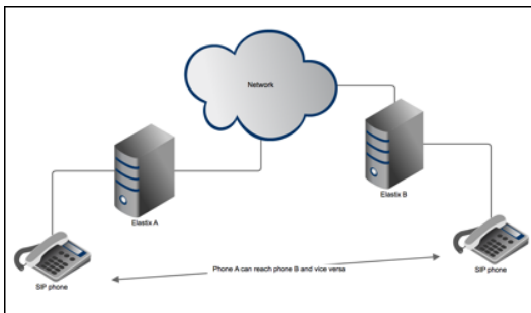
Figura 5.1: Interconectando dos Elastix
